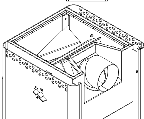
Fig. 8: Tourner le raccordement du conduit de fumée
