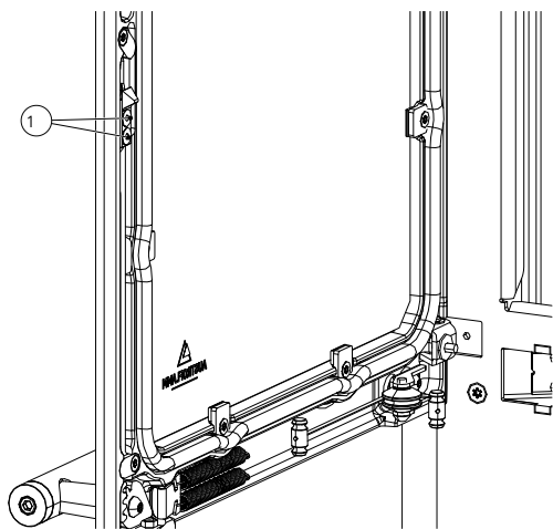
Fig. 11: Régler la distance de la porte par rapport au corps du poêle
