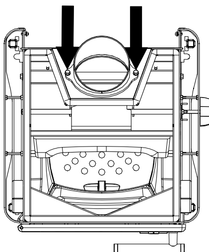
Fig. 7: Enlever la découpe perforée
