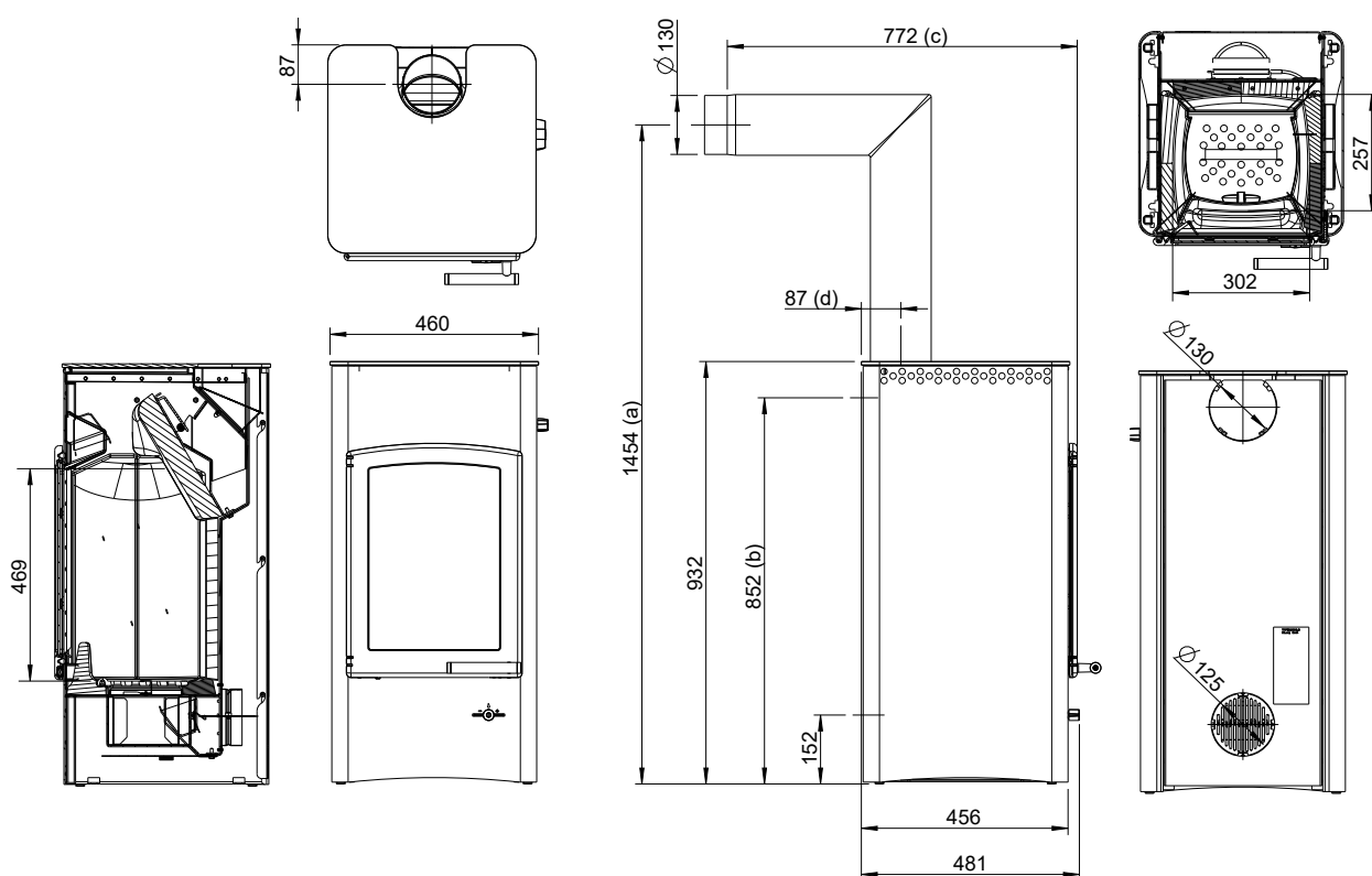
Fig. 1: Dimensions
