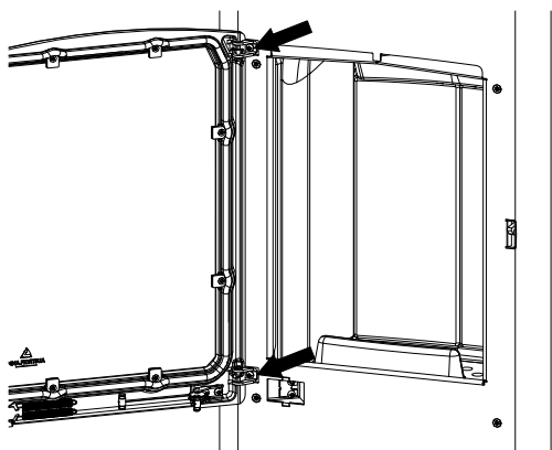
Fig. 12: Régler la porte
