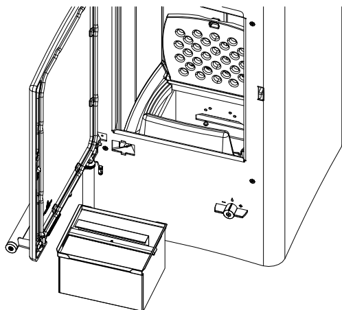
Fig. 22: Enlever et vider le bac à cendres
