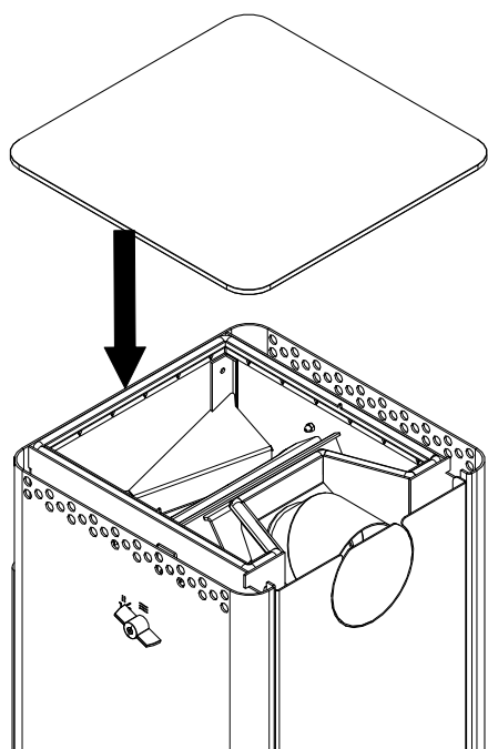
Fig. 9: Installer le panneau arrière et mettre le couvercle en place
