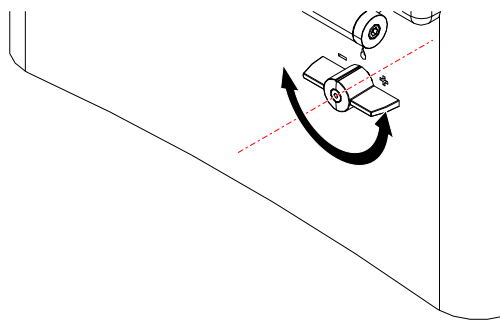
Fig. 13: Manette de régulation de l'air primaire / secondaire
