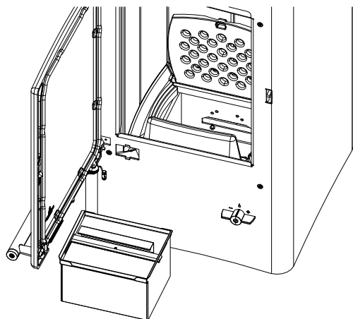
Fig. 24: Enlever et vider le bac à cendres
