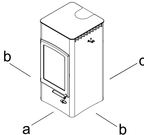
Fig. 7: Distances de sécurité
