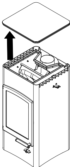
Fig. 25: Enlever la plaque de cuisson
