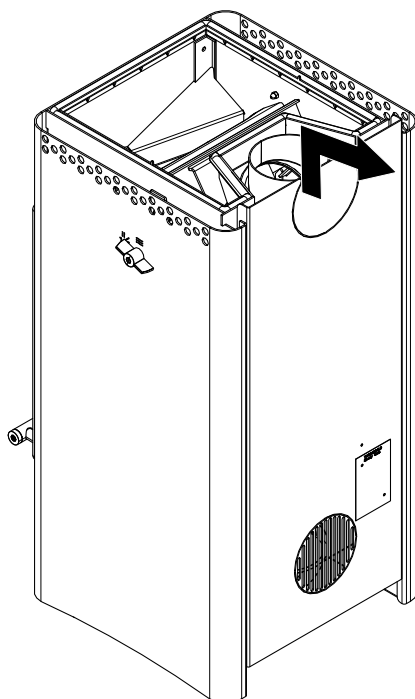
Fig. 26: Déposer la paroi arrière
