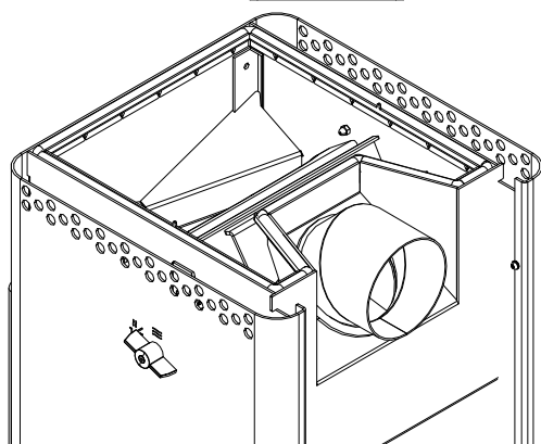
Fig. 8: Rotazione del tubo dei fumi
