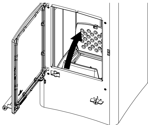
Fig. 19: Sollevamento della griglia
