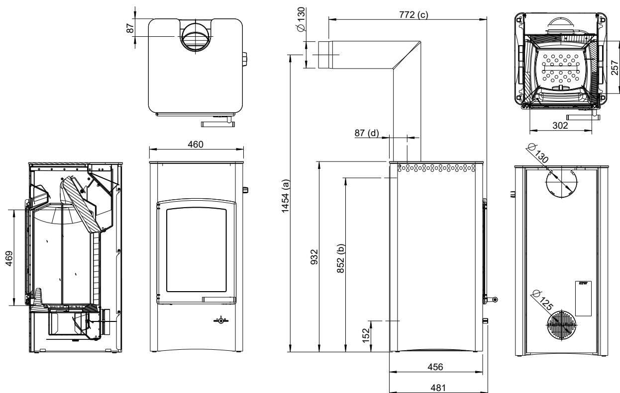
Fig. 1: Dimensioni
