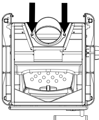
Fig. 7: Rimozione della parte perforata
