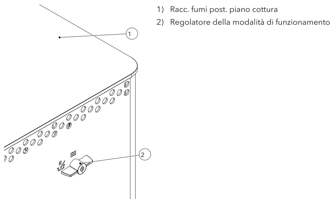
Fig. 16: Piastra di cottura e selettore della modalità di funzionamento
