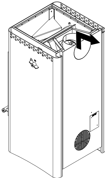
Fig. 24: Smontaggio della parete posteriore
