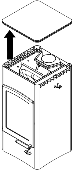
Fig. 23: Rimuovere la copertura.
