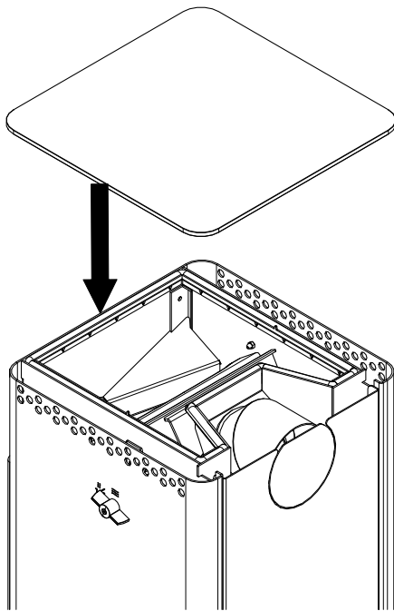
Fig. 9: Montaggio della parete posteriore e ricollocazione del coperchio
