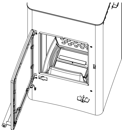
Fig. 23: Chiusura del coperchio
