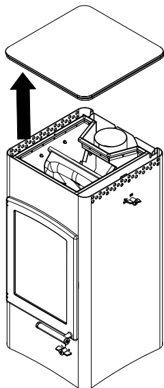
Fig. 25: Rimozione della piastra di cottura
