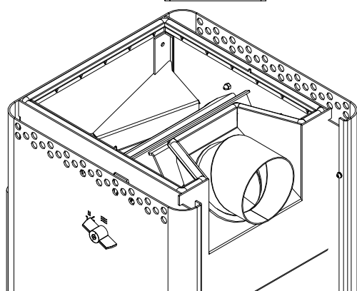
Fig. 9: Rotazione del tubo dei fumi
