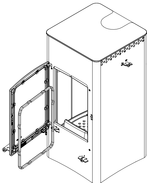
Fig. 20: Sostituzione della guarnizione
