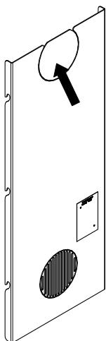
Fig. 8: Rimozione del taglio perforato
