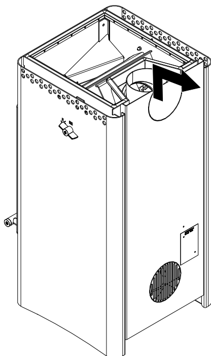
Fig. 26: Smontaggio della parete posteriore
