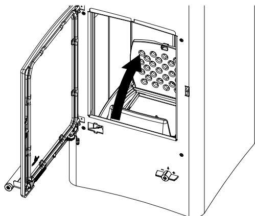
Fig. 21: Sollevamento della griglia
