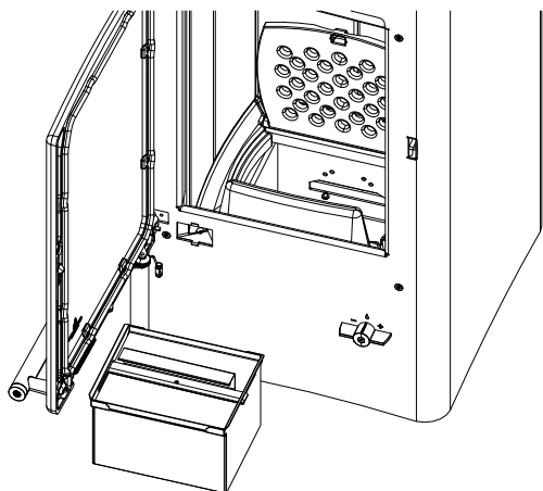
Fig. 24: Rimozione e svuotamento del box cenere
