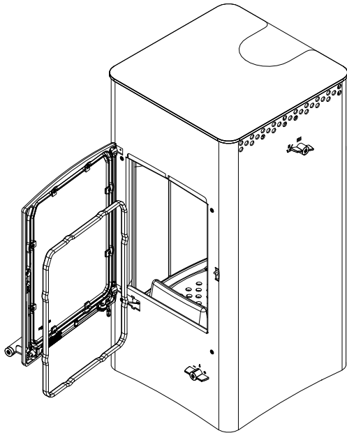
Abb. 21: Dichtung tauschen
