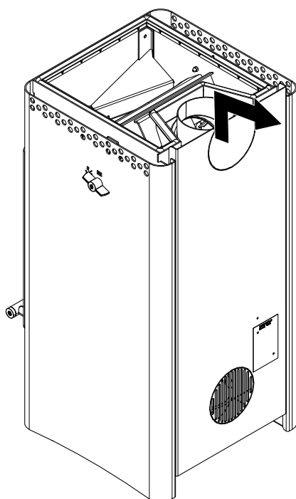
Abb. 27: Rückwand demontieren
