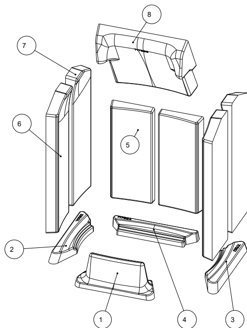
Abb. 12: Keramott
