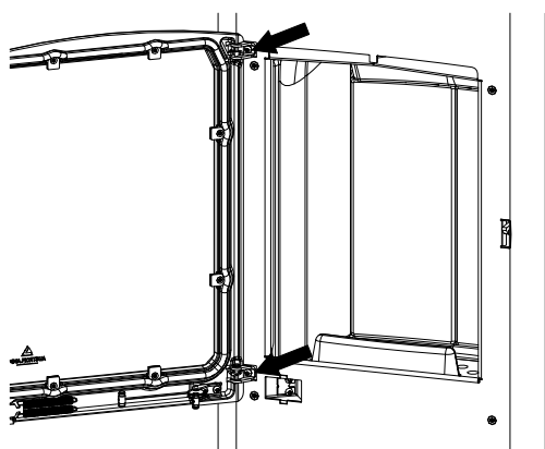
Abb. 14: Tür einstellen
