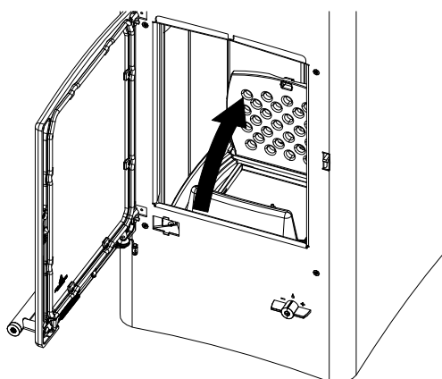
Abb. 22: Rost hochklappen
