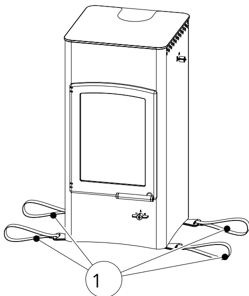
Abb. 7: Transportsicherungen entfernen
