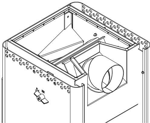
Abb. 10: Rauchrohranschluss drehen
