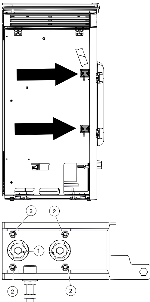
Fig. 16: Vis de réglage de la porte
