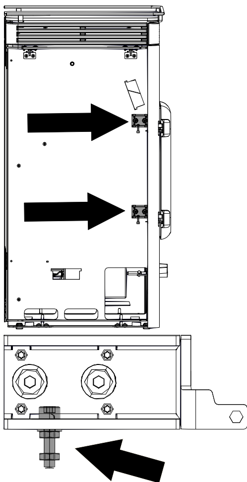
Fig. 18: Régler la force de fermeture de la porte
