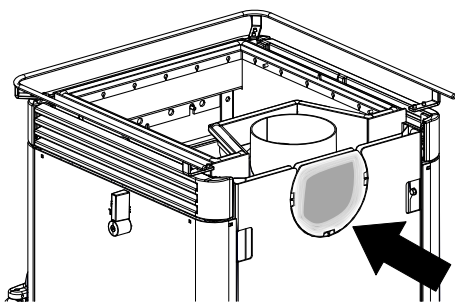
Fig. 8: Enlever la découpe perforée
