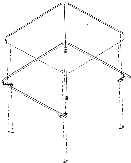
Fig. 14: Installer la main-courante (vue de dessous)
