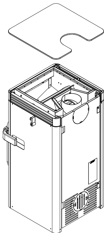
Fig. 13: Poser la plaque de cuisson
