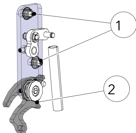
Fig. 17: Régler la serrure de la porte
