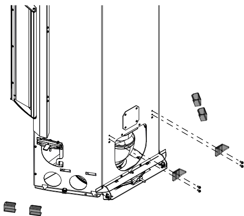
Fig. 31: Montaggio dei lamierini dell'HMS
