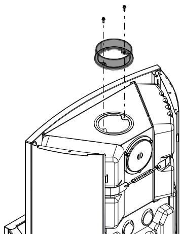
Fig. 24: Smontaggio della presa della canna fumaria
