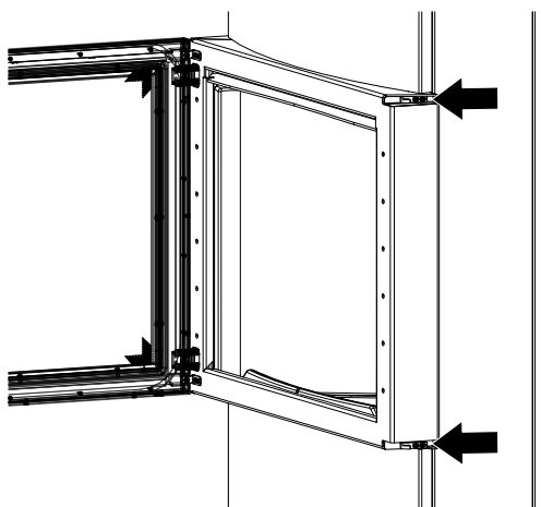
Fig. 50: Regolazione della serratura dello sportello
