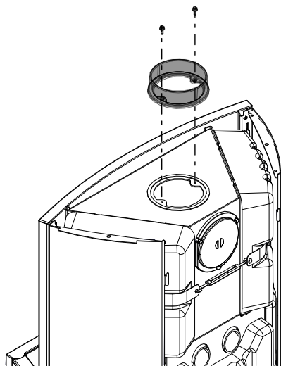
Fig. 17: Smontaggio della presa della canna fumaria
