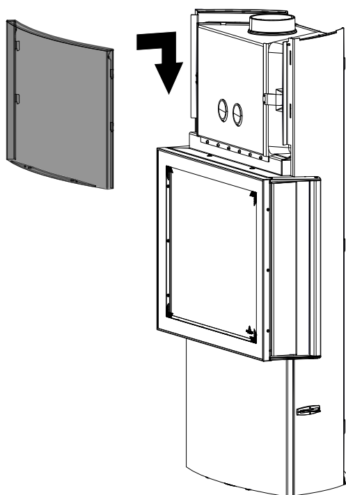
Fig. 39: Montaggio del diaframma superiore
