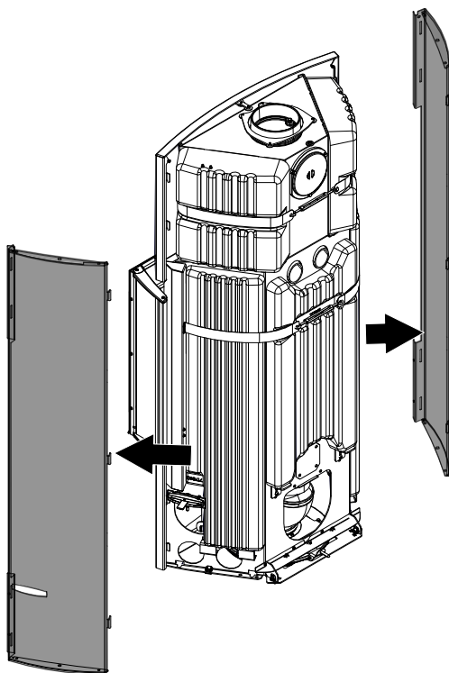
Fig. 68: Rimozione del rivestimento laterale
