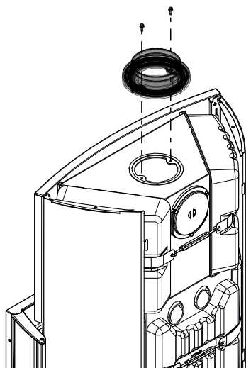
Fig. 18: Montaggio della presa della canna fumaria rotante
