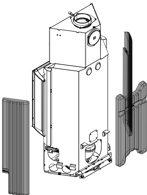
Fig. 32: Montaggio delle pietre HMS lateralmente
