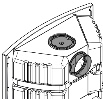
Fig. 11: Coperchio e pezzo di collegamento sostituiti
