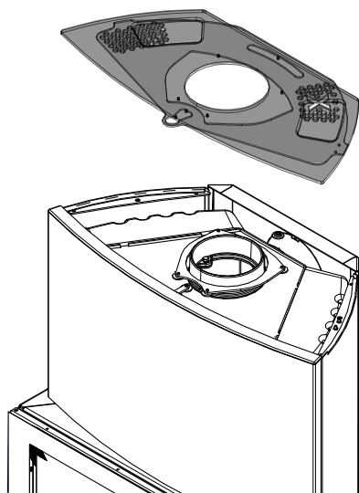
Fig. 45: Collocazione del coperchio
