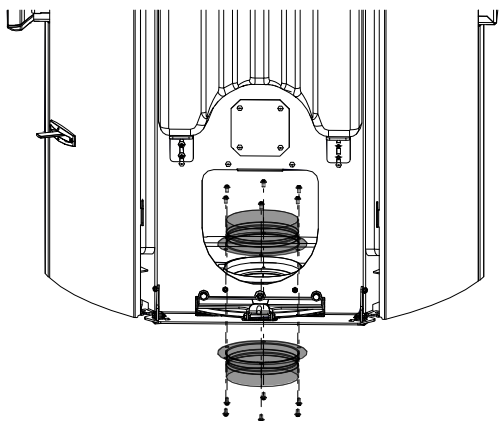
Fig. 28: Montaggio di entrambi i supporti
