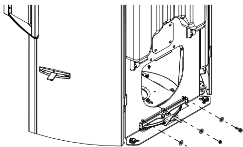
Fig. 20: Avvitamento del piatto girevole
