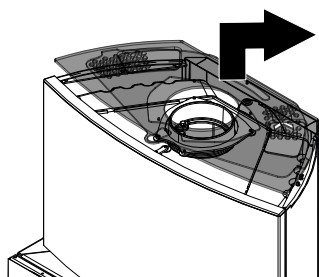
Fig. 22: Rimozione del coperchio
