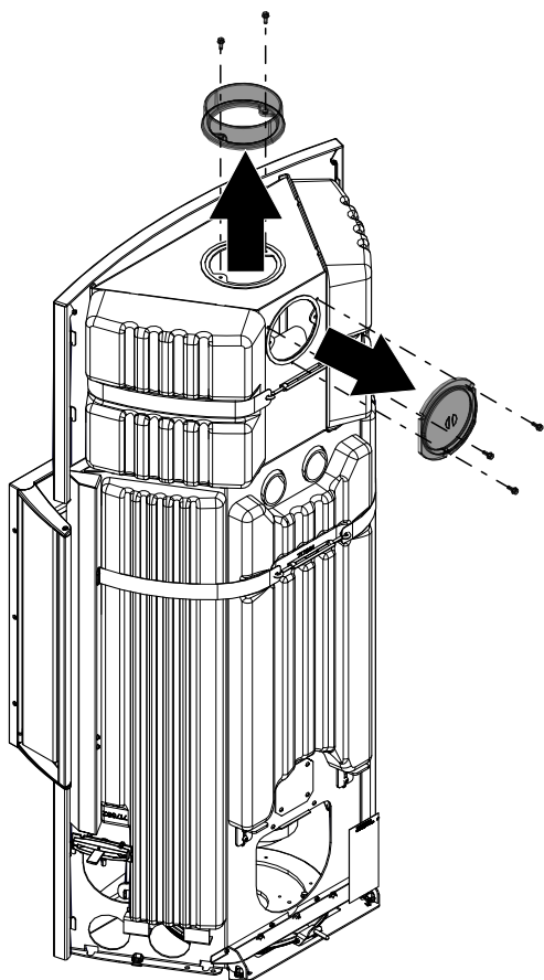
Fig. 9: Smontaggio del coperchio e della presa della canna fumaria
