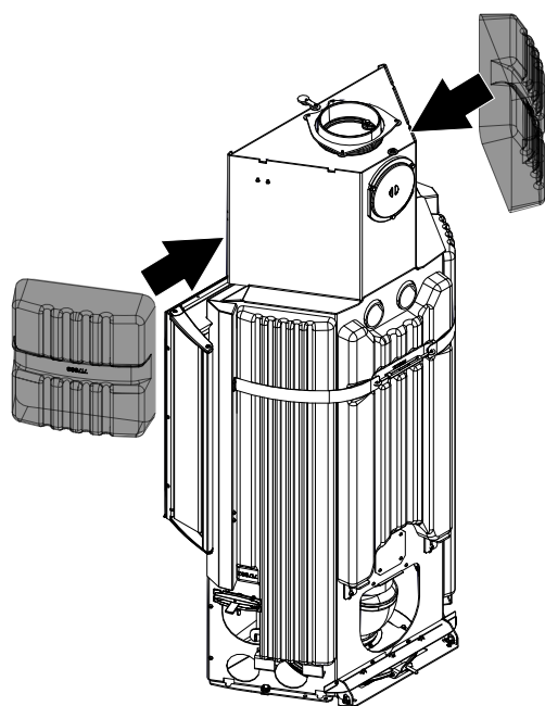
Fig. 34: Posizionamento delle pietre HMS in alto
