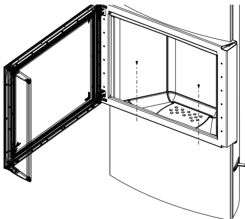
Fig. 42: Avvitamento del diaframma anteriormente
