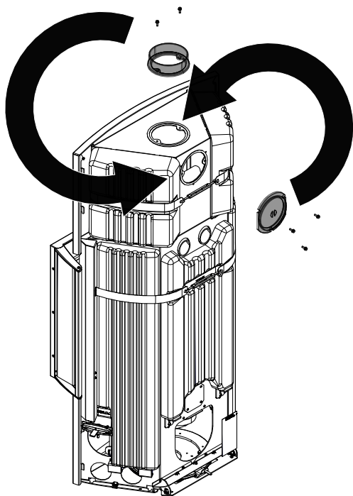
Fig. 10: Sostituzione del coperchio e del pezzo di collegamento
