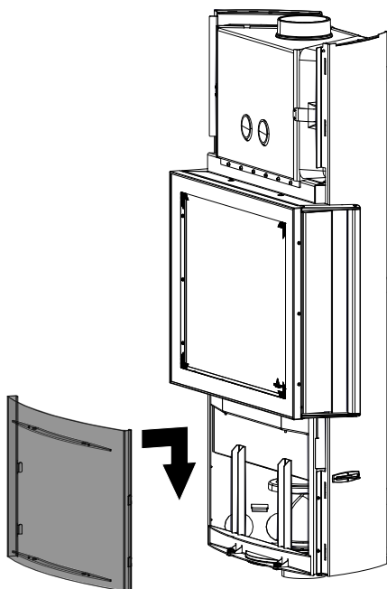
Fig. 38: Montaggio del diaframma inferiore
