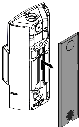
Fig. 59: Rimozione della parete posteriore
