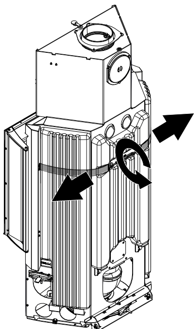
Fig. 71: Allentamento del tenditore
