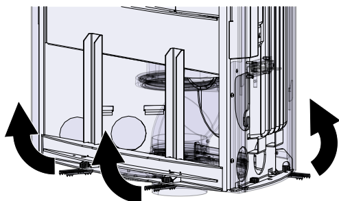
Fig. 6: Rimozione dei fermi di trasporto
