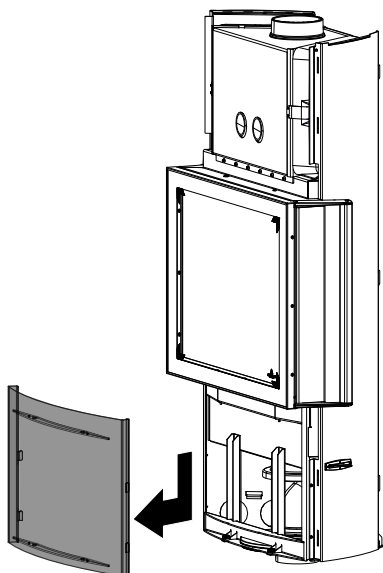
Fig. 66: Smontaggio del diaframma inferiore
