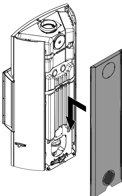
Fig. 44: Rimontaggio della parete posteriore e del coperchio
