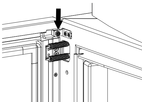
Fig. 47: Vite di regolazione dello sportello in alto
