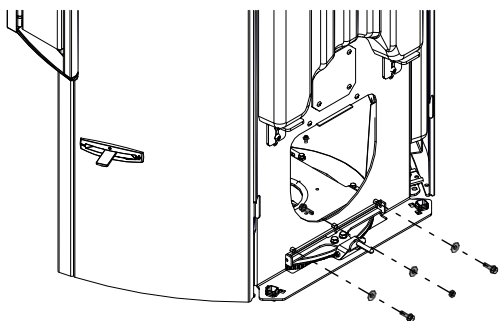
Fig. 27: Avvitamento del piatto girevole
