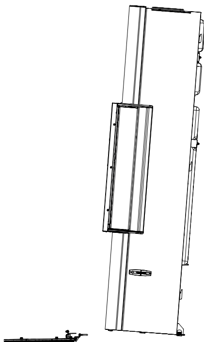
Fig. 18: Montaggio della presa della canna fumaria rotante
