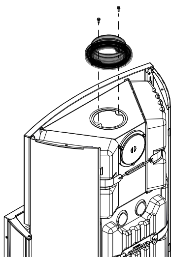
Fig. 25: Montaggio della presa della canna fumaria rotante
