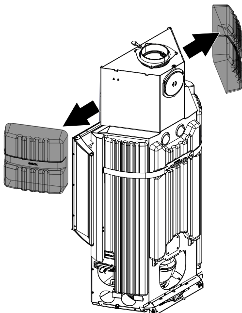
Fig. 70: Smontaggio delle pietre HMS lateralmente
