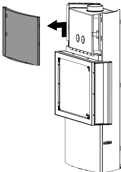
Fig. 64: Montaggio del diaframma superiore
