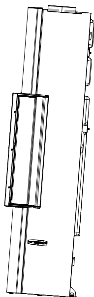
Fig. 65: Inclinare la stufa indietro
