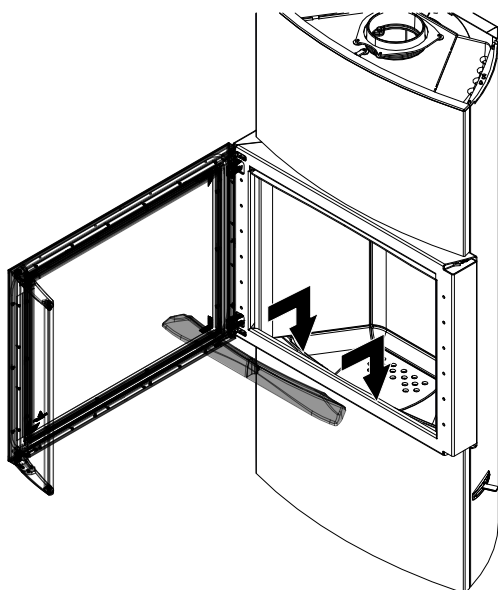
Fig. 43: Montaggio del fermalegna
