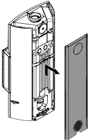
Fig. 16: Rimozione della parete posteriore
