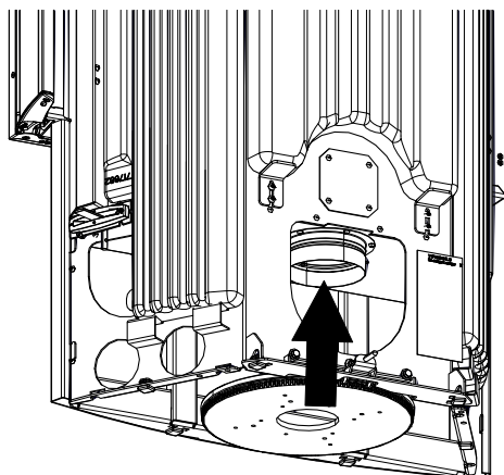
Fig. 14: Fissaggio del tubo Aluflex
