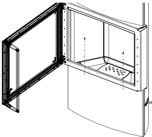
Fig. 62: Allentamento del collegamento a vite anteriore del diaframma
