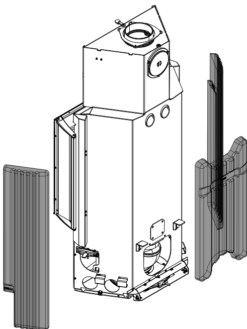
Fig. 72: Smontaggio delle pietre HMS
