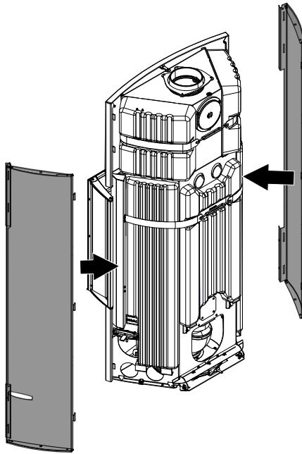
Fig. 36: Montaggio del rivestimento laterale
