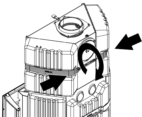
Fig. 35: Fissaggio delle pietre HMS in alto
