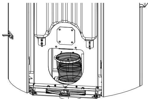
Fig. 29: Fissaggio del tubo
