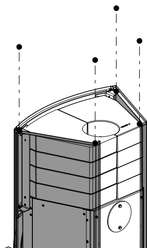
Fig. 34: Enlever l'habillage latéral
