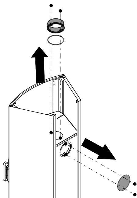
Fig. 9: Démonter le recouvrement et la tubulure de fumées
