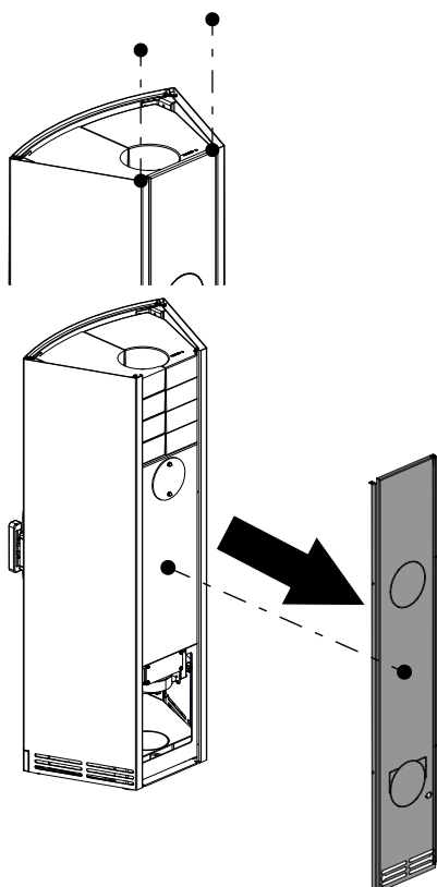
Fig. 33: Dévisser les vis de la paroi arrière
