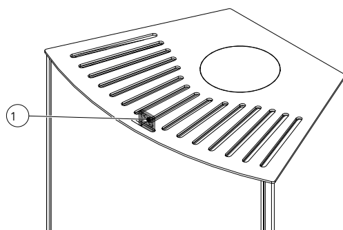
Abb. 32: Konvektionsluftregler
