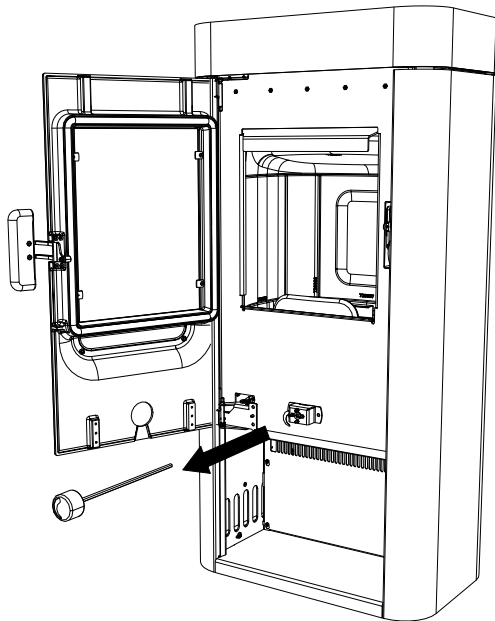
Abb. 15: Drehreglereinheit ausbauen
