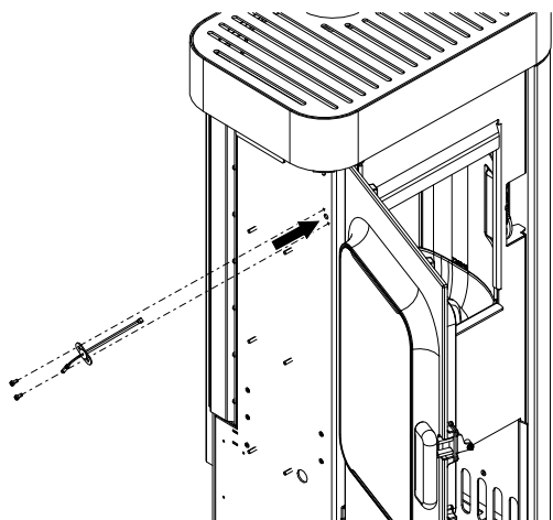
Abb. 18: Feuerraumtemperaturfühler befestigen
