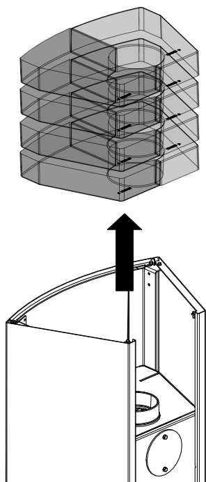
Abb. 9: Xtra-Steine rausnehmen
