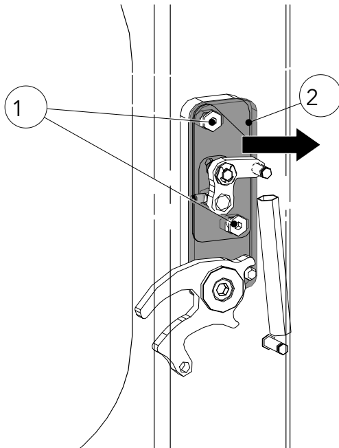
Abb. 23: Türverschluss einstellen
