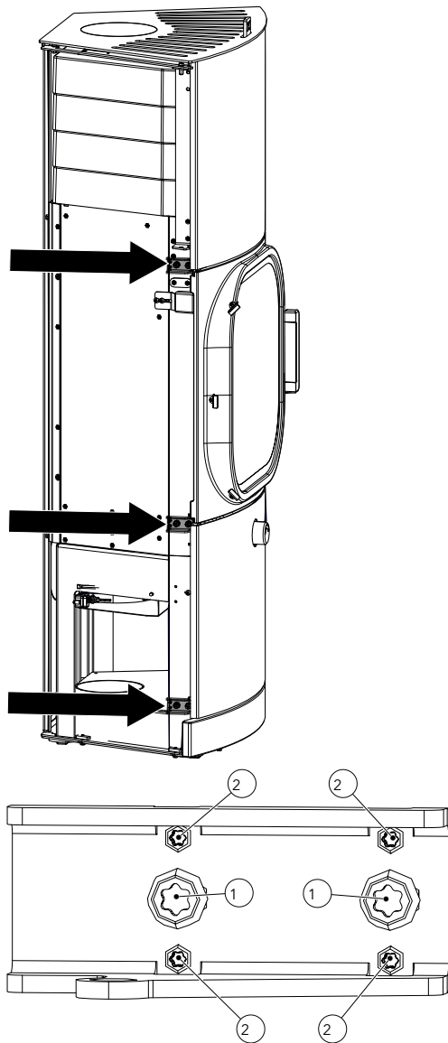
Abb. 21: Türeinstellschrauben
