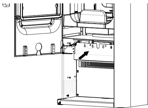
Abb. 20: Abdeckung montieren
