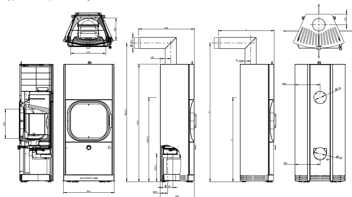
Abb. 2: Abmessungen Grundgerät
