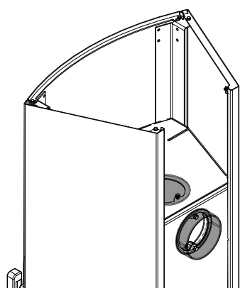
Fig. 11: Recouvrement et tubulure échangés
