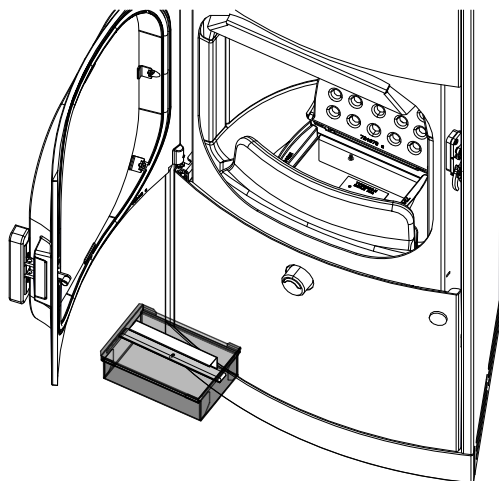
Fig. 30: Enlever et vider le bac à cendres
