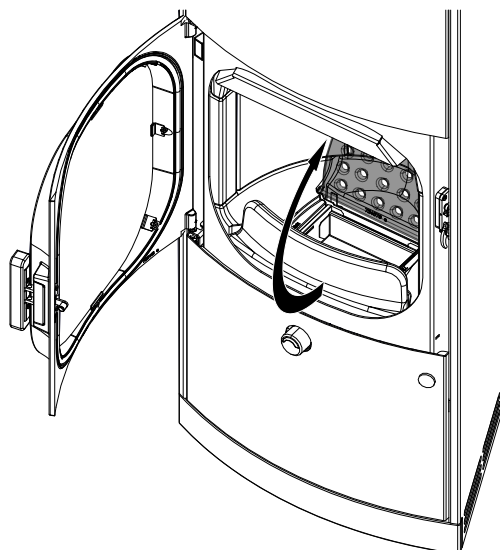
Fig. 27: Relever la grille
