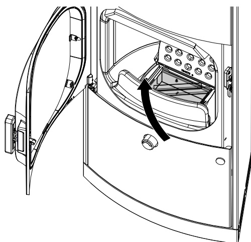
Fig. 28: Mettre le couvercle sur le bac à cendres
