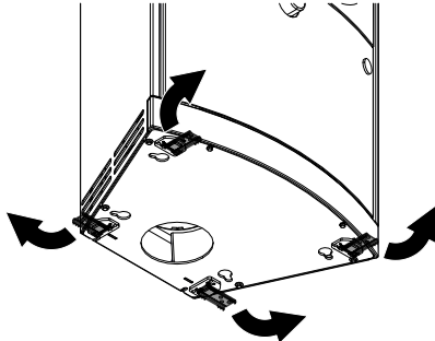
Abb. 6: Transportsicherung entfernen
