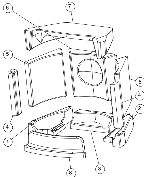
Abb. 14: Keramott montieren
