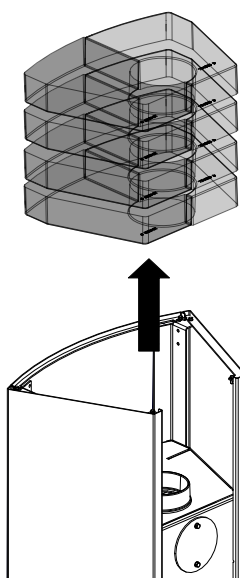
Abb. 9: Xtra-Steine herausnehmen
