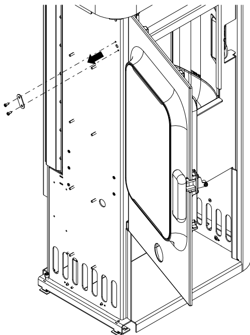
Abb. 16: Abdeckplatte entfernen
