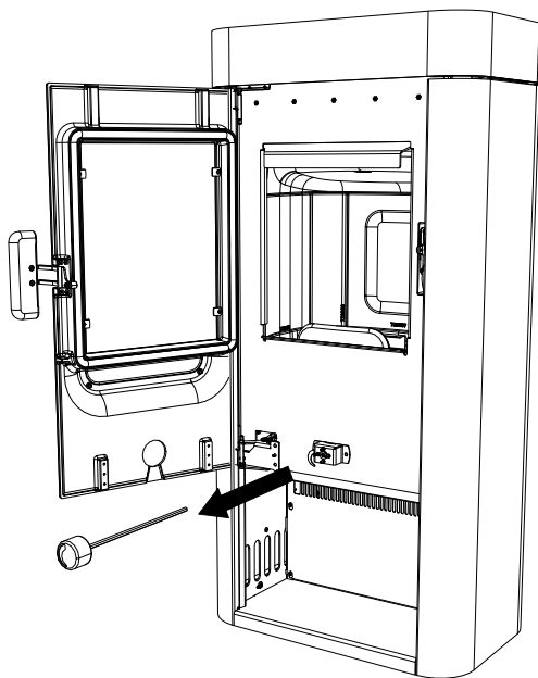
Abb. 15: Drehreglereinheit ausbauen
