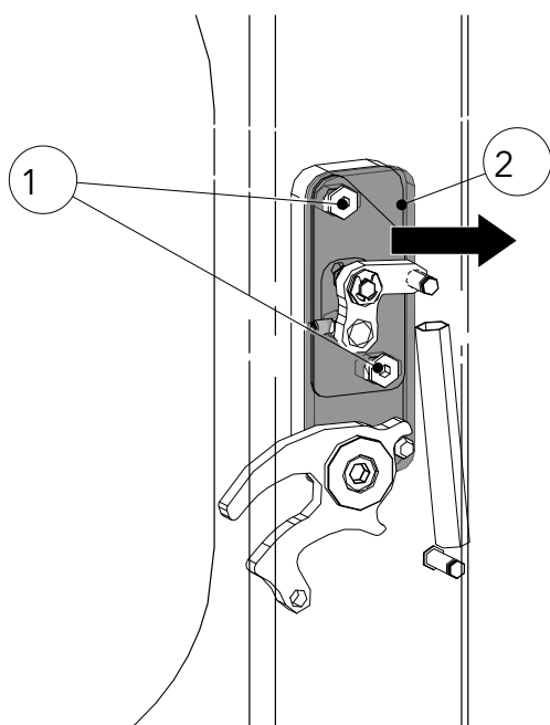
Abb. 23: Türverschluss einstellen
