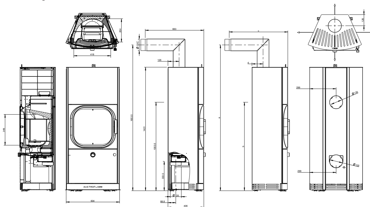
Abb. 2: Abmessungen Grundgerät
