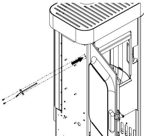
Abb. 18: Feuerraumtemperaturfühler befestigen
