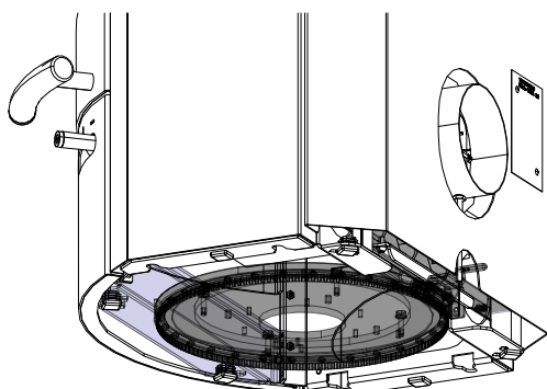
Fig. 23: Posizionamento del piatto girevole
