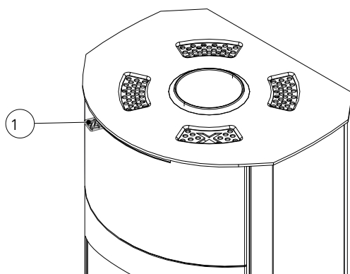
Fig. 34: Serranda di regolazione dell'aria di convezione APERTO-CHIUSO
