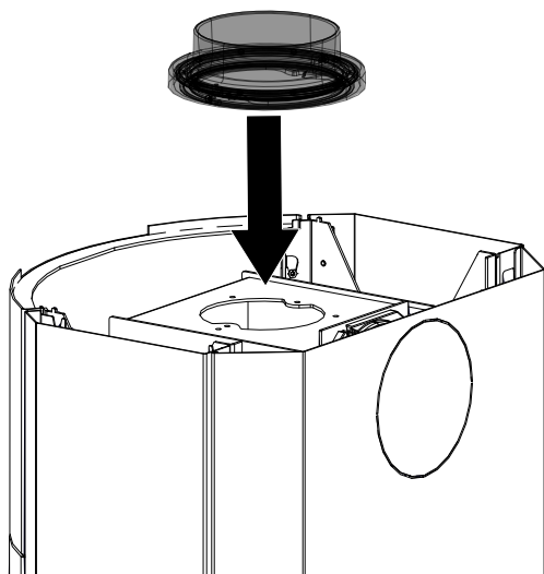
Fig. 20: Montaggio della presa della canna fumaria rotante
