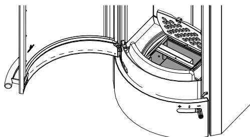
Fig. 32: Chiusura del coperchio
