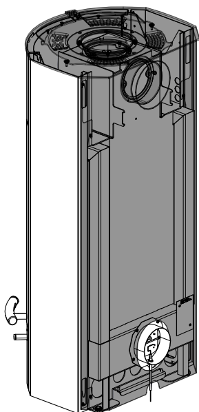
Fig. 15: Montaggio della parte posteriore
