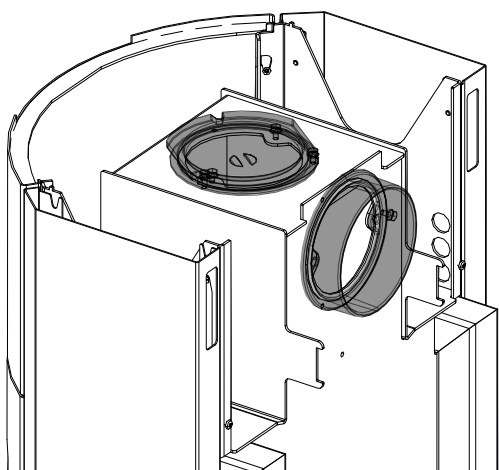
Fig. 14: Copertura e pezzo di collegamento sostituiti
