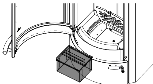
Fig. 33: Rimozione e svuotamento del box cenere
