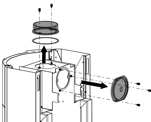
Fig. 12: Smontaggio del coperchio e della presa della canna fumaria
