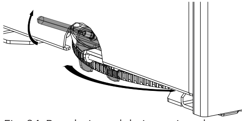
Fig. 24: Regolazione del piatto girevole
