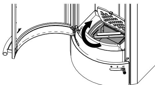
Fig. 31: Coperchio sul box cenere
