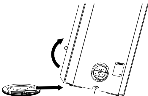
Fig. 22: Inclinamento della stufa
