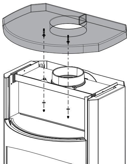
Fig. 55: Installer le couvercle
