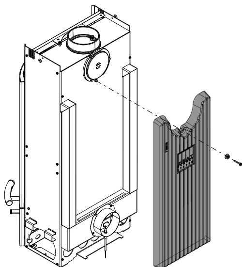
Fig. 30: Installer la pierre HMS au dos
