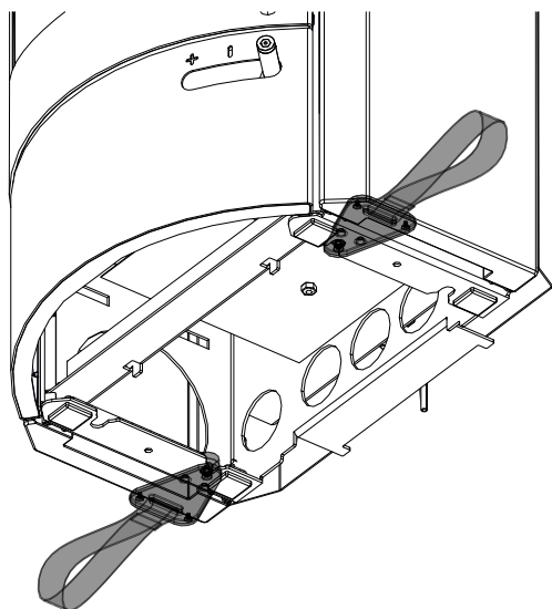
Fig. 6: Aide au transport
