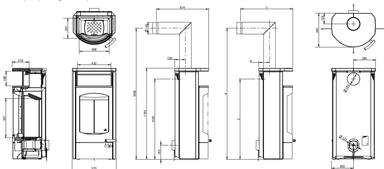
Fig. 1: Dimensions
