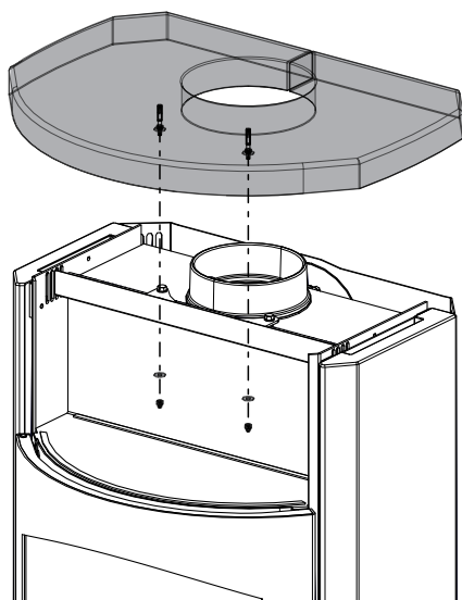
Fig. 34: Installer le couvercle
