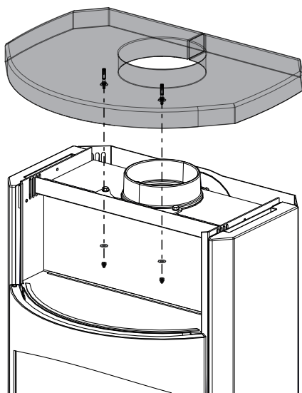
Fig. 17: Enlever le couvercle
