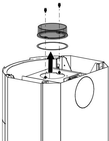
Fig. 19: Démonter la tubulure de fumées
