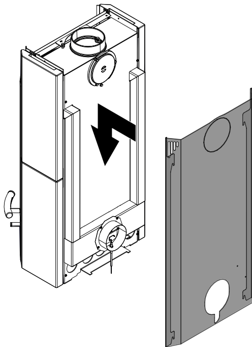
Fig. 54: Installer le panneau arrière
