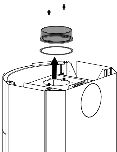
Fig. 19: Démonter la tubulure de fumées
