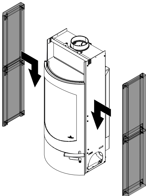
Fig. 25: Installer l'habillage latéral
