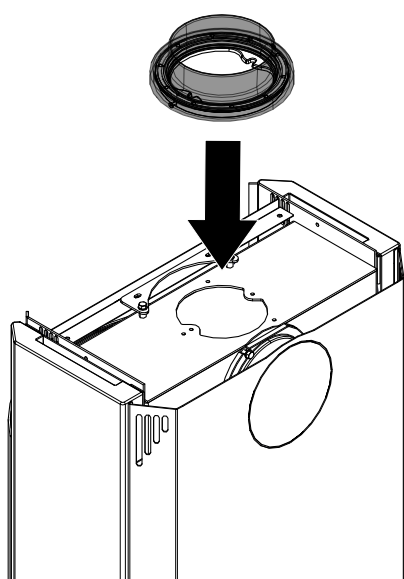
Fig. 20: Installer la tubulure de fumées orientable
