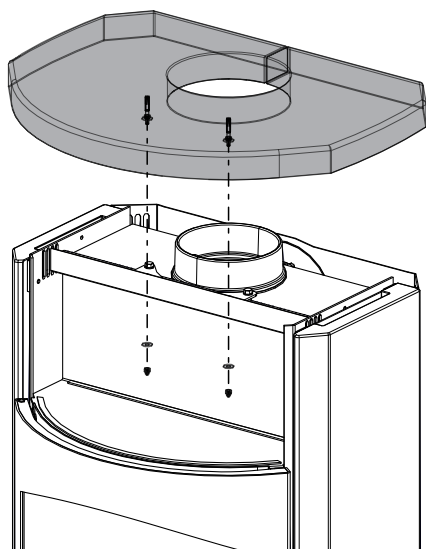
Fig. 17: Enlever le couvercle
