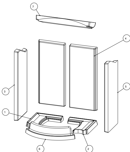
Fig. 15: Installer la Keramott
