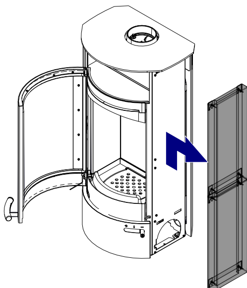
Fig. 38: Déposer l'habillage latéral
