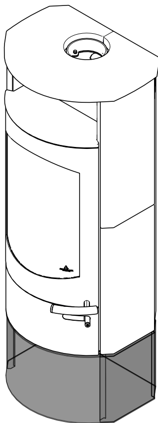
Fig. 16: Installer le socle
