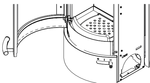
Fig. 39: Régler la serrure de la porte
