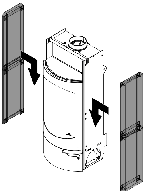
Fig. 53: Installer l'habillage latéral
