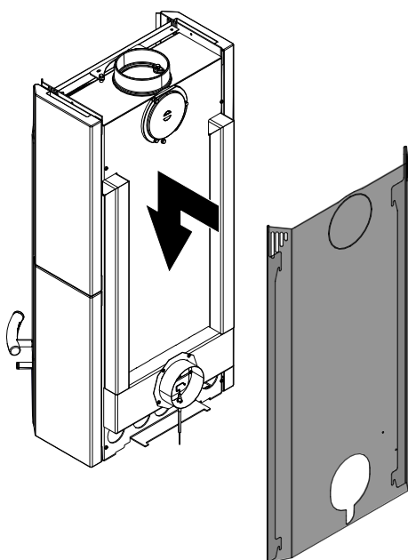
Fig. 33: Installer le panneau arrière
