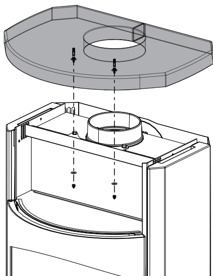
Fig. 14: Installer le couvercle
