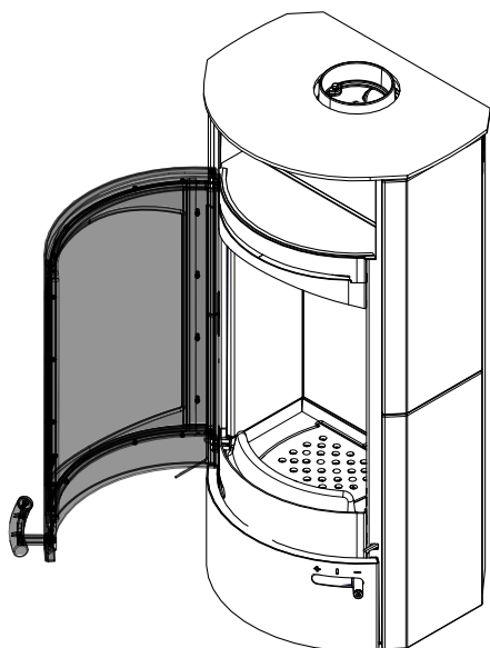
Fig. 40: Ouvrir la porte
