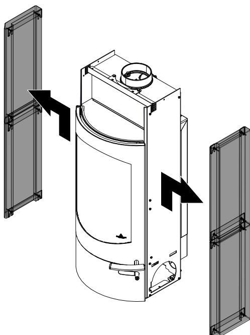
Fig. 50: Enlever l'habillage latéral
