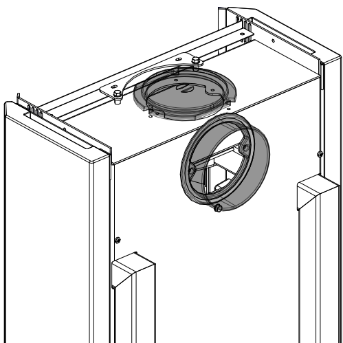
Fig. 12: Recouvrement et tubulure échangés
