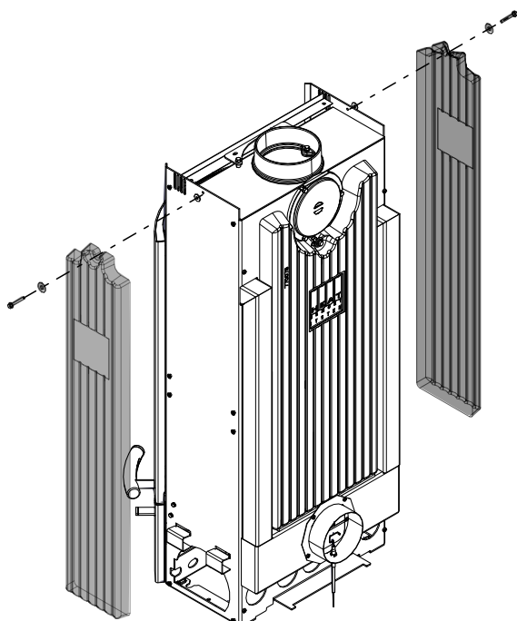
Fig. 31: Installer les pierres HMS sur le côté
