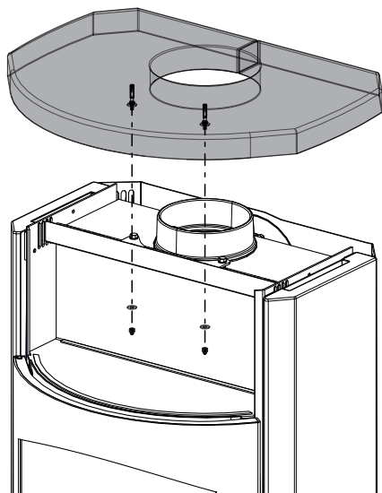
Fig. 7: Enlever le couvercle
