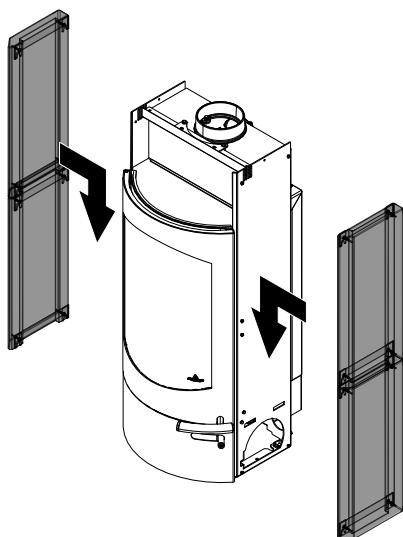
Fig. 32: Poser le capot latéral
