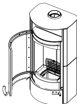
Fig. 45: Relever la grille
