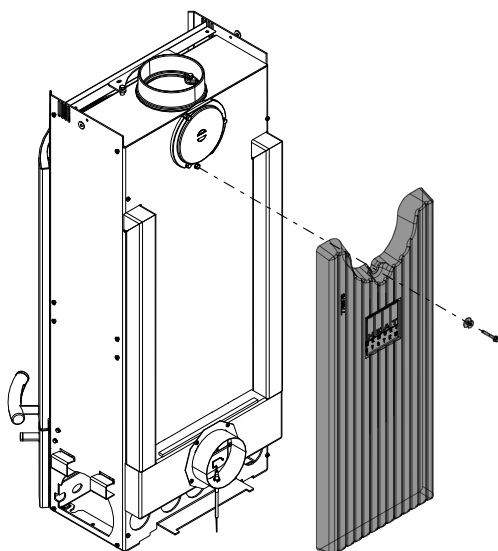
Fig. 30: Installer la pierre HMS au dos
