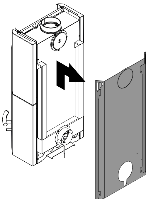
Fig. 8: Enlever la plaque arrière
