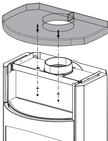
Fig. 55: Installer le couvercle
