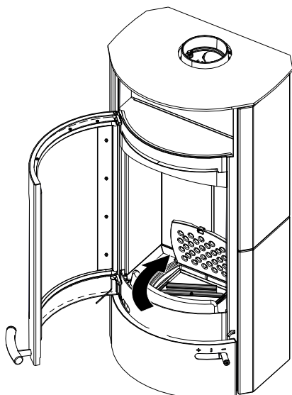
Fig. 46: Mettre le couvercle sur le bac à cendres
