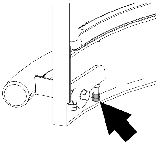
Fig. 41: Régler la force de fermeture de la porte
