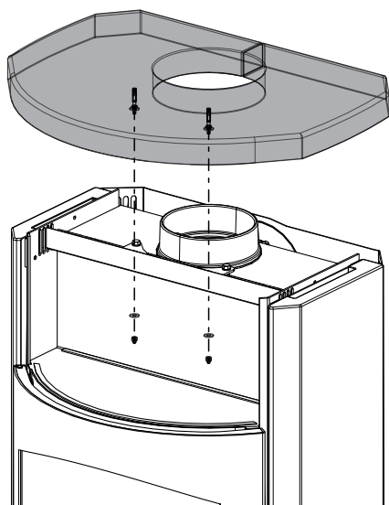
Fig. 34: Installer le couvercle
