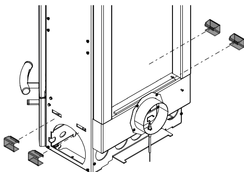
Fig. 29: Installer les tôles HMS
