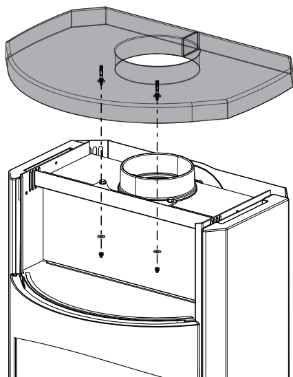
Fig. 49: Enlever le couvercle
