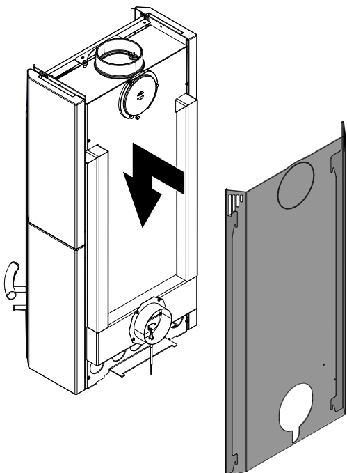
Fig. 13: Installer le panneau arrière
