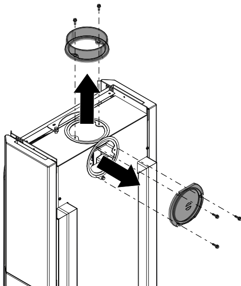
Fig. 10: Démonter le recouvrement et la tubulure de fumées
