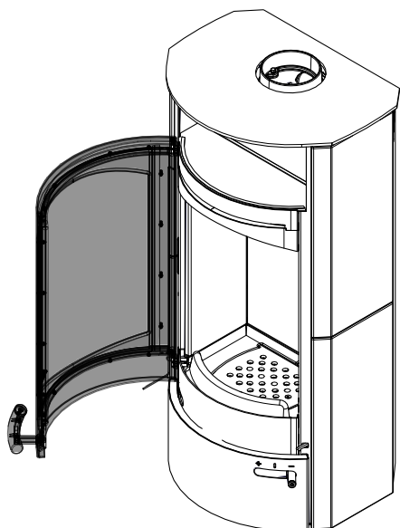
Fig. 37: Ouvrir la porte
