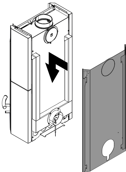
Fig. 26: Installer le panneau arrière
