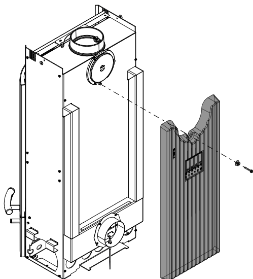
Fig. 52: Dévisser les vis et déposer l'HMS
