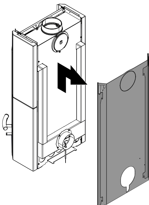
Fig. 18: Enlever le panneau arrière
