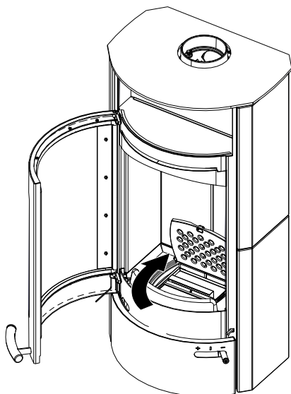
Fig. 47: Fermer le couvercle
