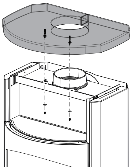
Fig. 17: Rimozione del coperchio
