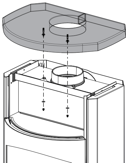
Fig. 7: Rimozione del coperchio
