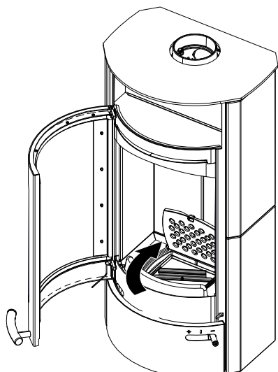
Fig. 46: Coperchio sul box cenere
