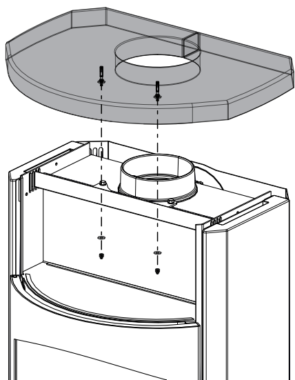
Fig. 14: Montaggio del coperchio
