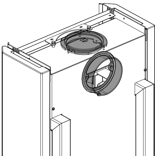
Abb. 13: Abdeckung und Stutzen vertauscht
