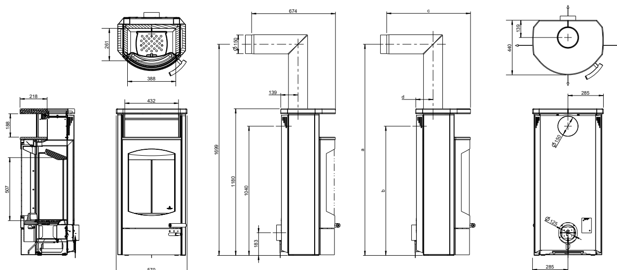
Abb. 2: Abmessungen
