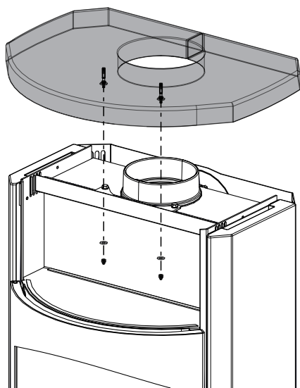
Abb. 56: Deckel montieren
