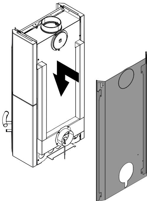
Abb. 55: Rückwand montieren
