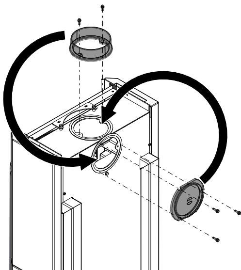
Abb. 12: Abdeckung und Stutzen tauschen
