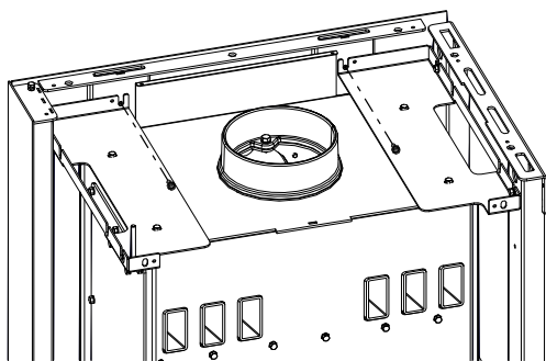
Fig. 37: Déposer le panneau arrière
