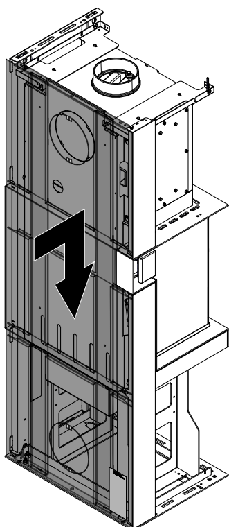
Fig. 9: Installer le panneau arrière
