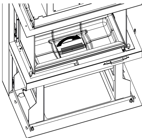
Fig. 34: Mettre le couvercle sur le bac à cendres et fermer le couvercle
