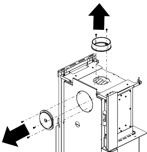
Fig. 12: Démonter le recouvrement et la tubulure de fumées
