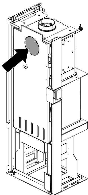
Fig. 11: Enlever la découpe perforée
