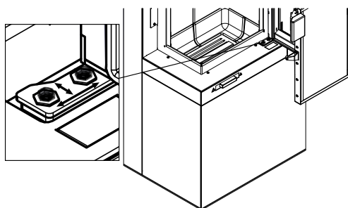
Fig. 24: Régler la charnière.
