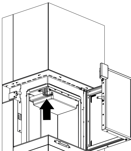
Fig. 32: Extraire la Keramott
