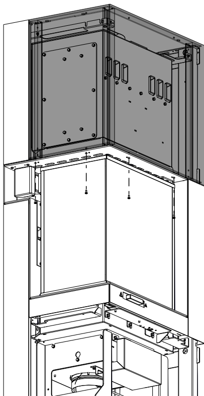
Fig. 44: Dévisser les vis du revêtement supérieur.
