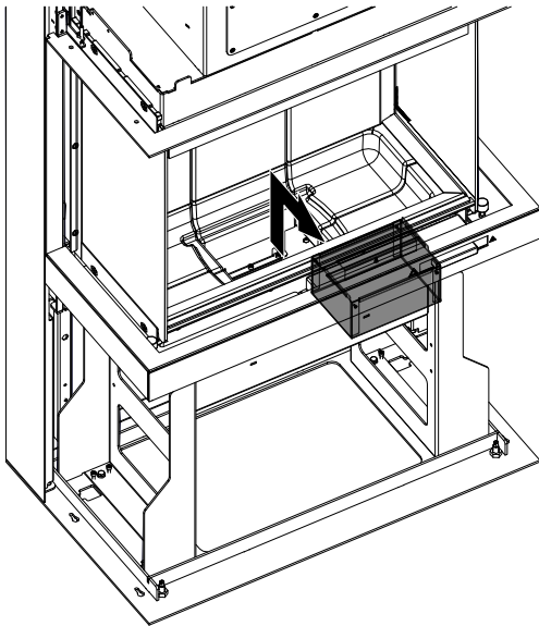
Fig. 35: Enlever et vider le bac à cendres
