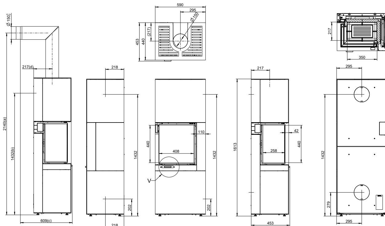
Fig. 1: Dimensions KAMIBA 59 K2 gauche
