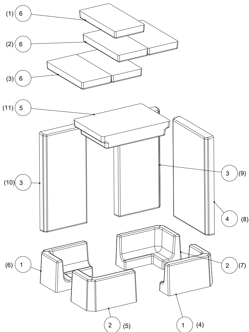
Fig. 20: Installer la Keramott
