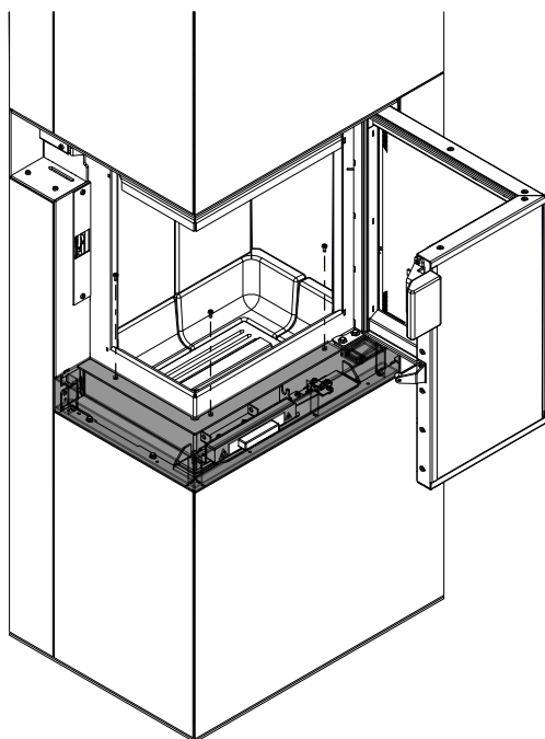
Fig. 41: Déposer le parement
