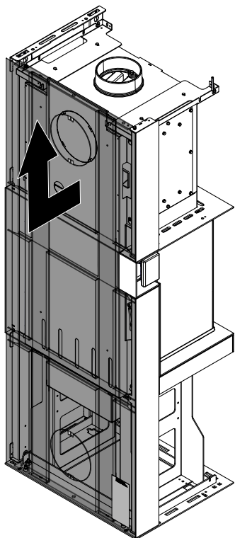
Fig. 17: Enlever la paroi arrière
