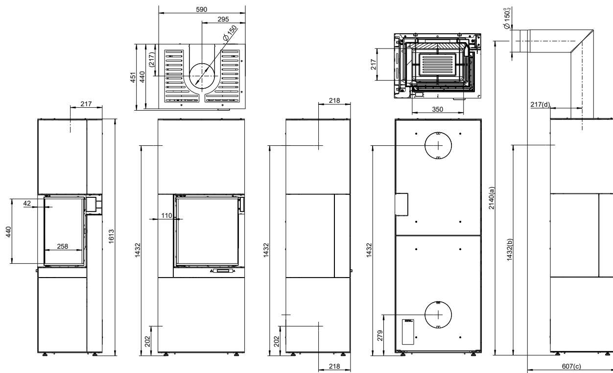
Fig. 2: Dimensions KAMIBA 59 K2 droite
