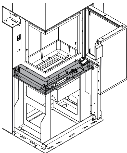
Fig. 43: Retirez le parement inférieur
