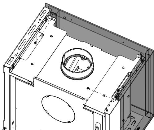
Fig. 45: Smontaggio del rivestimento superiore dall'alto.
