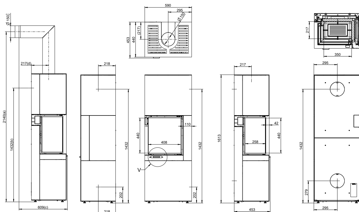
Fig. 1: Dimensioni Kamiba 59 K2 sinistra
