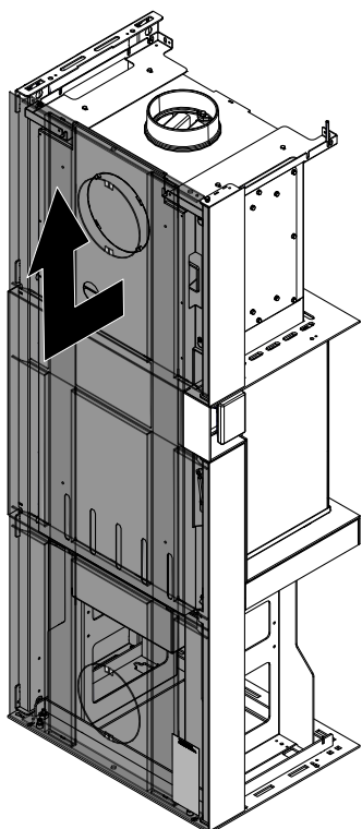
Fig. 17: Rimozione della parete posteriore
