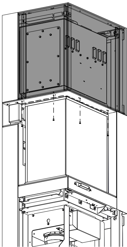
Fig. 44: Svitare le viti del rivestimento superiore.
