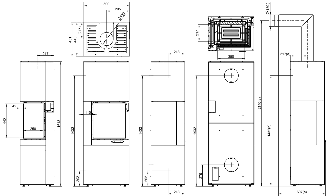
Fig. 2: Dimensioni Kamiba 59 K2 destra
