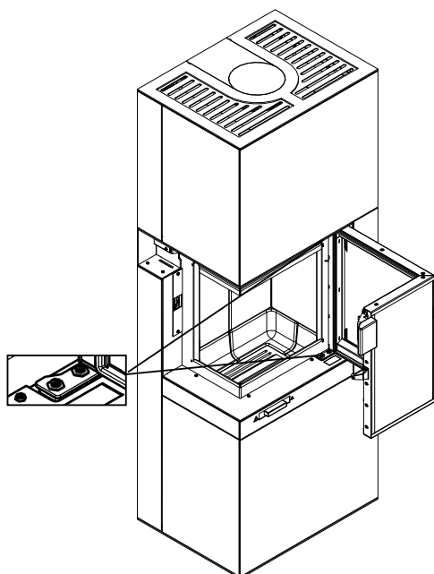
Fig. 23: Svitamento delle viti
