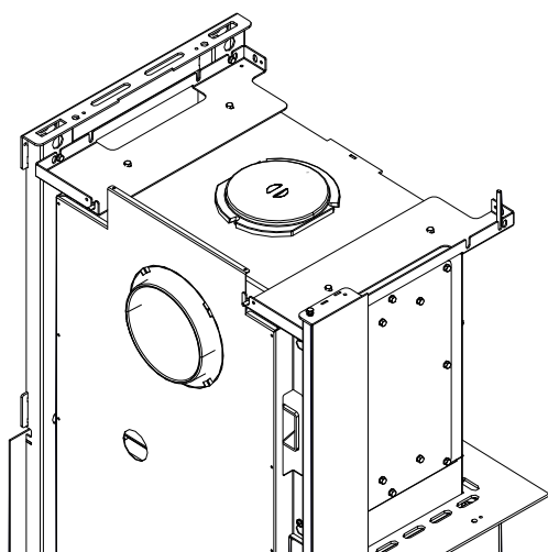
Fig. 14: Coperchio e la presa della canna fumaria scambiati
