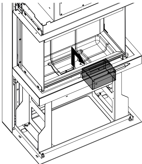
Fig. 35: Rimozione e svuotamento del box cenere
