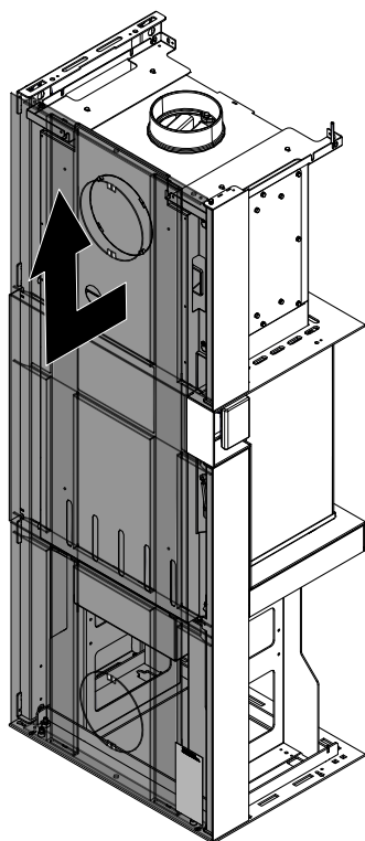
Fig. 38: Rimozione della parete posteriore
