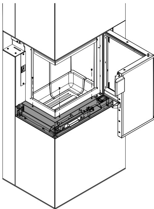
Fig. 41: Smontaggio del diaframma
