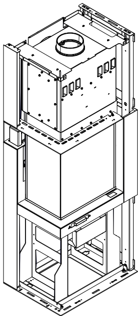
Fig. 36: Rimuovere il coperchio
