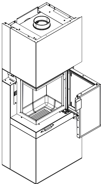
Fig. 40: Apertura dello sportello
