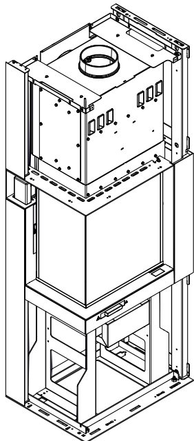
Fig. 15: Rimuovere il coperchio
