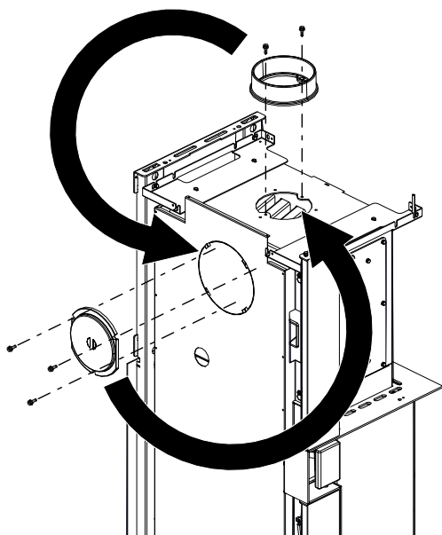
Fig. 13: Sostituire il coperchio e della presa la canna fumaria
