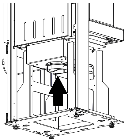
Fig. 19: Fissaggio del tubo Aluflex
