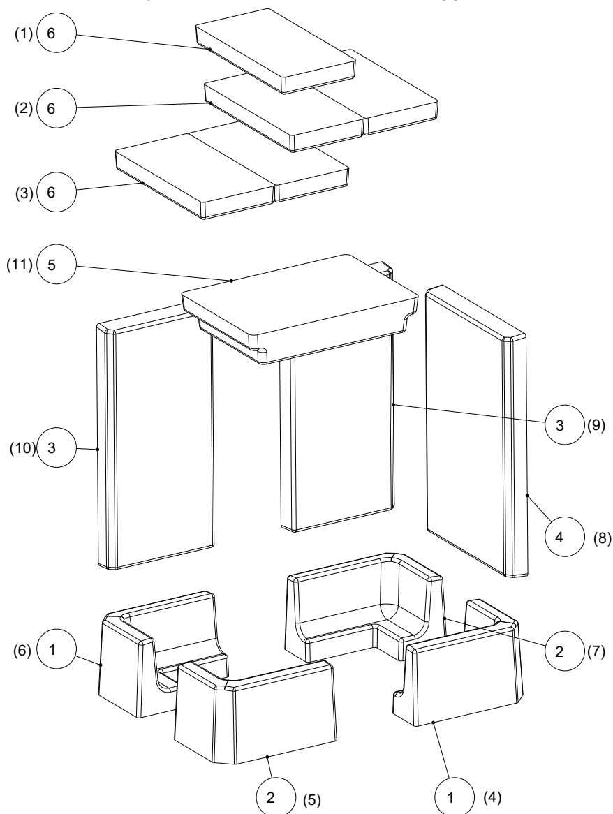
Fig. 20: Montaggio del Keramott
