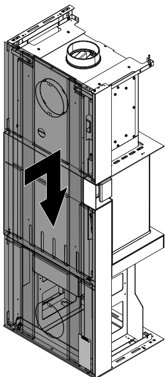
Fig. 9: Montaggio della parete posteriore
