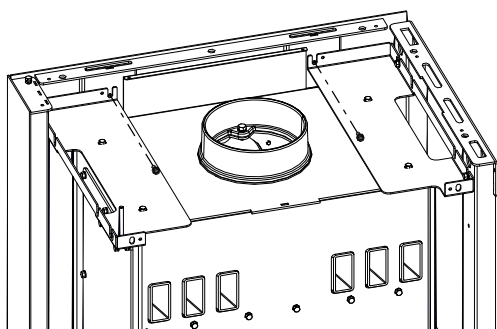
Fig. 10: Fissare il pannello posteriore.
