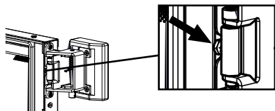
Fig. 27: Regolazione della serratura dello sportello
