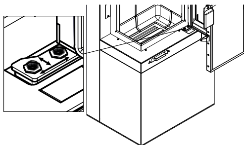
Fig. 24: Regolare la cerniera
