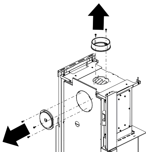
Fig. 12: Smontaggio del coperchio e della presa della canna fumaria
