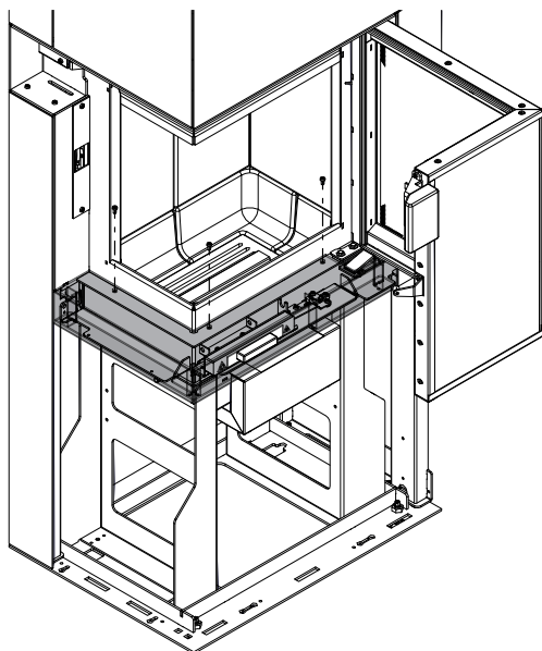
Fig. 43: Smontaggio del diaframma inferiore
