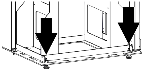
Fig. 21: Allineamento della stufa
