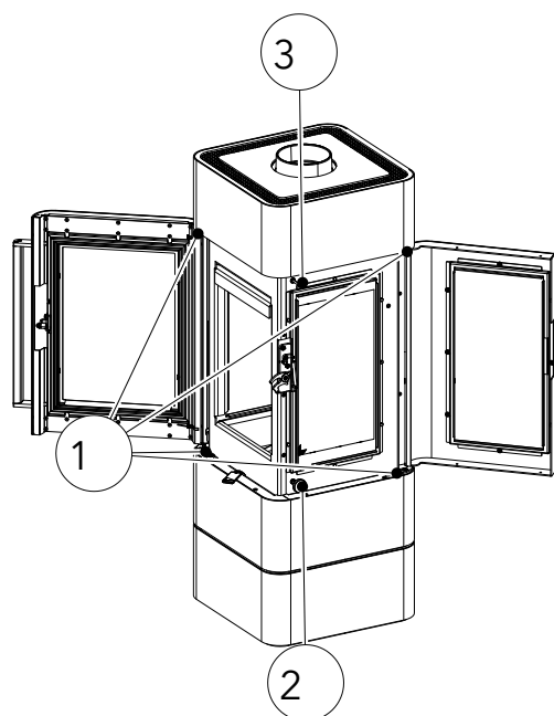
Fig. 25: Régler la porte
