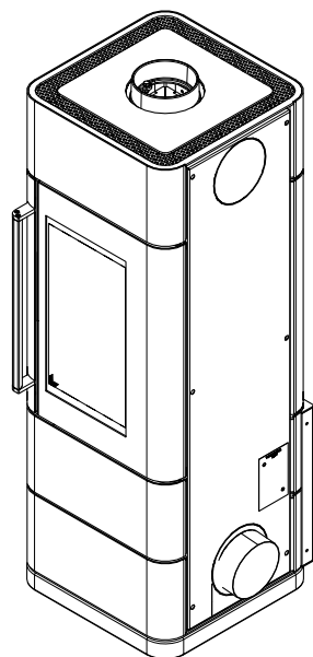
Fig. 24: Installer la paroi arrière
