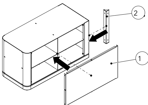
Fig. 16: Installer la paroi arrière et la cornière
