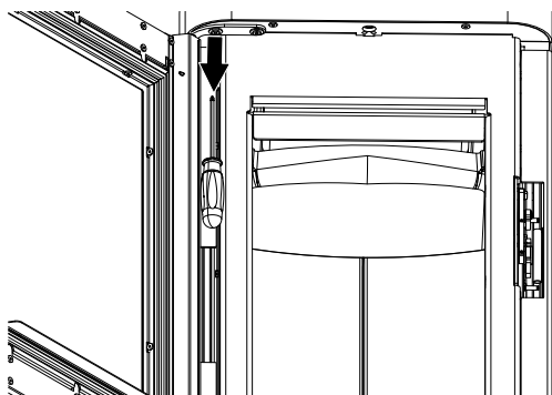
Fig. 39: Ouvrir la porte et dévisser la vis
