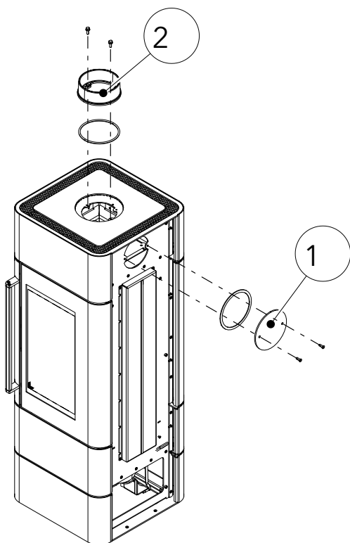
Fig. 8: Démonter le recouvrement et la tubulure
