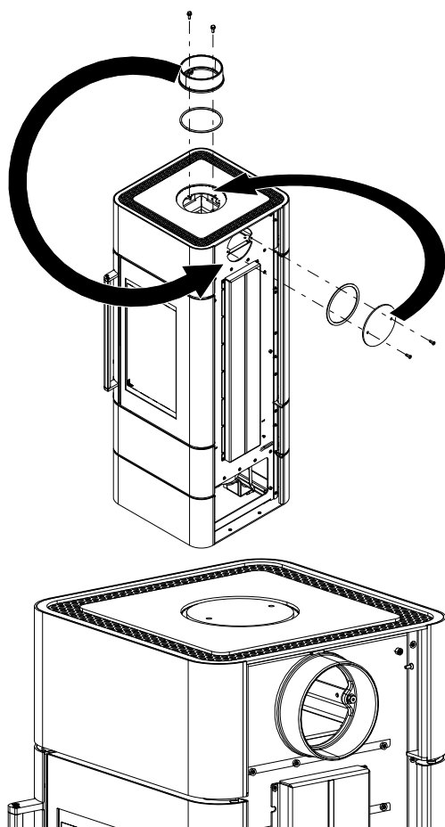
Fig. 9: Interchanger le recouvrement et la tubulure
