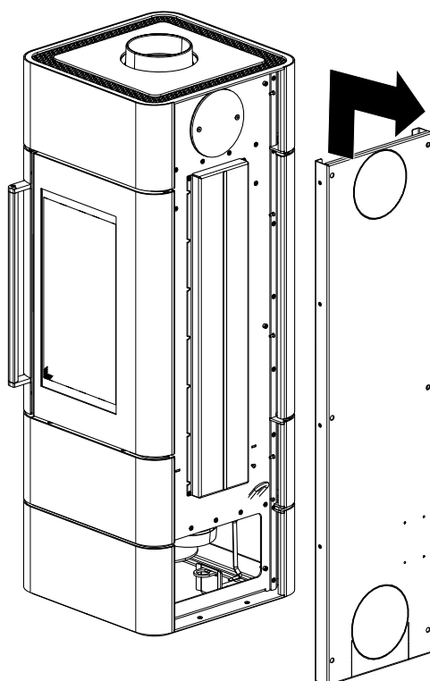
Fig. 38: Enlever la paroi arrière
