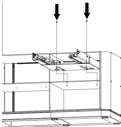
Fig. 19: Installer le support à glissières
