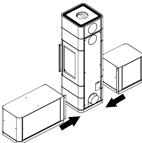
Fig. 17: Fixer l'élément latéral
