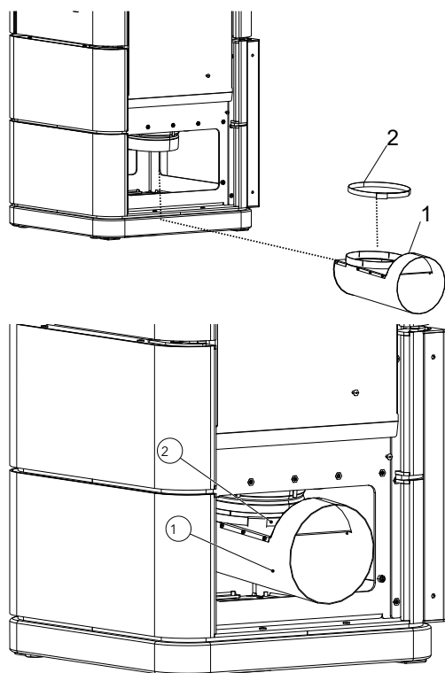
Fig. 23: Installer l'adaptateur d'arrivée d'air
