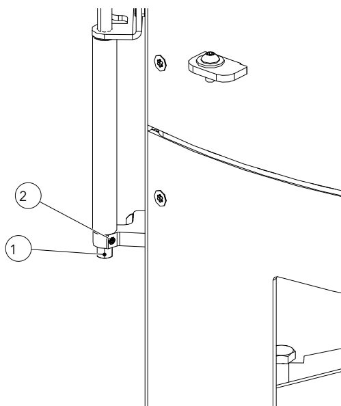
Fig. 29: Régler la force de fermeture de la porte
