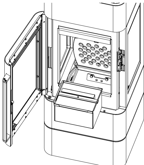
Fig. 36: Enlever et vider le bac à cendres
