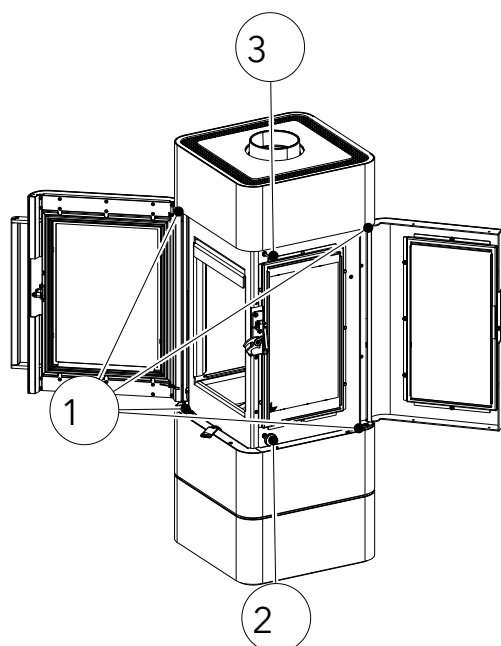
Fig. 15: Regolazione dello sportello
