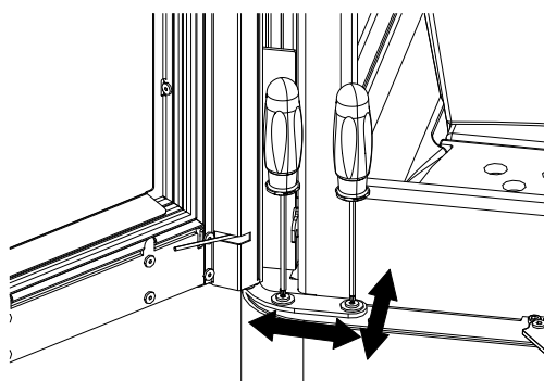
Fig. 16: Pos. 1 regolazione dello sportello
