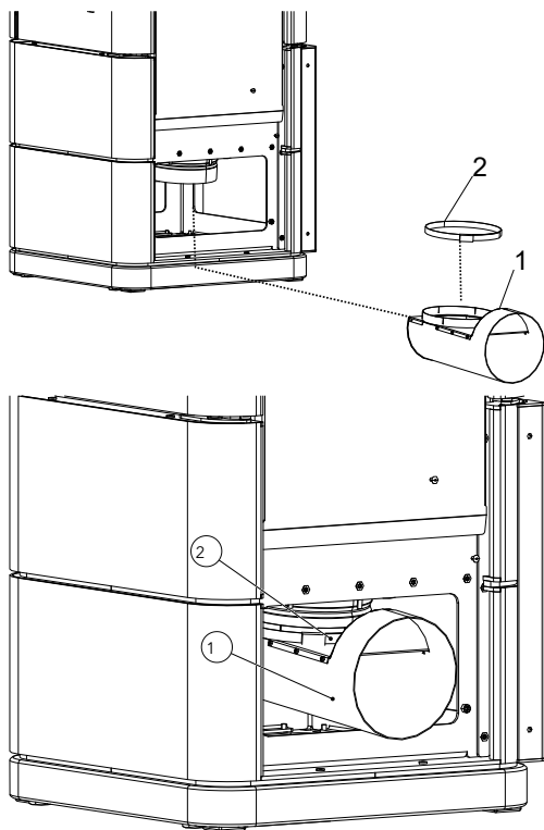
Fig. 13: Montaggio dell'adattatore dell'aria di alimentazione
