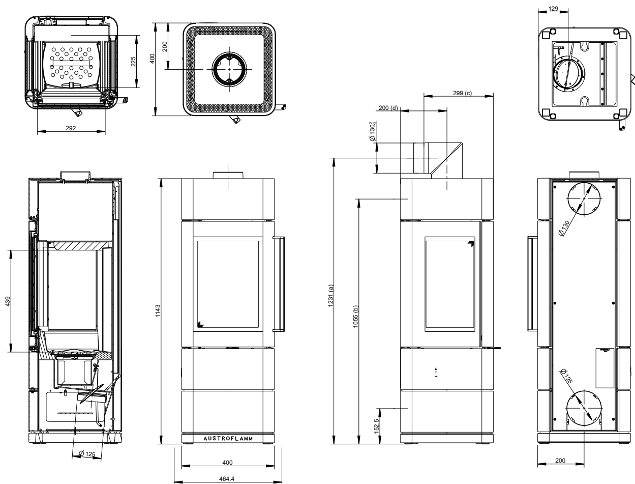
Fig. 1: Dimensioni Ivy
