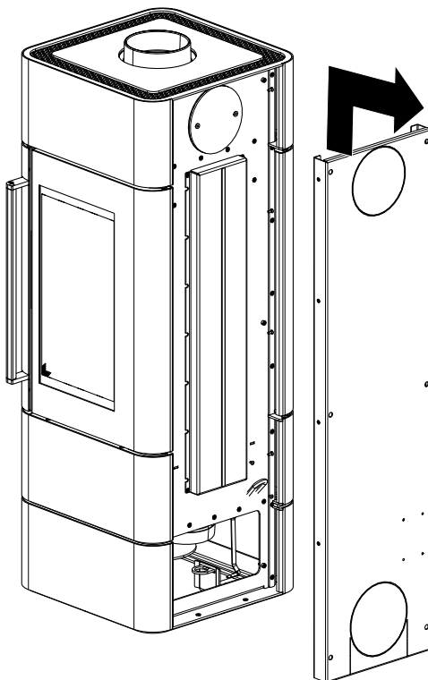
Fig. 28: Rimozione della parete posteriore
