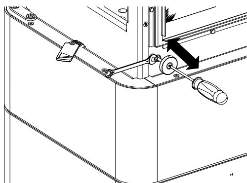
Fig. 17: Pos. 2 regolazione dello sportello
