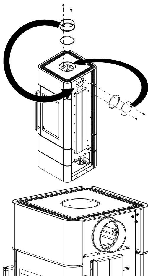
Fig. 9: Sostituzione della copertura e del pezzo di collegamento
