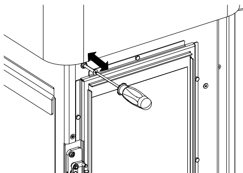
Fig. 18: Pos. 3 regolazione dello sportello
