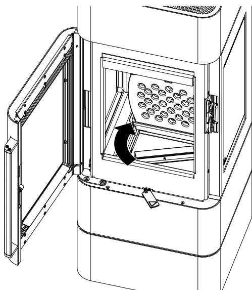
Fig. 24: Coperchio sul box cenere
