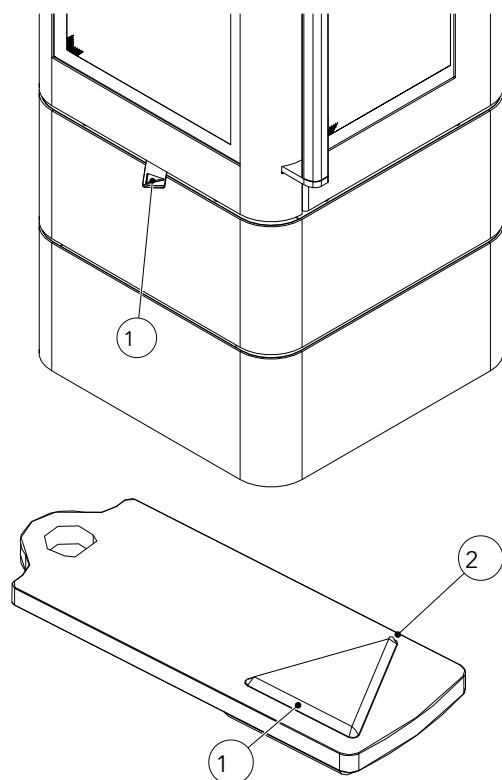
Fig. 20: Regolatore dell'aria primaria/secondaria
