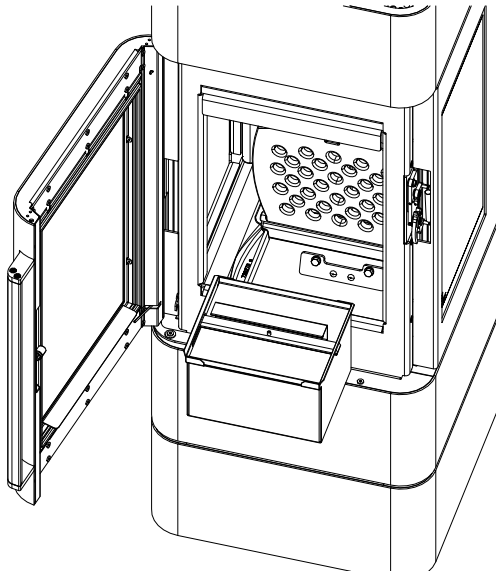
Fig. 26: Rimozione e svuotamento del box cenere
