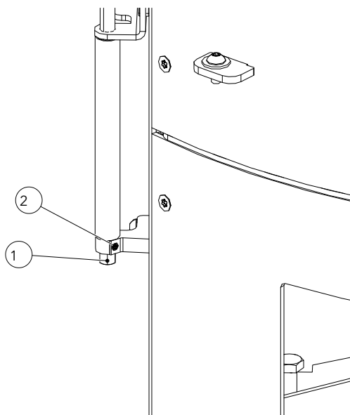
Fig. 19: Regolazione della forza di chiusura dello sportello
