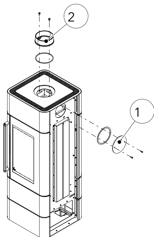
Fig. 8: Smontaggio del coperchio e del pezzo di collegamento
