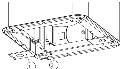
Fig. 5: Sicurezza per il trasporto
