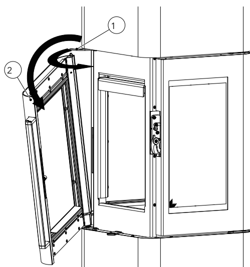
Fig. 40: Rimozione dello sportello
