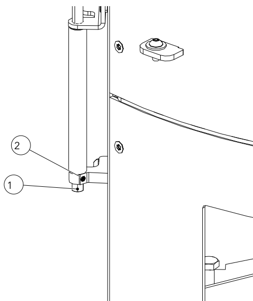
Fig. 29: Regolazione della forza di chiusura dello sportello
