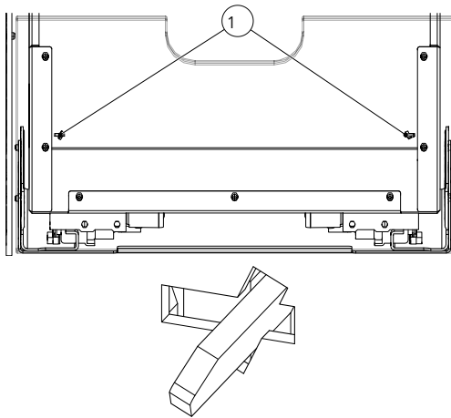
Fig. 21: Perni di fissaggio
