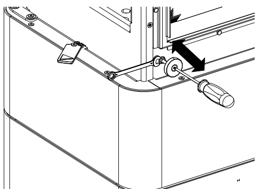
Fig. 27: Pos. 2 regolazione dello sportello
