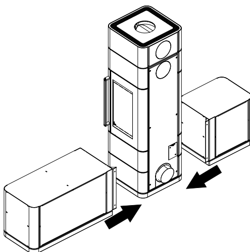
Fig. 17: Montaggio del box laterale
