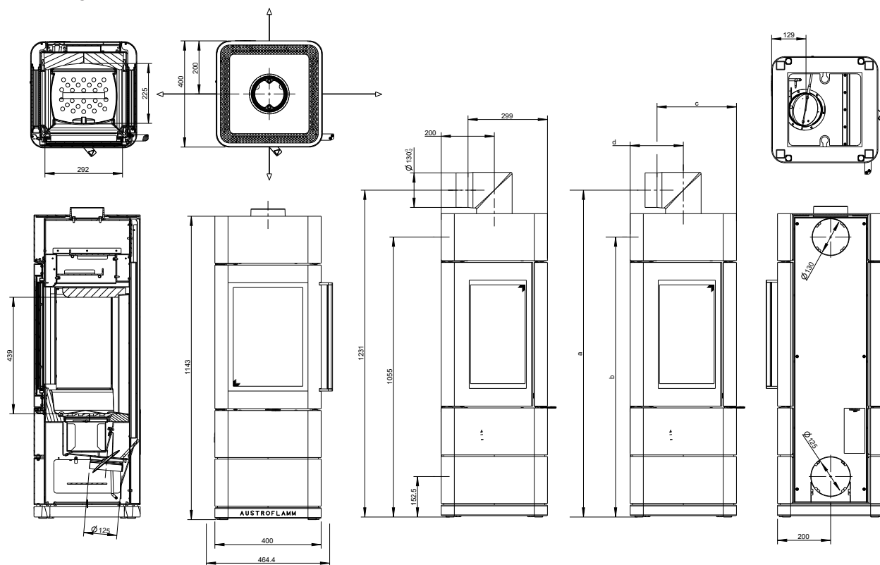
Fig. 1: Dimensioni Ivy
