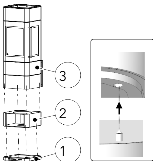
Fig. 14: Montaggio della base
