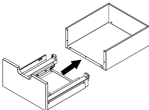
Fig. 18: Rimozione del cassetto di legno dalla guida
