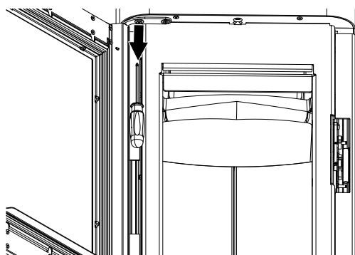
Fig. 39: Apertura dello sportello e svitamento delle viti
