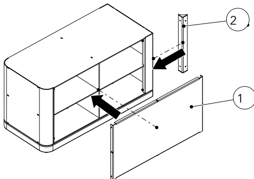
Fig. 16: Montaggio della parete posteriore e dell'angolare
