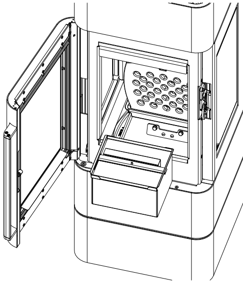
Fig. 36: Rimozione e svuotamento del box cenere
