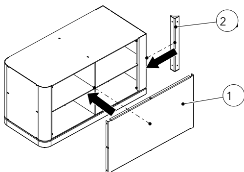
Abb. 17: Rückwand und Winkel montieren
