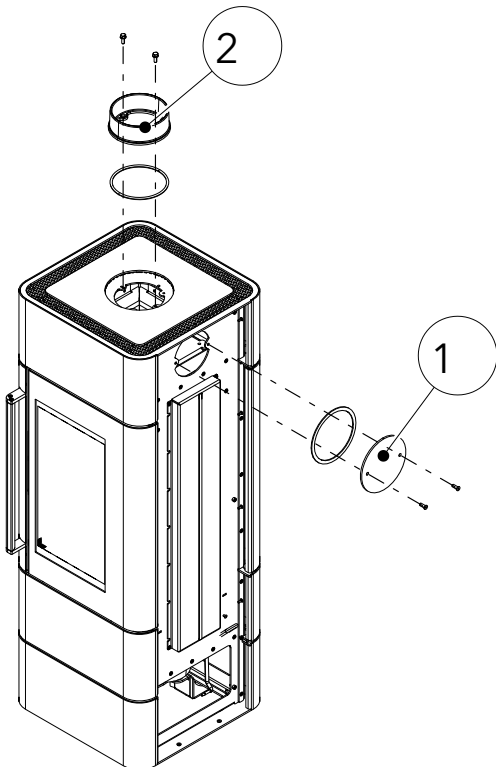
Abb. 9: Abdeckung und Stutzen demontieren
