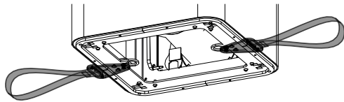
Abb. 7: Transporthilfe
