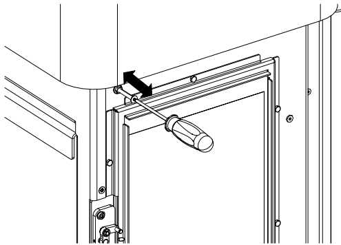
Abb. 29: Pos. 3 Tür einstellen
