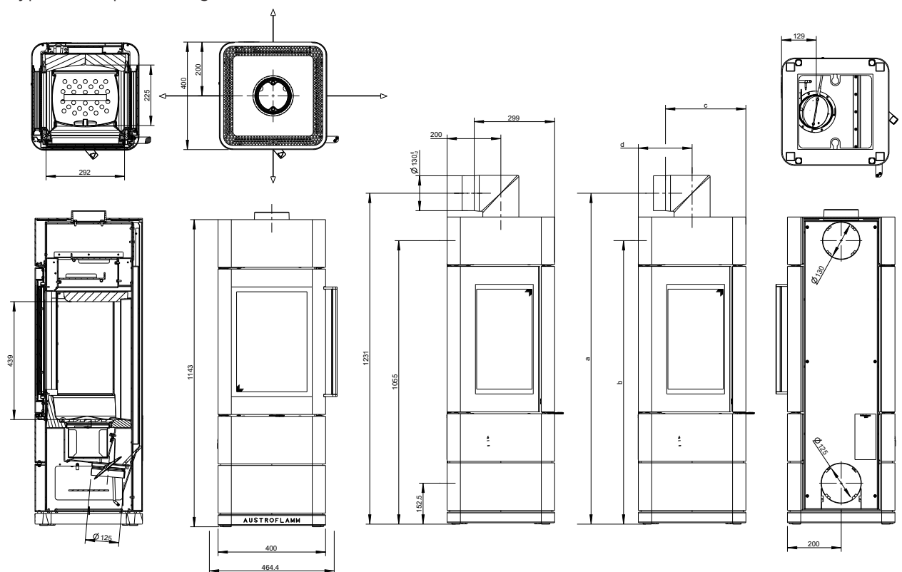
Abb. 2: Abmessungen Ivy
