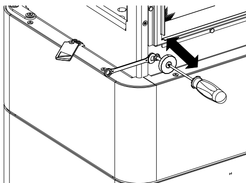
Abb. 28: Pos. 2 Tür einstellen
