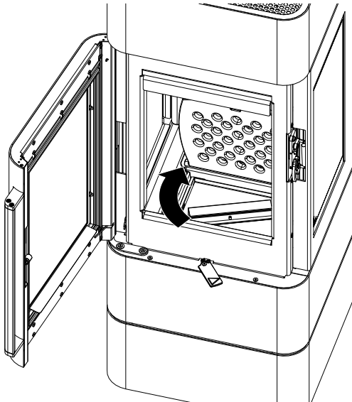
Abb. 35: Deckel auf Aschebox geben
