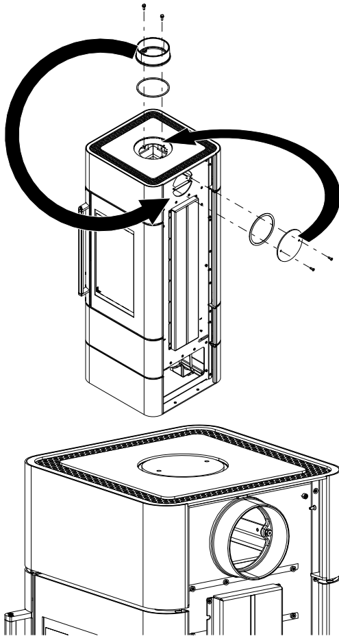
Abb. 10: Abdeckung und Stützen tausche
