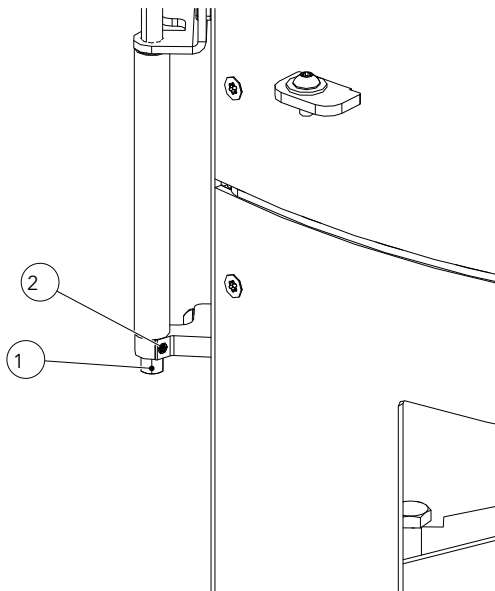
Abb. 30: Türschließkraft einstellen
