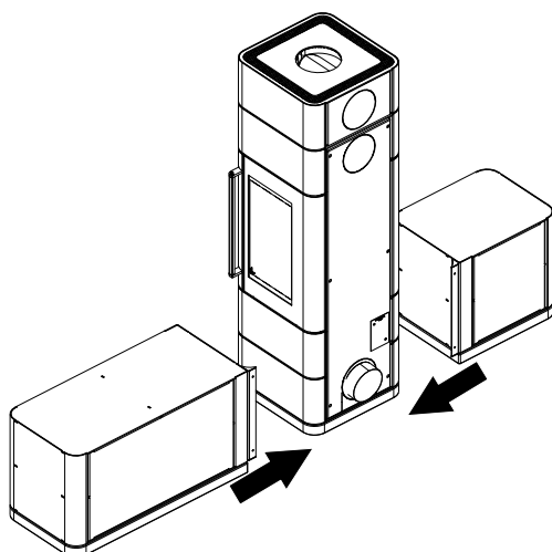
Abb. 18: Beistellbox anbringen
