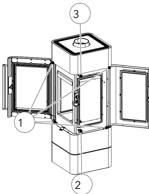
Abb. 26: Tür einstellen
