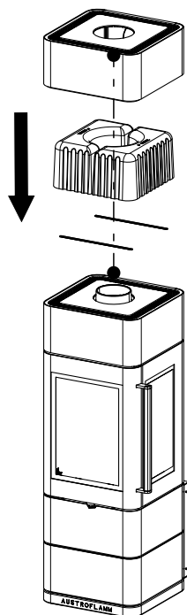
Abb. 12: HMS montieren
