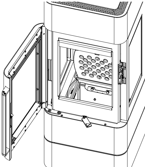
Abb. 34: Rost hochklappen
