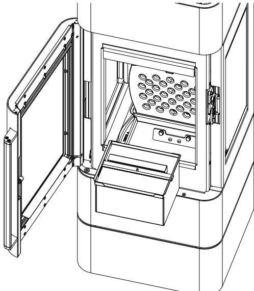
Abb. 37: Aschebox rausnehmen und entleeren
