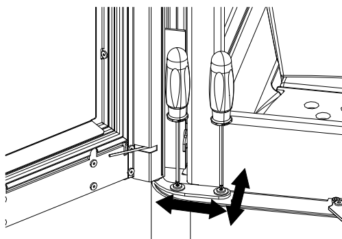
Abb. 27: Pos. 1 Tür einstellen
