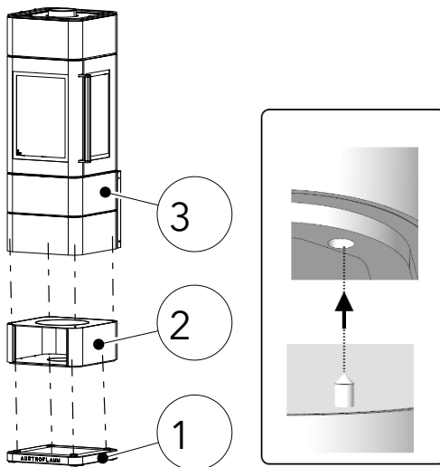
Abb. 15: Sockel montieren
