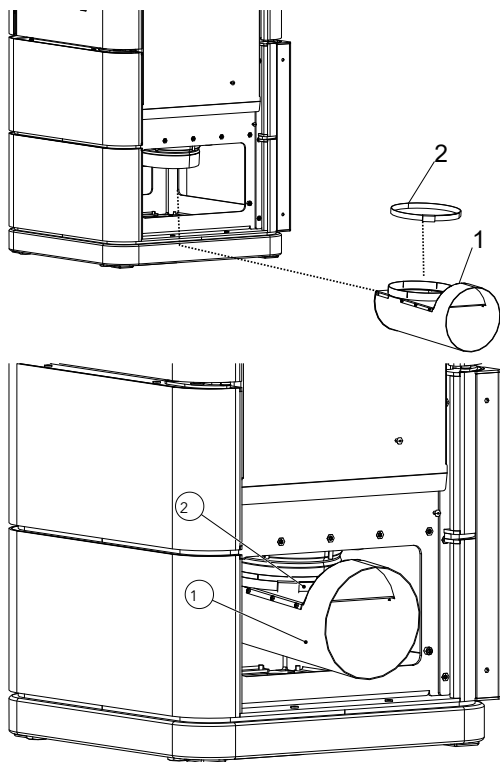
Fig. 25: Installer l'adaptateur d'arrivée d'air
