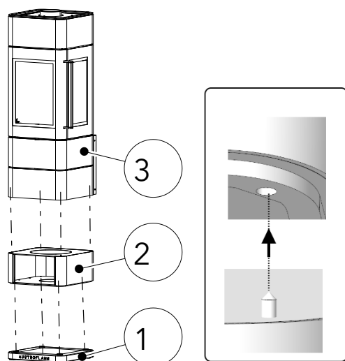
Fig. 16: Installer le socle
