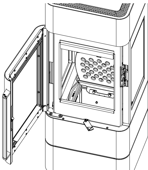
Fig. 36: Relever la grille
