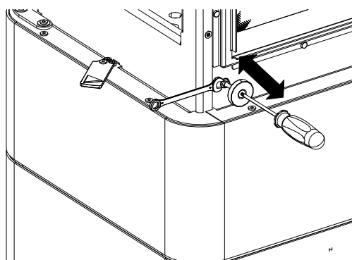
Fig. 29: Pos. 2 Régler la porte
