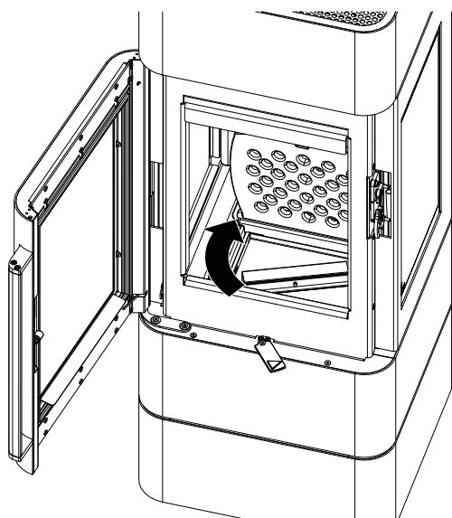
Fig. 37: Mettre le couvercle sur le bac à cendres
