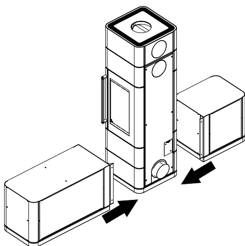
Fig. 19: Fixer l'élément latéral
