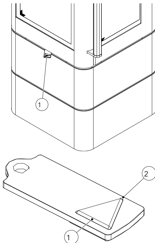
Fig. 32: Manette de régulation de l'air primaire / secondaire
