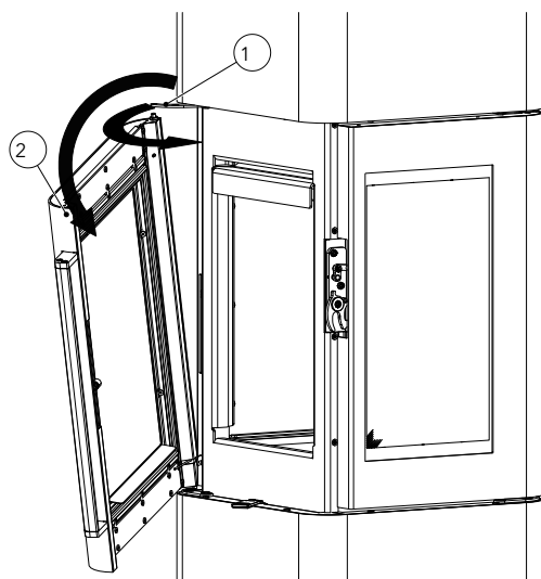
Fig. 43: Décrocher la porte
