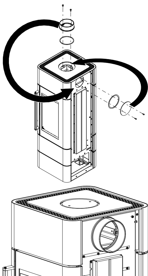
Fig. 11: Interchanger le recouvrement et la tubulure
