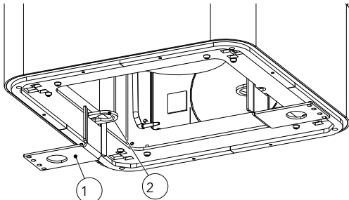
Fig. 7: Sécurité de transport
