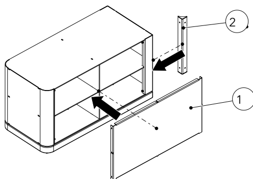
Fig. 18: Installer la paroi arrière et la cornière
