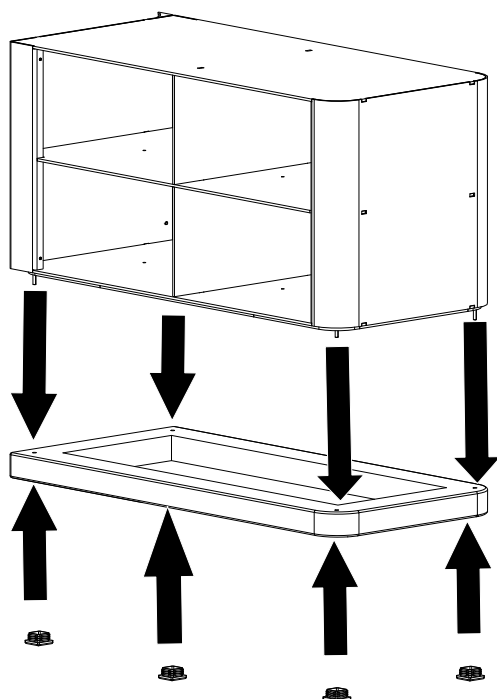
Fig. 17: Installer l'élément latéral
