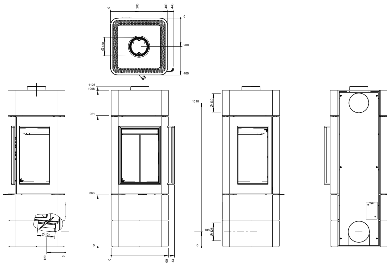
Fig. 1: Dimensions
