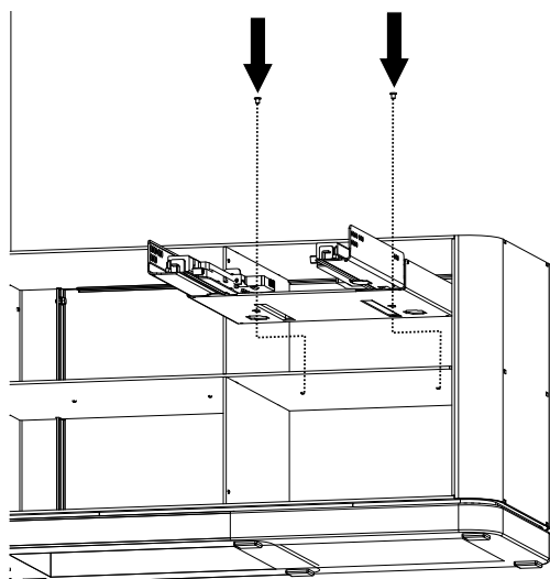
Fig. 21: Installer le support à glissières
