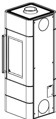
Fig. 12: Installer la protection contre le rayonnement et la paroi arrière
