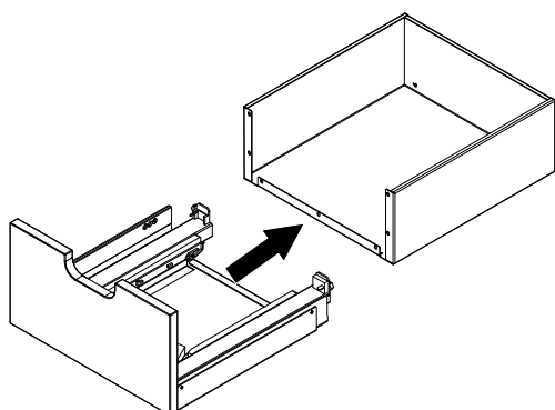
Fig. 20: Séparer le tiroir à bois des glissières
