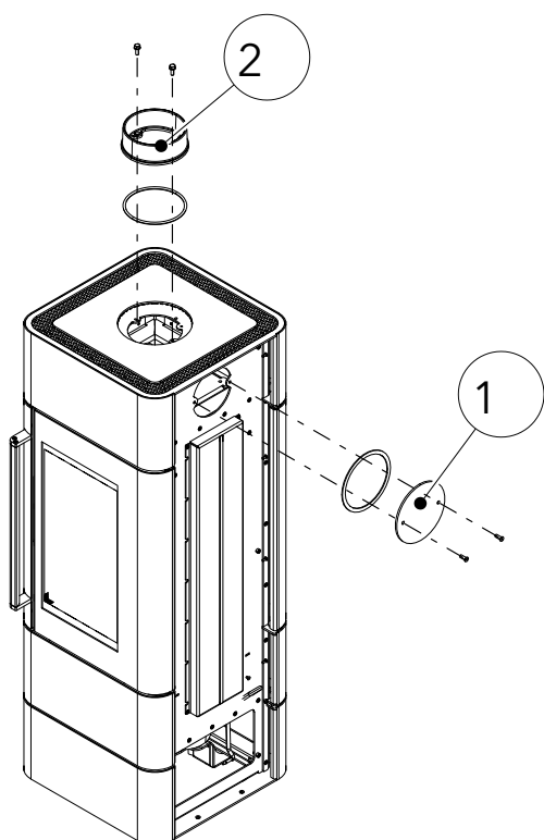
Fig. 10: Démonter le recouvrement et la tubulure
