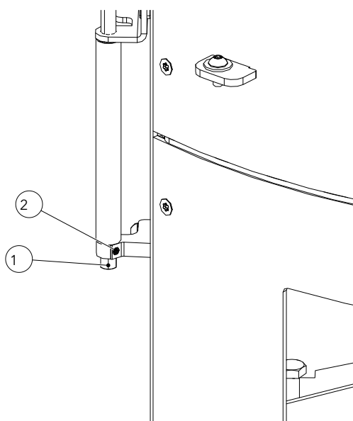
Fig. 31: Régler la force de fermeture de la porte
