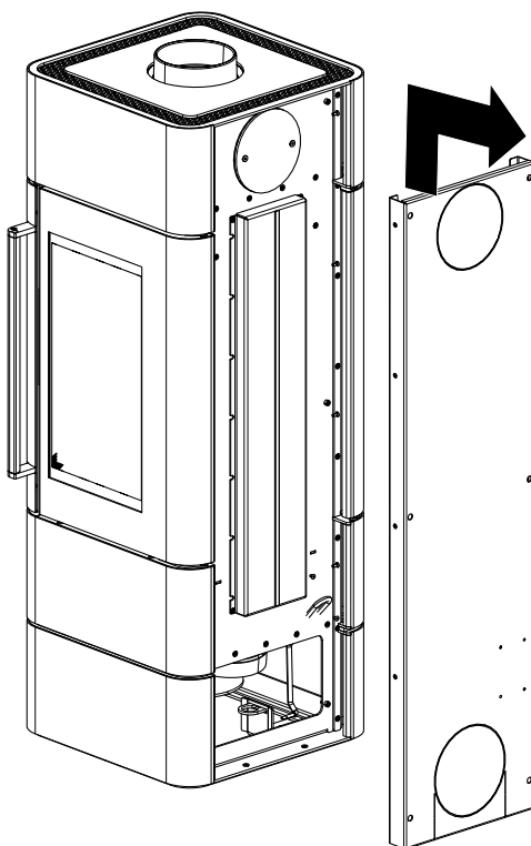
Fig. 41: Enlever la paroi arrière
