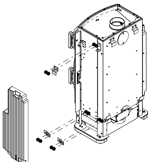
Fig. 22: Installer les fixations HMS et les pierres HMS
