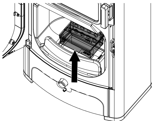
Fig. 54: Enlever et vider le bac à cendres
