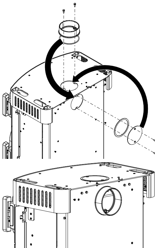
Fig. 13: Interchanger le recouvrement et la tubulure
