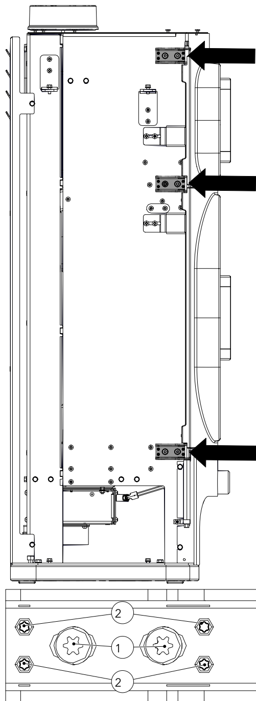
Fig. 40: Vis de réglage
