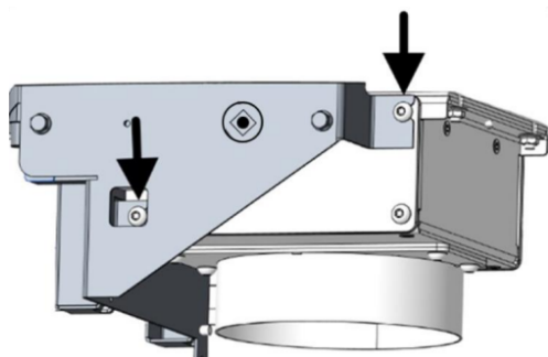
Fig. 37: Unité de commande
