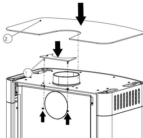
Fig. 7: Installer le plan de cuisson.
