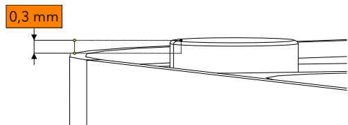
Fig. 15: Tampons en caoutchouc (1) à 0,3 mm.
