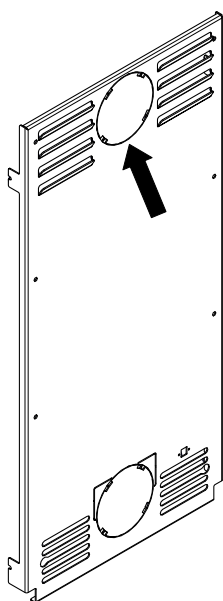
Fig. 10: Enlever la découpe perforée
