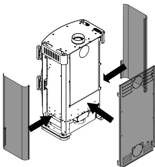
Fig. 18: Installer la paroi arrière et l'habillage latéral
