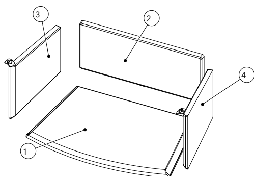
Fig. 26: Compartiment cuisson en Keramott
