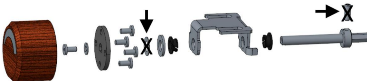
Fig. 36: Modification de la molette
