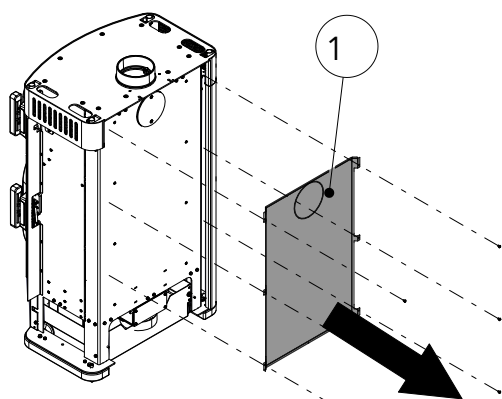
Fig. 17: Installer la protection contre le rayonnement
