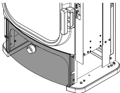
Fig. 32: Fixer le nouveau parement.
