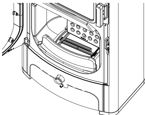
Fig. 53: Fermer le couvercle
