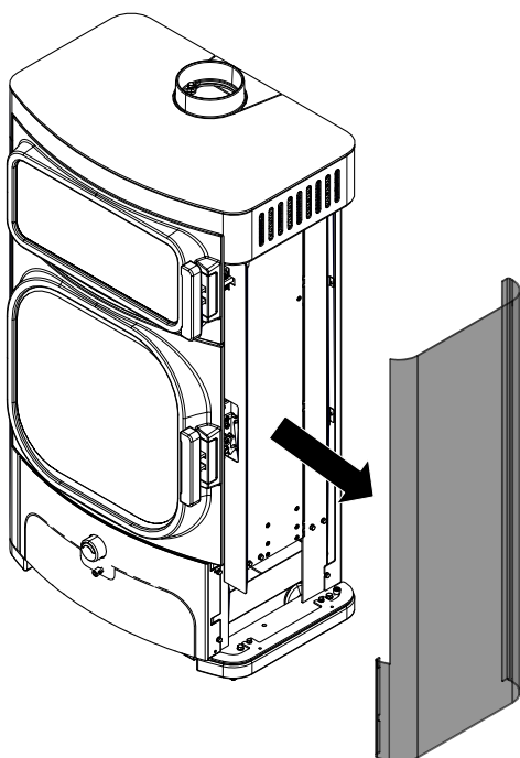
Fig. 57: Enlever l'habillage latéral
