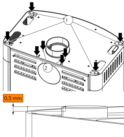
Fig. 6: Ajuster les tampons en caoutchouc
