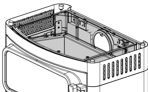
Fig. 50: Nettoyer les canaux de circulation des fumées
