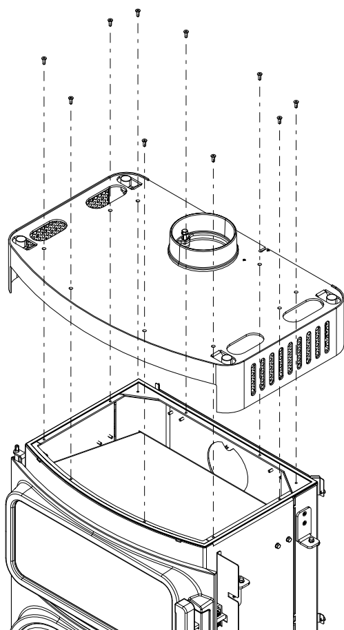
Fig. 49: Déposer le couvercle
