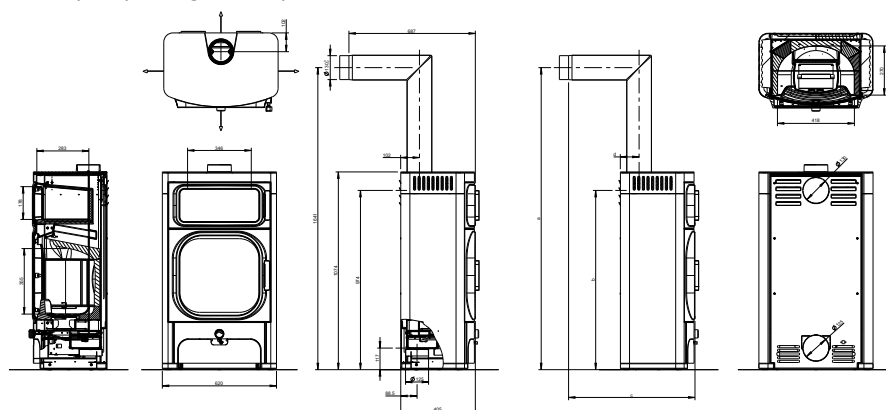
Fig. 1: Dimensions de l'appareil de base
