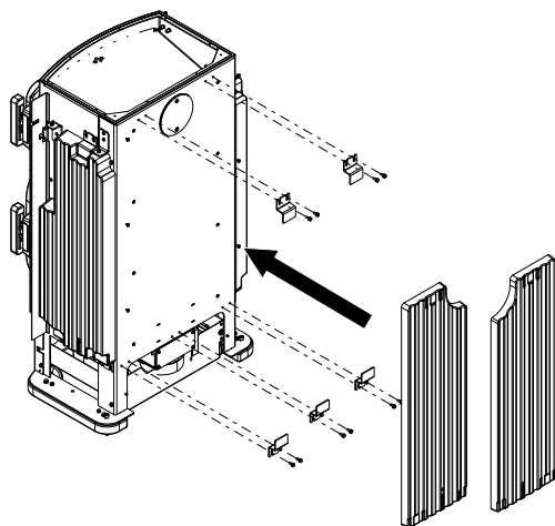
Fig. 23: Poser la pierre HMS à l'arrière
