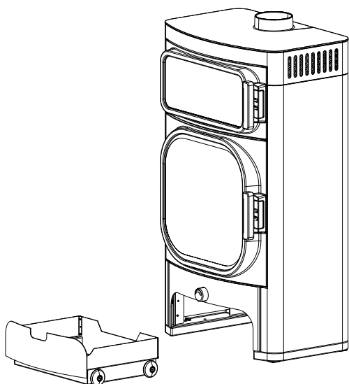
Fig. 30: Insérer le tiroir à bois
