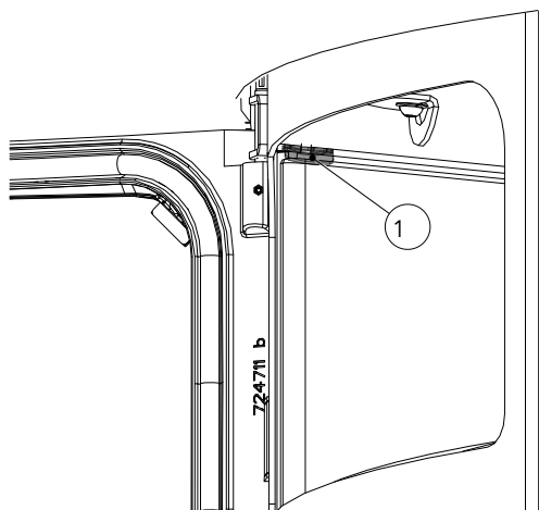
Fig. 27: Fixation pour pierres en Keramott
