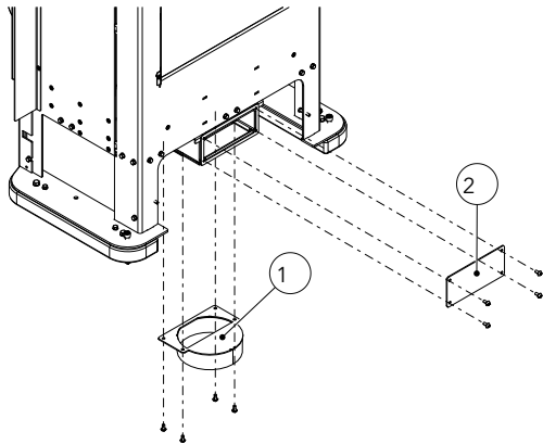
Fig. 28: Démontez le collet d'arrivée d'air
