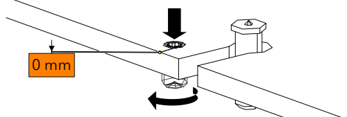
Fig. 16: Vis de réglage (2) à 0 mm
