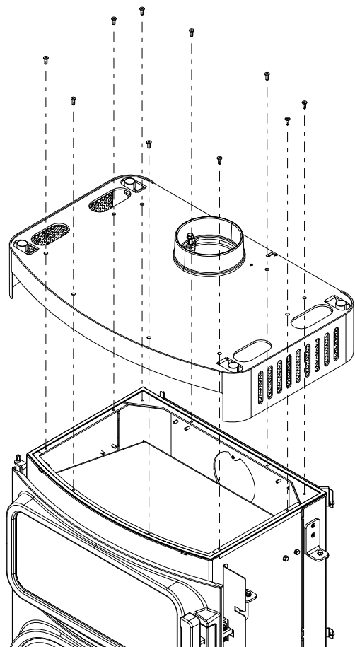
Fig. 21: Déposer le couvercle
