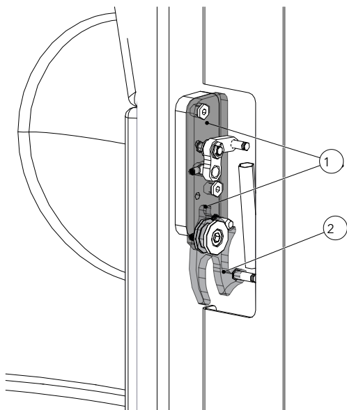
Fig. 42: Régler la serrure de la porte
