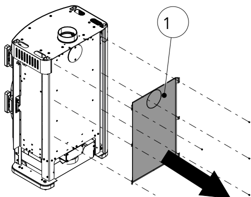
Fig. 20: Démontez la protection contre le rayonnement
