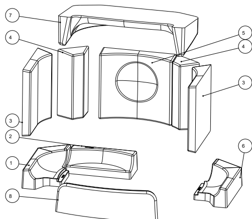
Fig. 25: Chambre de combustion en Keramott
