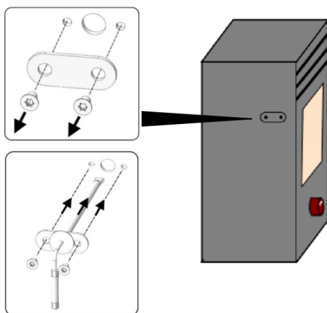
Fig. 35: Fixer le capteur de temp. de la chambre de combustion
