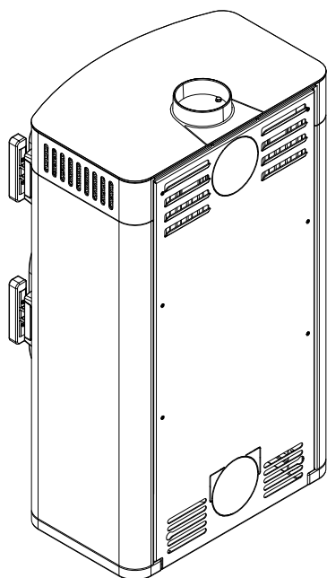
Fig. 24: Installer l'habillage latéral, le couvercle et le plan de cuisson
