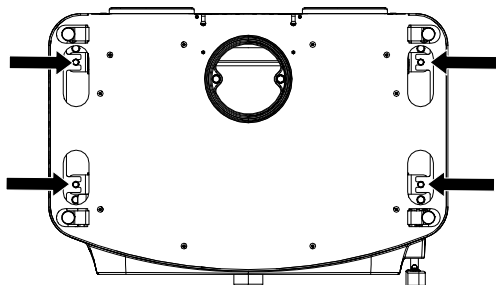
Fig. 55: Dévisser les vis par le haut
