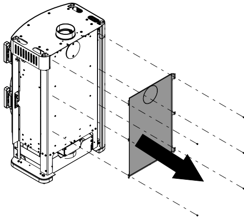
Fig. 11: Démonter la protection contre le rayonnement
