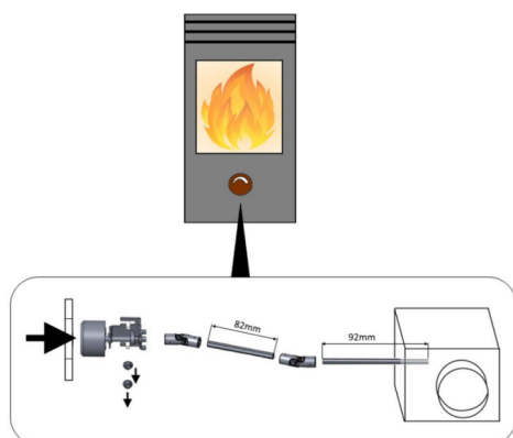
Fig. 34: Déposer la molette
