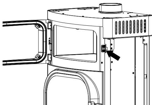
Fig. 43: Régler la serrure de la porte
