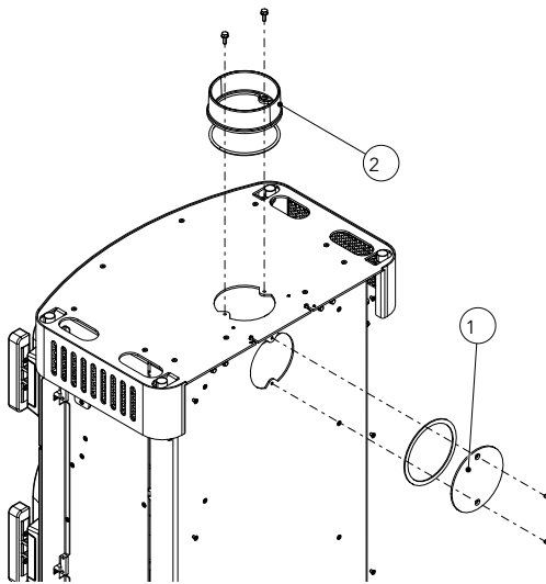
Fig. 12: Démonter le recouvrement et la tubulure
