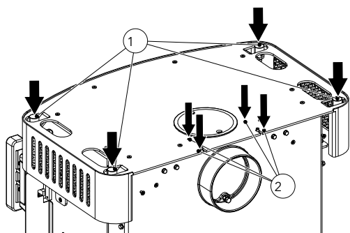
Fig. 14: Ajuster les tampons en caoutchouc et les vis de réglage
