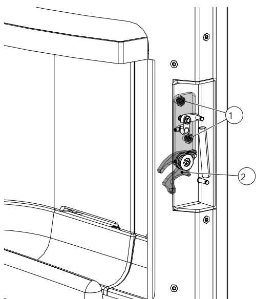
Fig. 38: Régler la serrure de la porte
