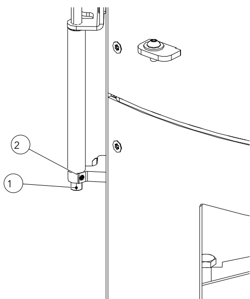
Fig. 37: Régler la force de fermeture de la porte
