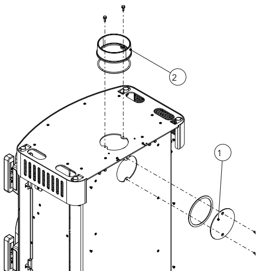
Fig. 13: Démonter le recouvrement et la tubulure
