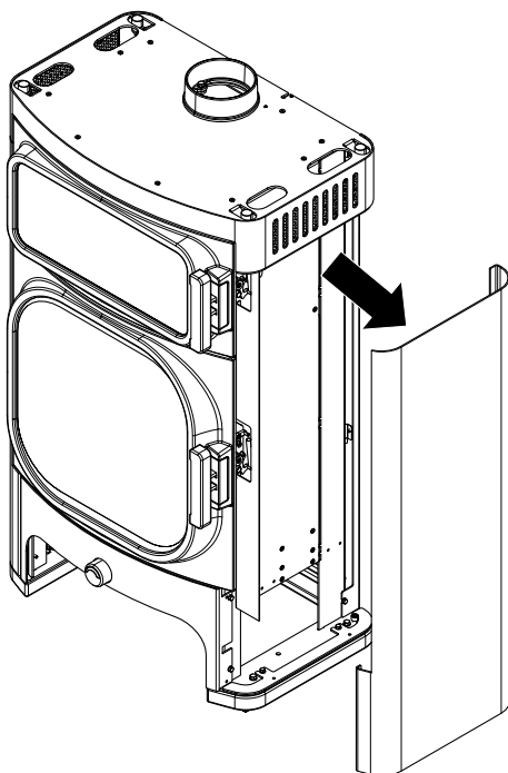
Fig. 49: Enlever l'habillage latéral
