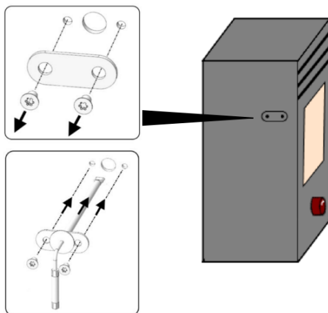
Fig. 31: Fixer le capteur de temp. de la chambre de combustion
