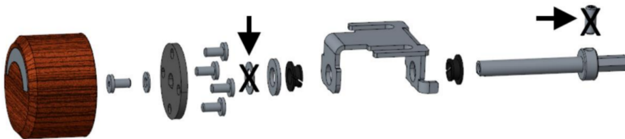
Fig. 32: Modification de la molette
