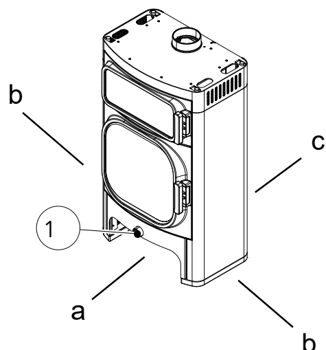
Fig. 2: Distances de sécurité (a,b,c) / manette de régulation de l'air
