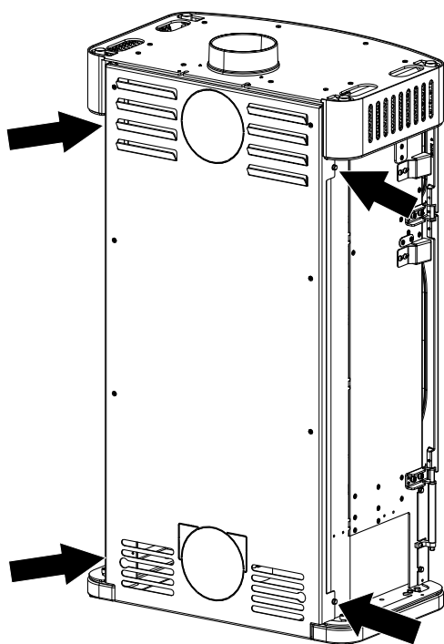
Fig. 50: Dévisser les vis gauche et droite de la paroi arrière
