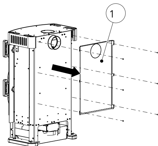
Fig. 21: Démontez la protection contre le rayonnement
