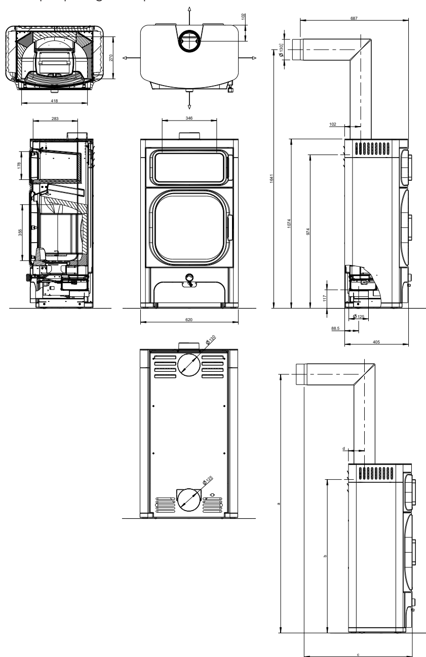
Fig. 1: Dimensions
