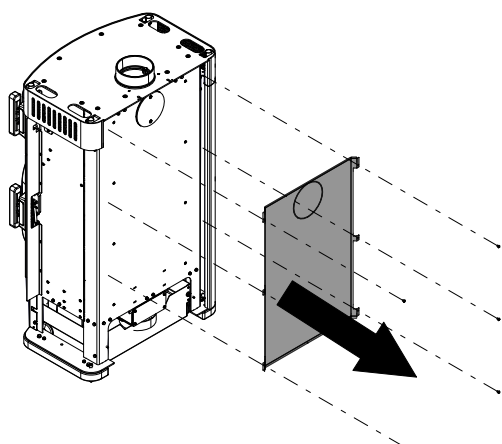
Fig. 11: Smontaggio della protezione anti-irradiazione
