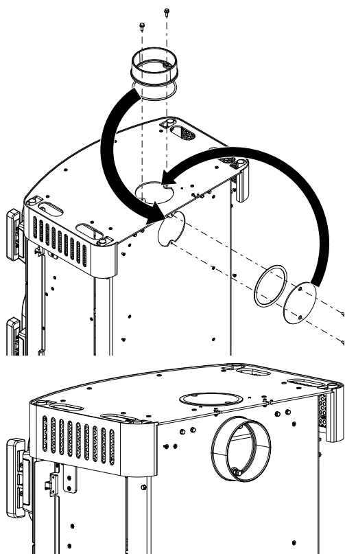
Fig. 13: Sostituzione della copertura e del pezzo di collegamento
