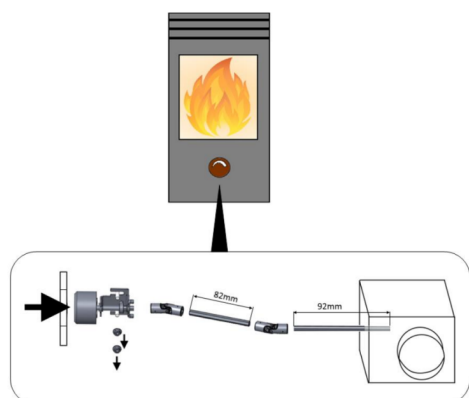
Fig. 34: Rimozione dell'unità del controllo rotativo
