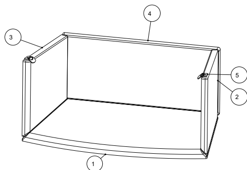
Fig. 26: Keramott - scomparto di cottura
