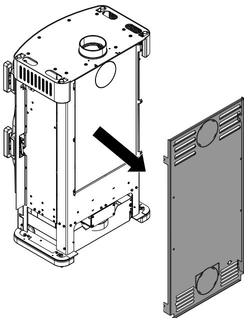
Fig. 59: Rimozione della parete posteriore
