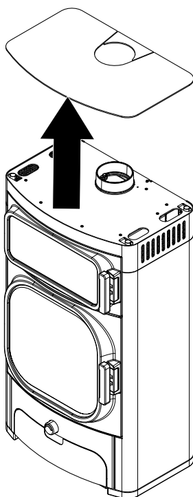
Fig. 48: Rimuovere la piastra di cottura
