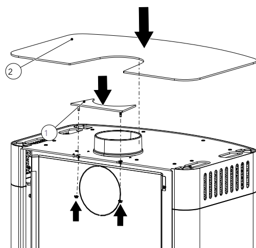
Fig. 7: Posizionamento della piastra di cottura
