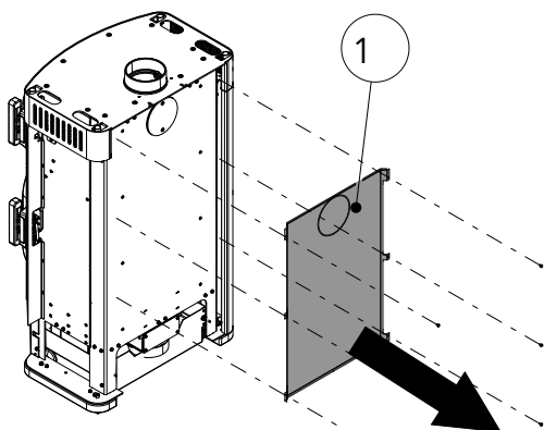
Fig. 20: Smontaggio della protezione anti-irraggiamento
