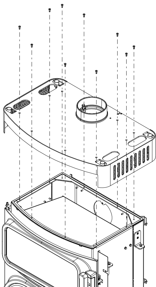
Fig. 49: Smontaggio del coperchio
