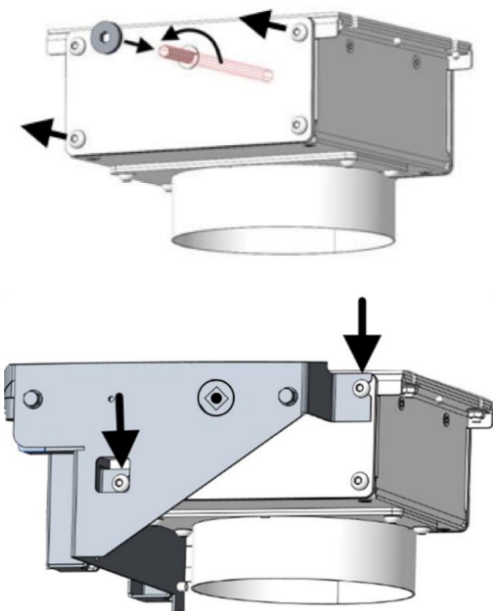
Fig. 37: Unità di comando
