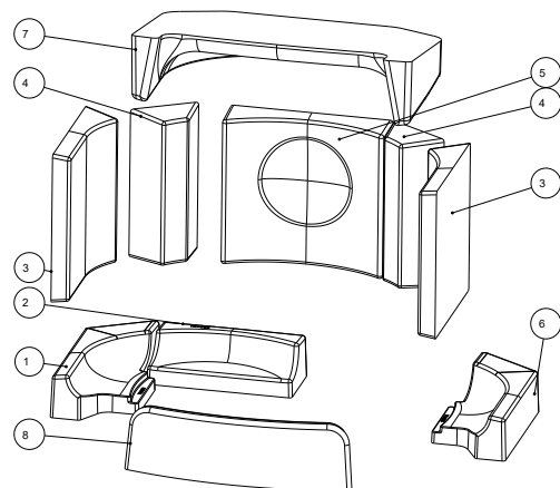
Fig. 25: Keramott - camera di combustione
