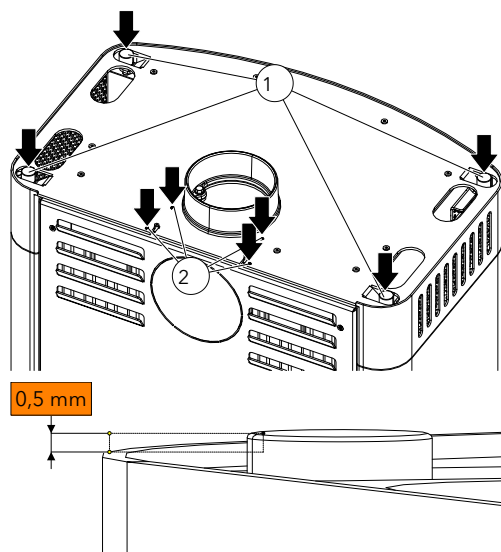
Fig. 6: Regolazione del tampone di gomma
