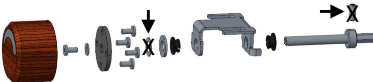
Fig. 36: Modifica dell'unità del controllo rotativo
