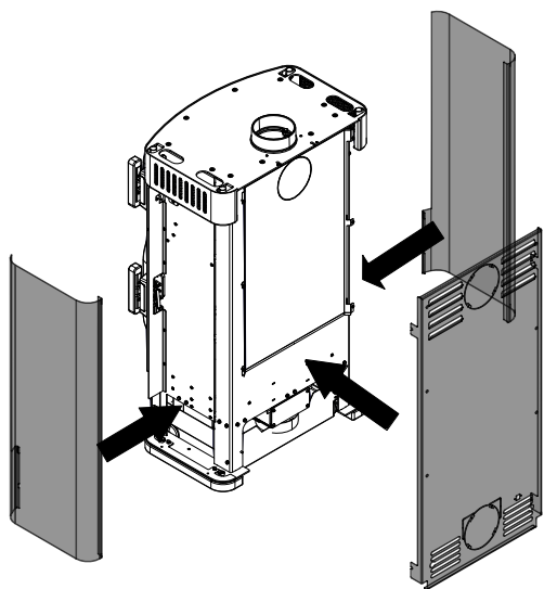
Fig. 18: Montaggio della parete posteriore e del rivestimento laterale
