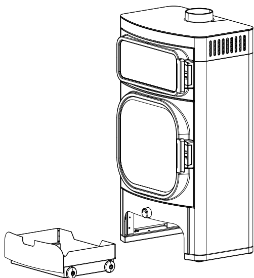
Fig. 30: Inserimento del cassetto in legno
