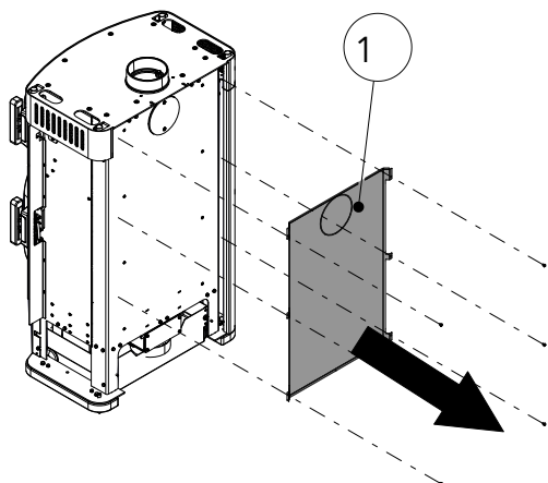
Fig. 17: Montaggio della protezione anti-irraggiamento
