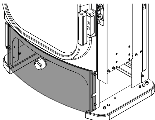
Fig. 32: Fissare il pannello/diaframma nuovo.
