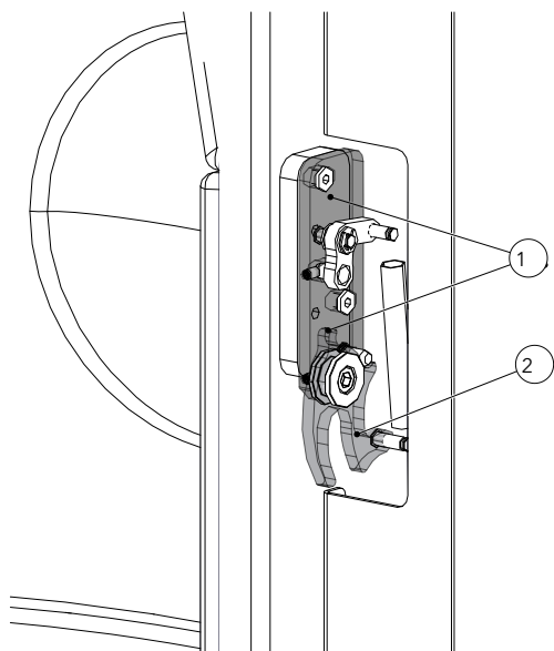
Fig. 42: Regolazione della serratura dello sportello
