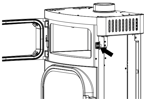
Fig. 43: Regolazione della serratura dello sportello
