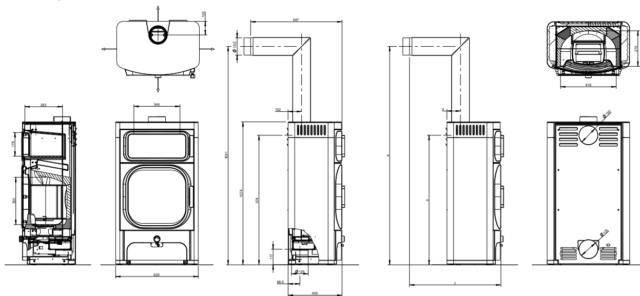
Fig. 2: Dimensioni dell'apparecchio di base
