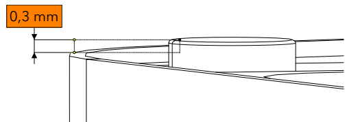
Fig. 15: Tampone di gomma (1) su 0,3 mm
