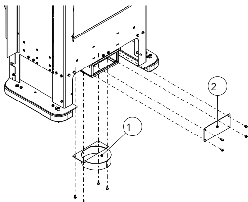
Fig. 28: Smontare la flangia dell'aria di alimentazione
