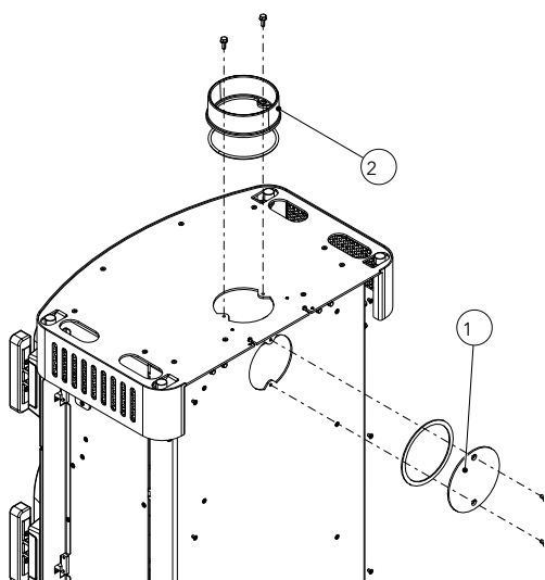
Fig. 12: Smontaggio del coperchio e del pezzo di collegamento
