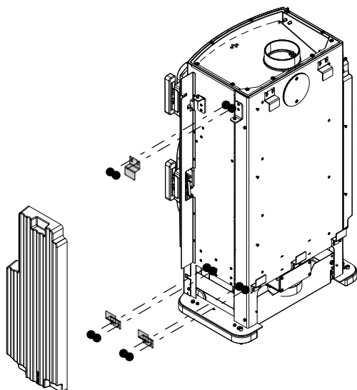
Fig. 22: Montare i supporti HMS e la pietra HMS.
