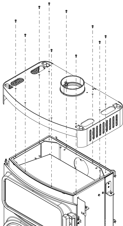
Fig. 21: Smontaggio del coperchio
