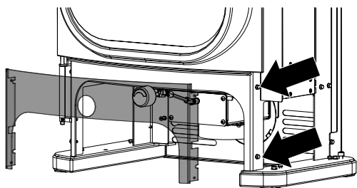
Fig. 31: Rimozione del pannello
