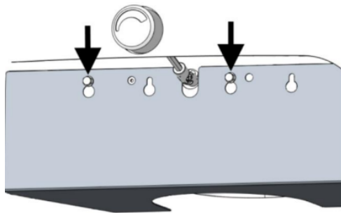
Fig. 38: Montaggio della copertura
