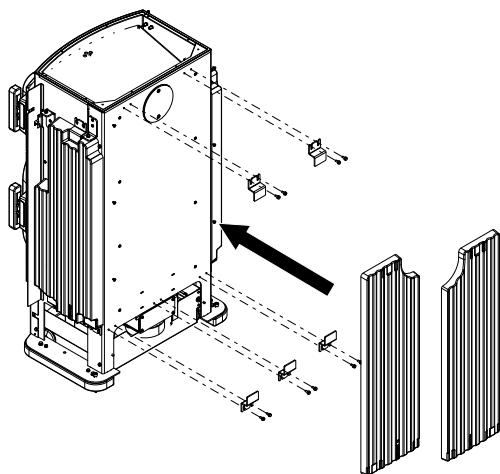
Fig. 23: Montaggio della pietra HMS sul retro
