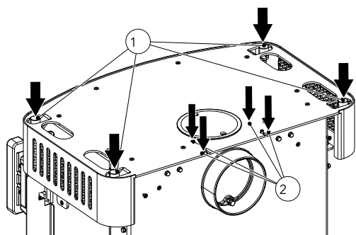
Fig. 14: Regolazione del tampone in gomma e delle viti di regolazione
