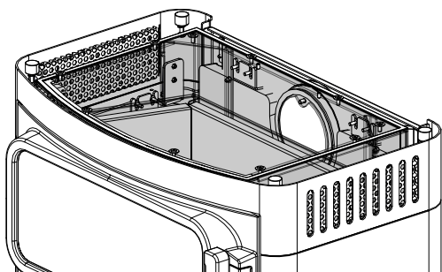
Fig. 50: Pulire i passaggi dei gas di scarico
