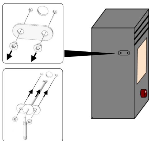
Fig. 35: Fissaggio del sensore di temperatura della camera di combustione
