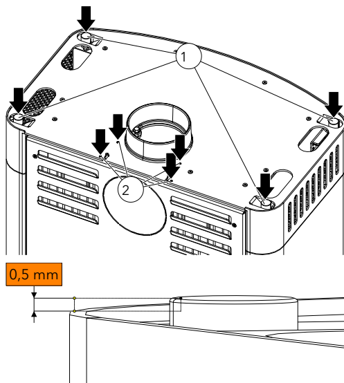
Abb. 6: Gummipuffer einstellen
