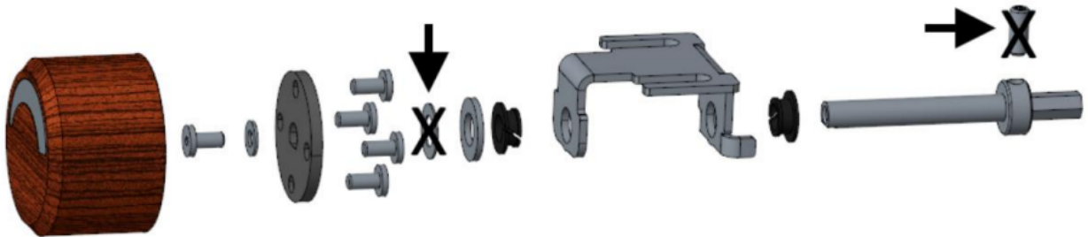
Abb. 36: Umbau Drehreglereinheit
