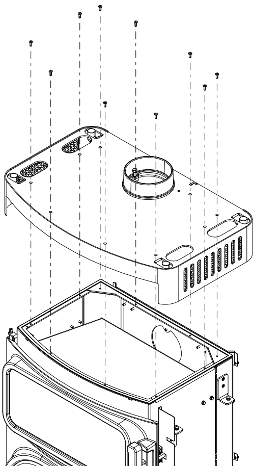
Abb. 21: Deckel abmontieren
