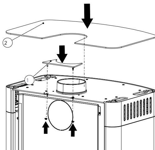
Abb. 7: Kochfeld anbringen
