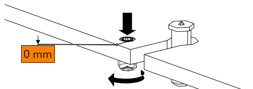
Abb. 16: Einstellschrauben (2) auf 0 mm
