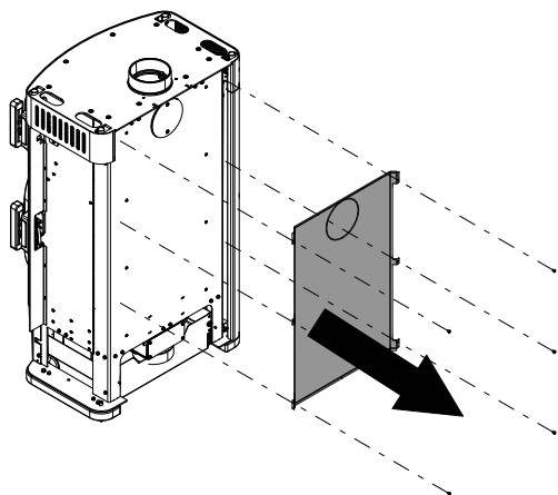
Abb. 11: Strahlungsschutz demontieren
