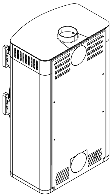
Abb. 24: Seitenverkleidung, Deckel und Kochfeld anbringen
