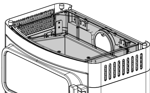
Abb. 50: Rauchgaswege reinigen
