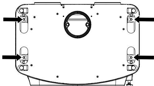
Abb. 55: Von oben die Schrauben lösen
