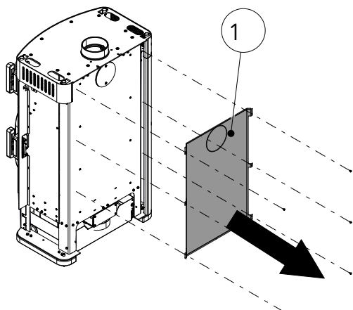
Abb. 17: Strahlungsschutz montieren
