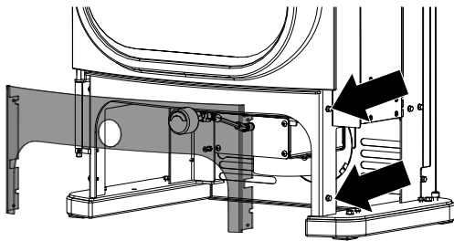
Abb. 31: Blende abnehmen
