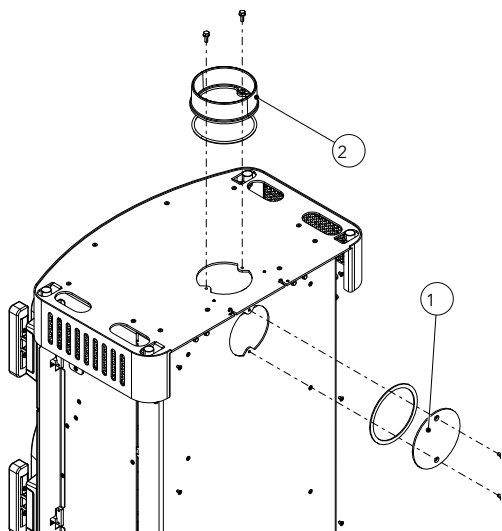
Abb. 12: Abdeckung und Stutzen demontieren
