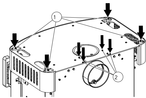
Abb. 14: Gummipuffer und Einstellschrauben einstellen
