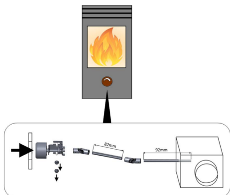
Abb. 34: Drehreglereinheit ausbauen
