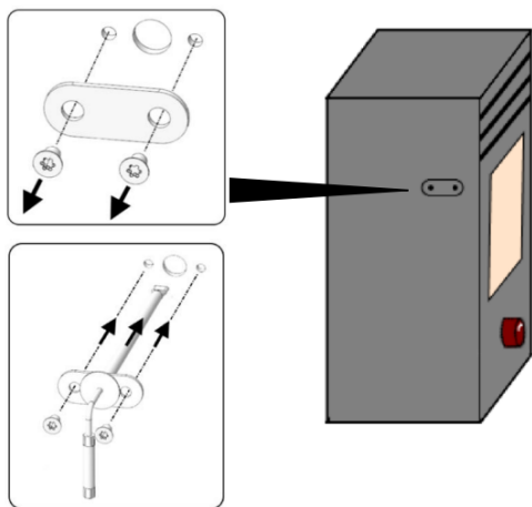
Abb. 35: Feuerraumtemp.fühler befestigen
