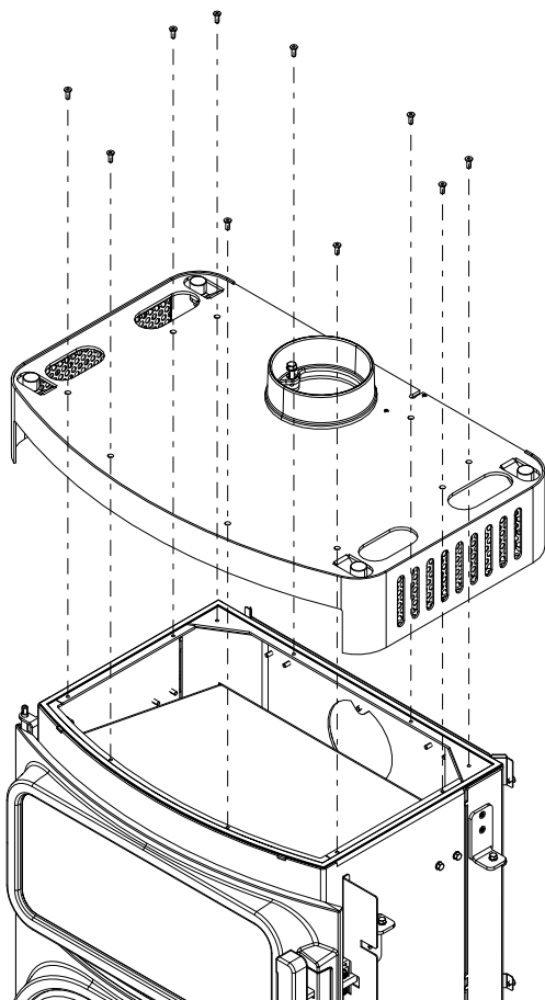
Abb. 49: Deckel abmontieren
