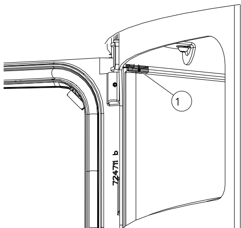
Abb. 27: Halter für Keramott-Steine
