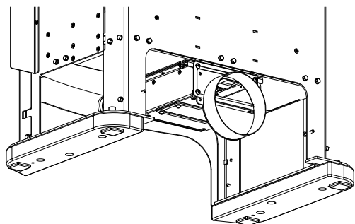
Abb. 29: Teile getauscht
