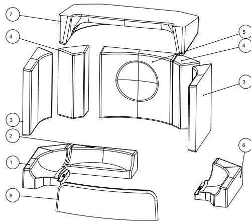
Abb. 25: Keramott Feuerraum
