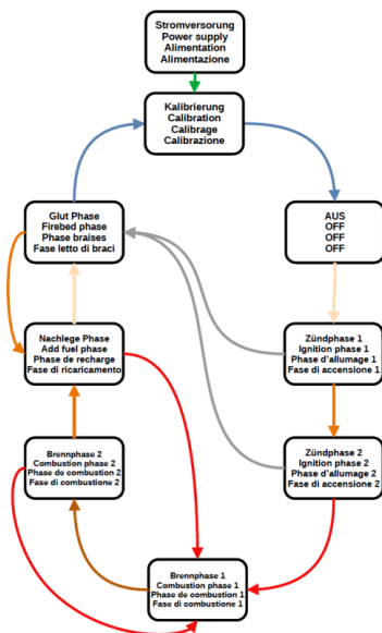
Abb. 39: Phase
