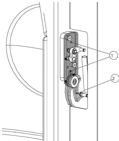
Abb. 42: Türverschluss einstellen
