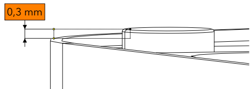
Abb. 15: Gummipuffer (1) auf 0,3 mm
