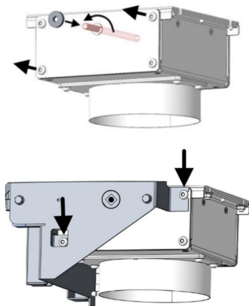
Abb. 37: Steuereinheit
