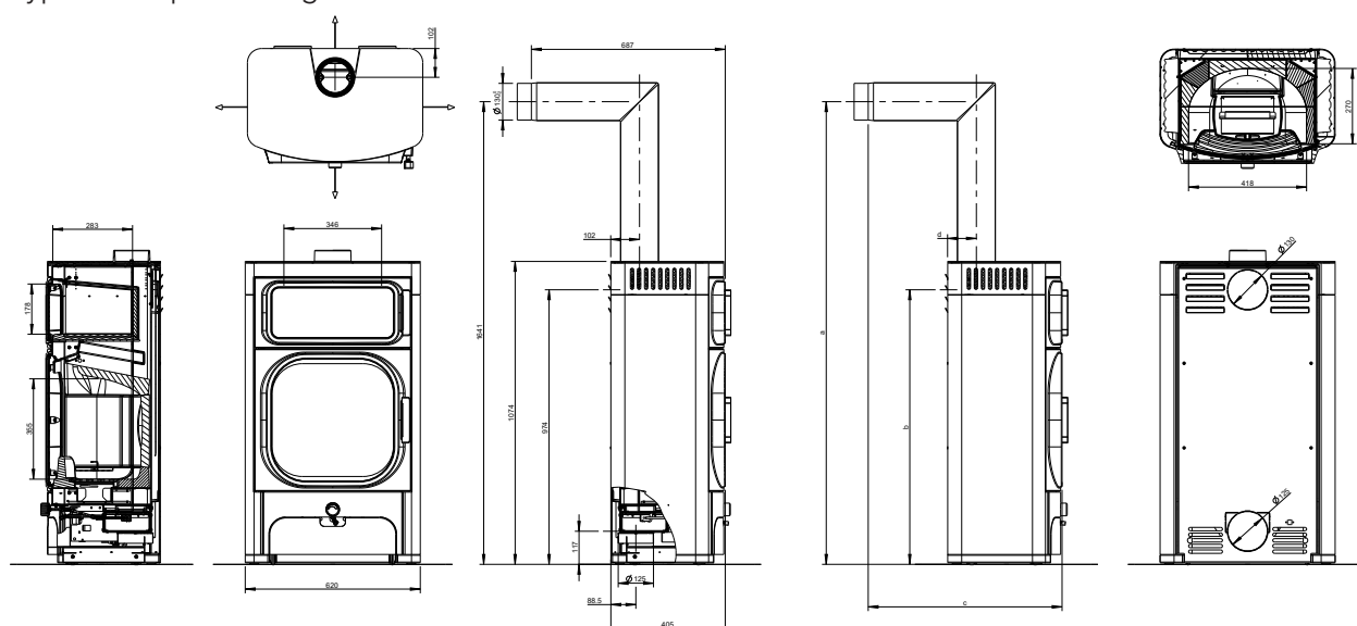
Abb. 2: Abmessungen Grundgerät
