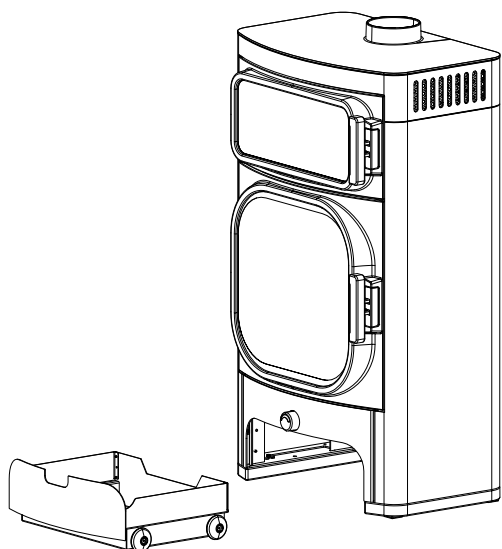
Abb. 30: Holzlade einsetzen
