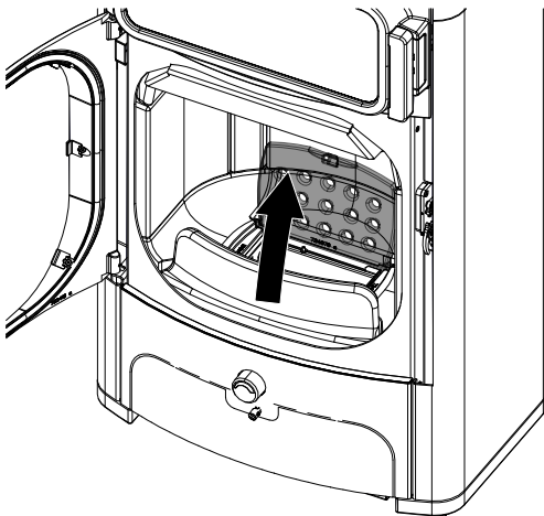
Abb. 51: Rost hochklappen
