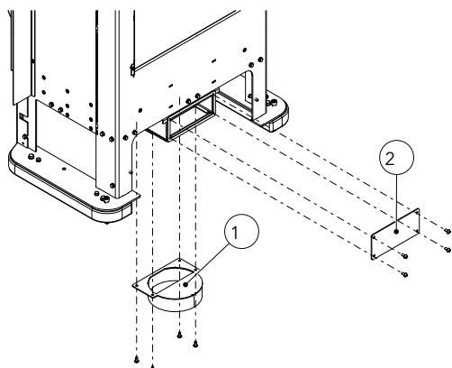
Abb. 28: Zuluftflansch abmontieren
