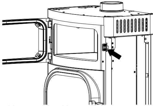
Abb. 43: Türverschluss einstellen
