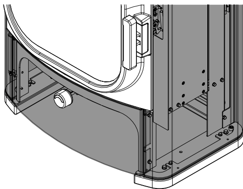
Abb. 33: Seitenverkleidung montieren
