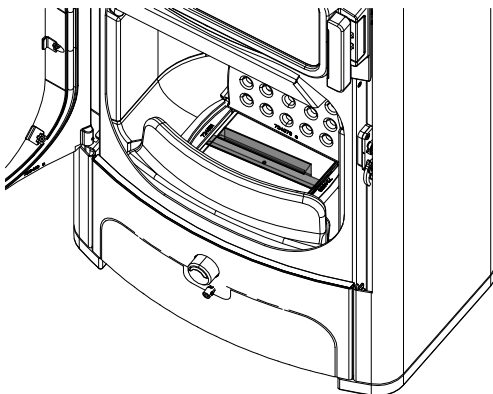
Abb. 53: Deckel zumachen
