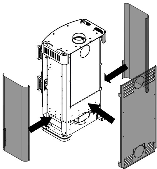
Abb. 18: Rückwand und Seitenverkleidung montieren
