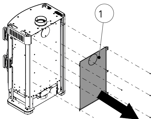
Abb. 20: Strahlungsschutz demontieren
