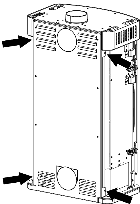
Abb. 58: Schrauben links und rechts von der Rückwand lösen
