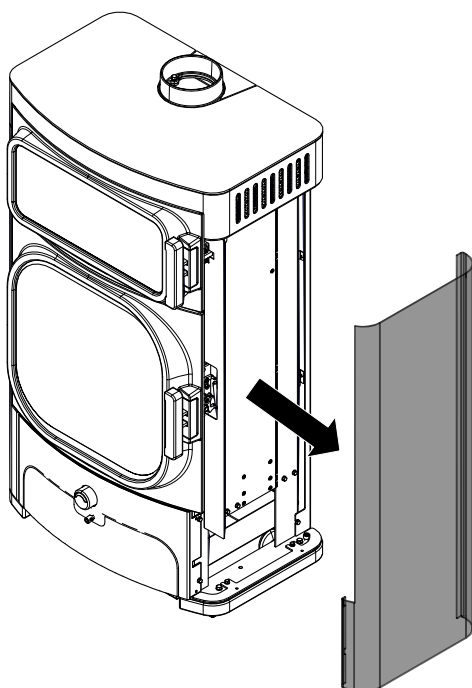
Abb. 57: Seitenverkleidung abnehmen
