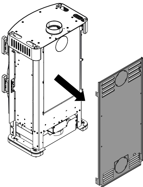
Abb. 59: Rückwand abnehmen
