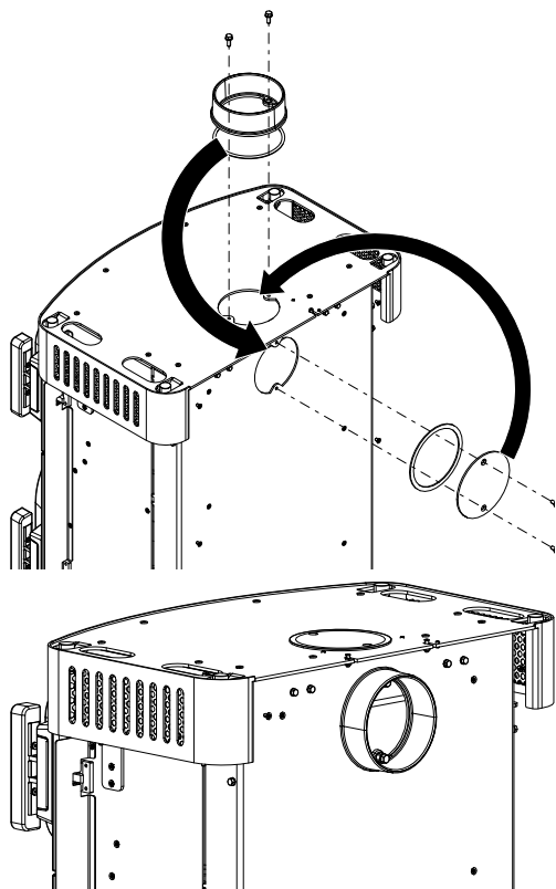
Abb. 13: Abdeckung und Stützen tausche
