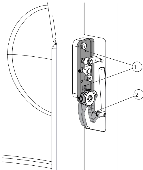
Abb. 41: Türverschluss einstellen
