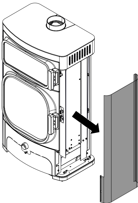
Abb. 53: Seitenverkleidung abnehmen
