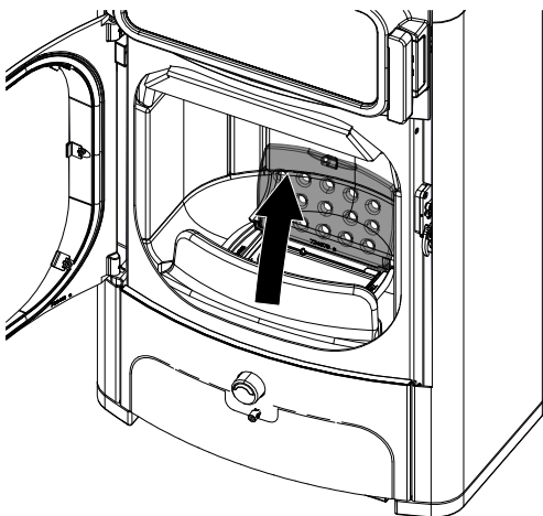
Abb. 47: Rost hochklappen
