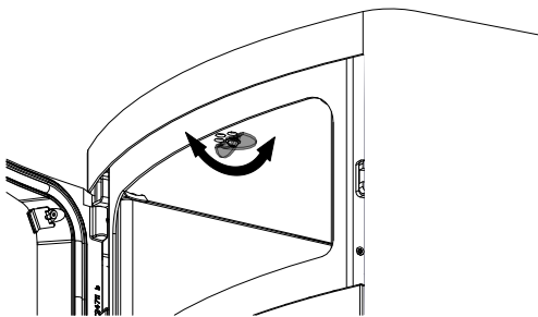
Abb. 43: Lüftregler
