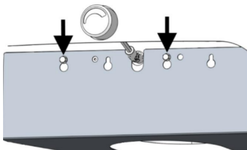
Abb. 37: Abdeckung montieren
