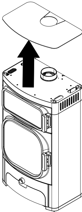
Abb. 11: Kochfeld abnehmen
