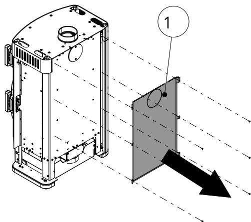
Abb. 19: Strahlungsschutz montieren
