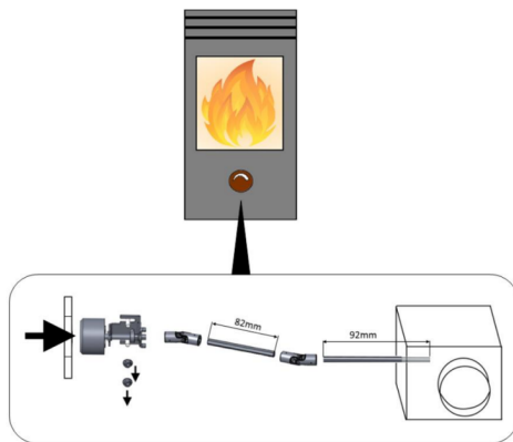
Abb. 33: Drehreglereinheit ausbauen
