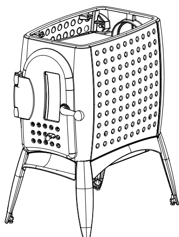
Fig. 26: Rimozione del coperchio
