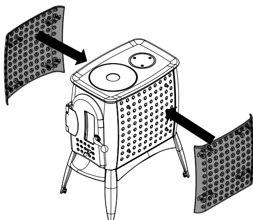
Fig. 18: Installazione del cappotto KV
