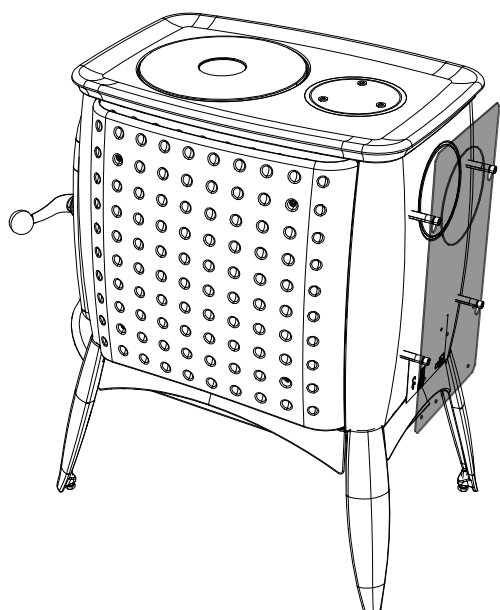
Fig. 16: Montaggio della protezione anti-irradiazione posteriore
