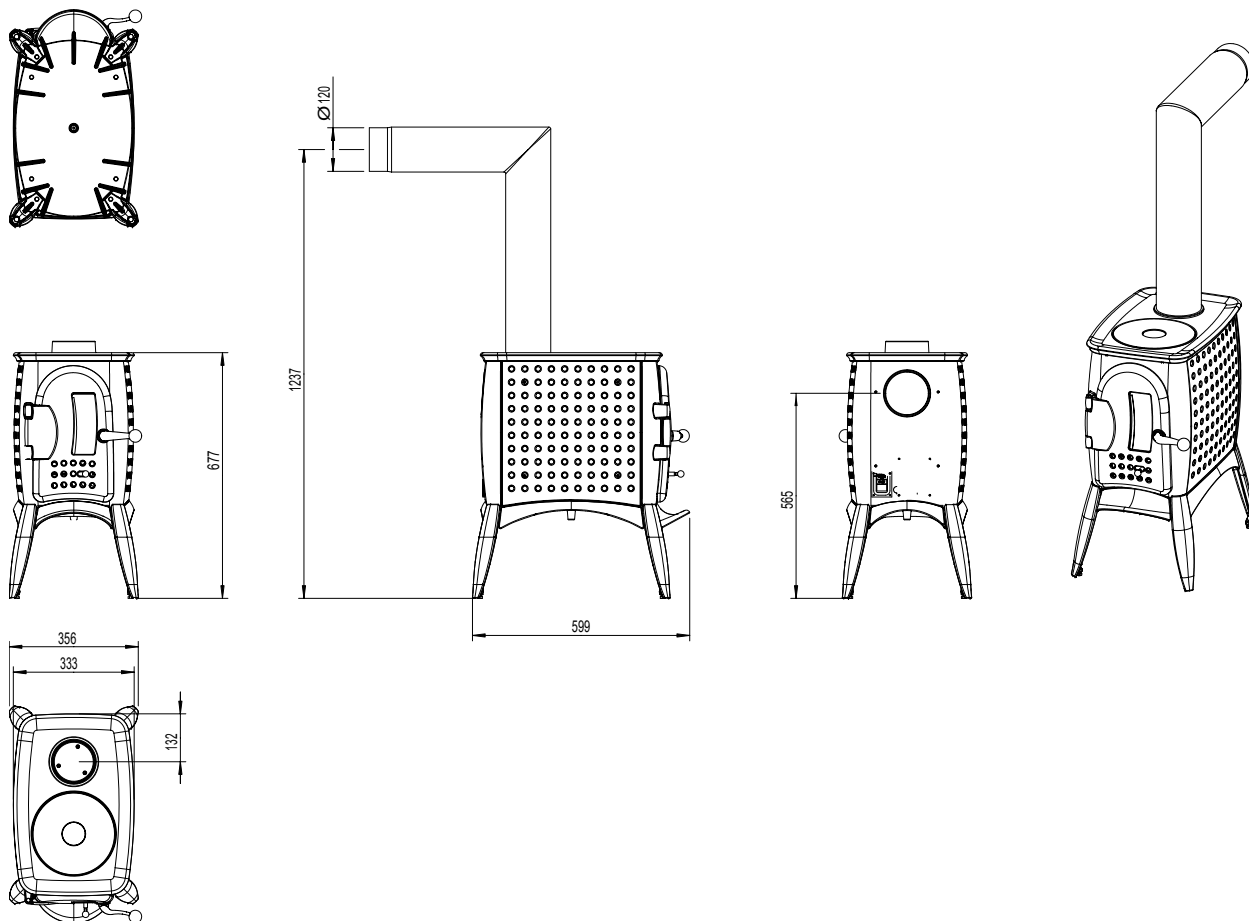
Fig. 1: Dimensioni G1
