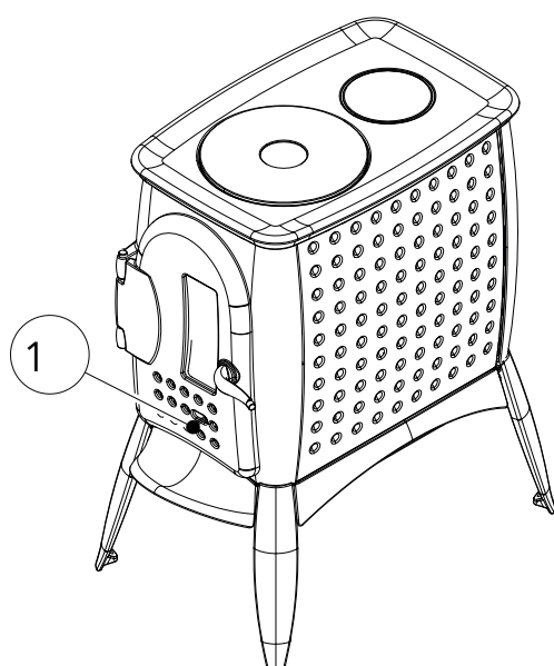
Fig. 20: Serranda dell'aria
