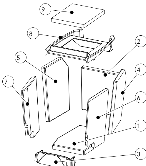
Fig. 19: Installazione del Keramott
