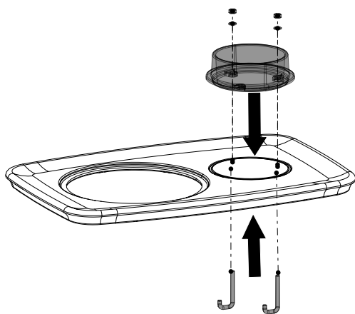
Fig. 9: Montaggio della presa della canna fumaria sul coperchio
