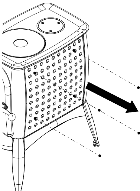
Fig. 17: Svitamento delle viti a perno
