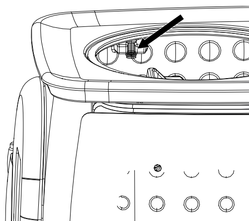
Fig. 6: Rimozione della vite di tenuta
