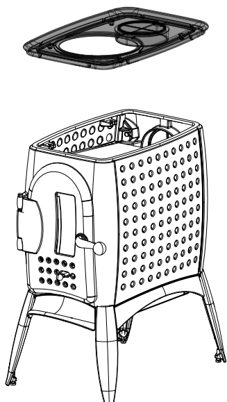
Fig. 7: Rimozione del coperchio
