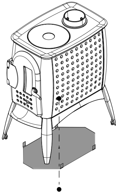
Fig. 13: Montaggio della protezione anti-irradiazione in basso
