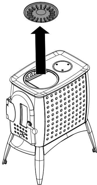
Abb. 6: Kochplatte abnehmen
