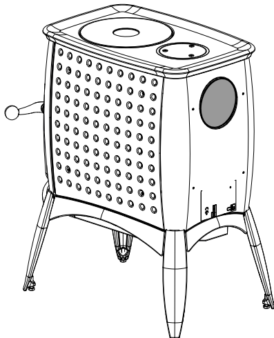
Abb. 12: Stelle einschlagen
