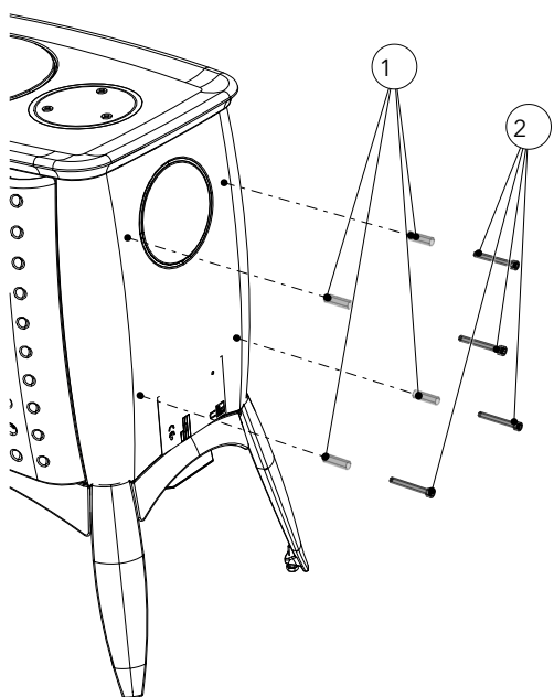
Abb. 16: Distanzen über Schrauben
