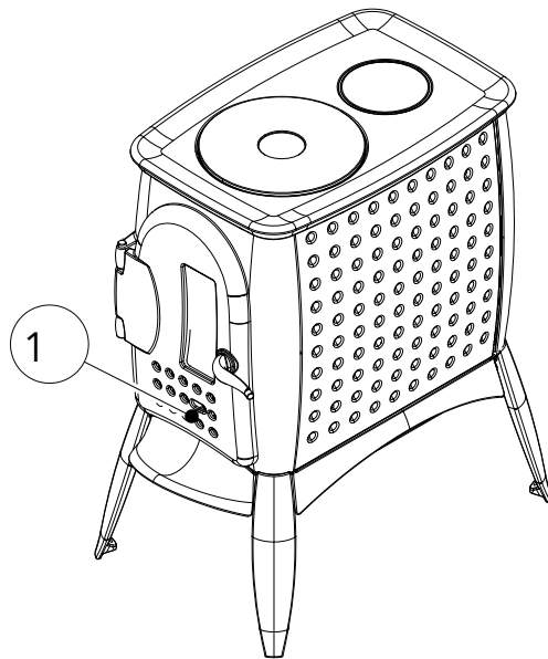
Abb. 3: Luftschieber
