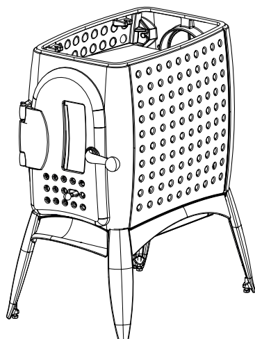
Abb. 28: Umlenkplatte entfernen
