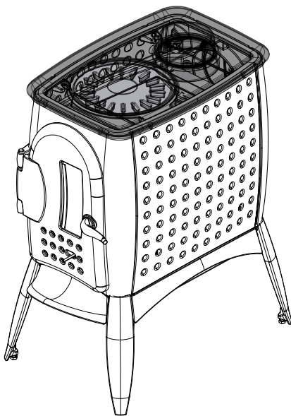
Abb. 11: Deckel und Kochplatte anbringen
