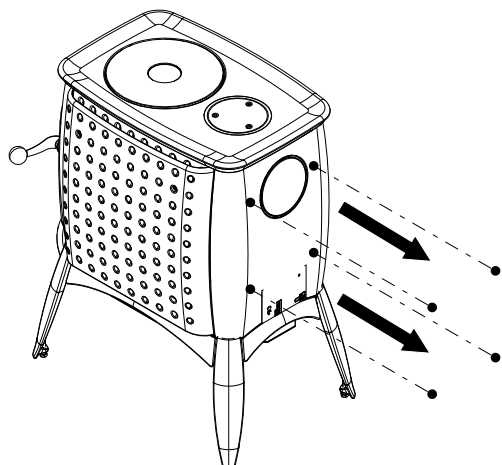
Abb. 15: Stiftschrauben heraus-schrauben
