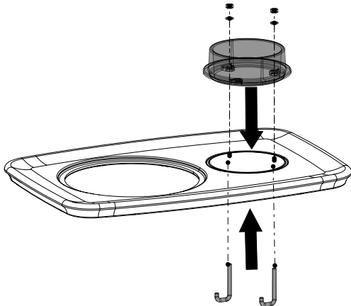
Abb. 10: Rauchrohrstutzen auf dem Deckel montieren
