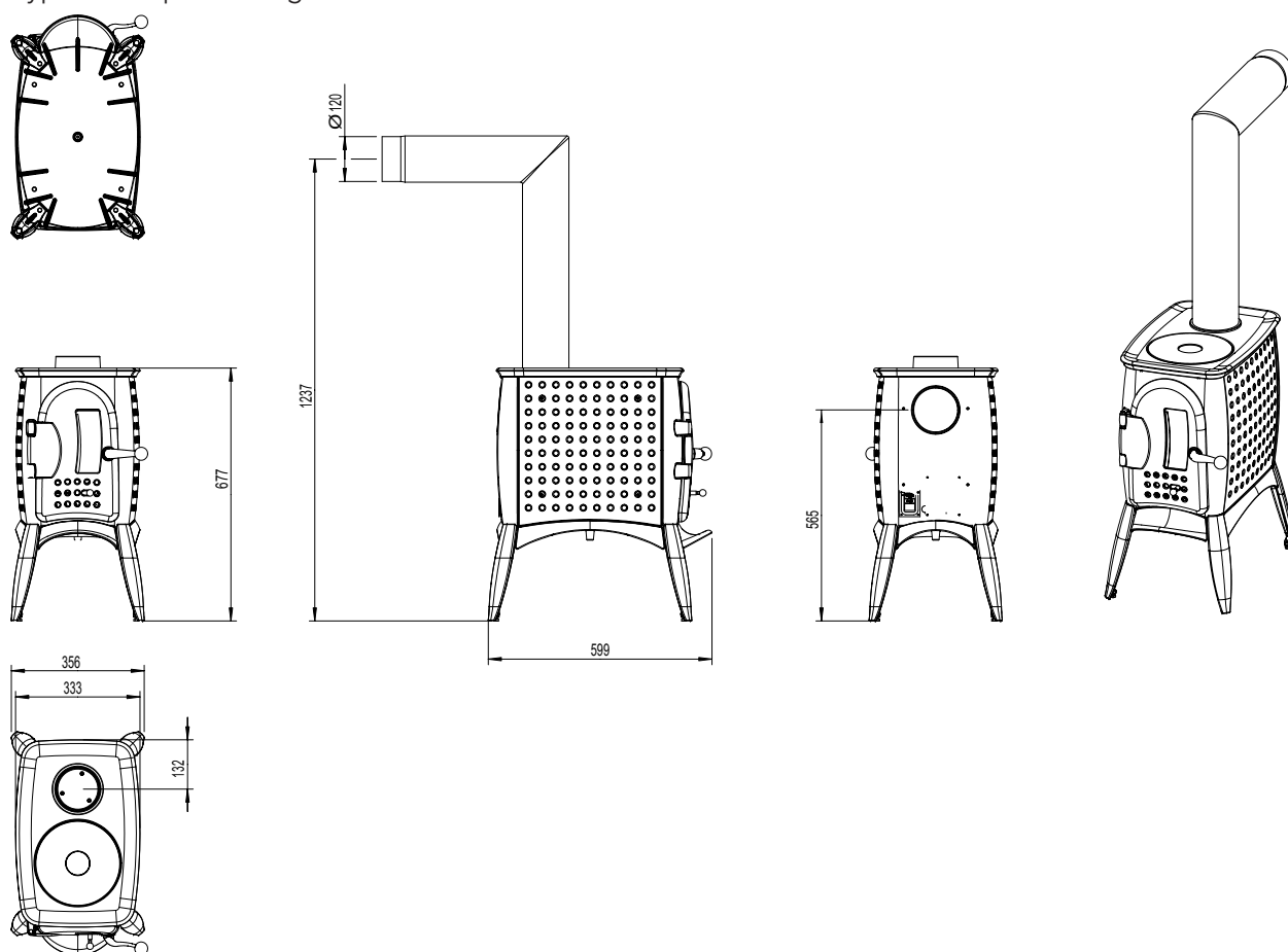
Abb. 2: Abmessungen G1
