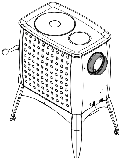
Abb. 13: Rauchrohrstutzen hinten montieren
