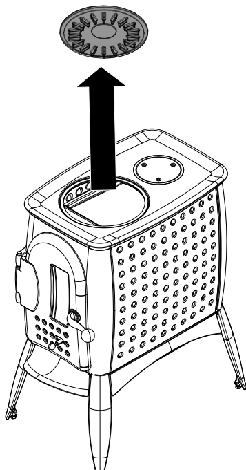
Abb. 24: Kochplatte abnehmen
