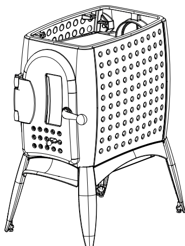
Abb. 27: Deckel abnehmen
