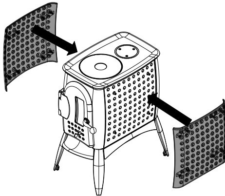
Abb. 19: KV-Mantel montieren
