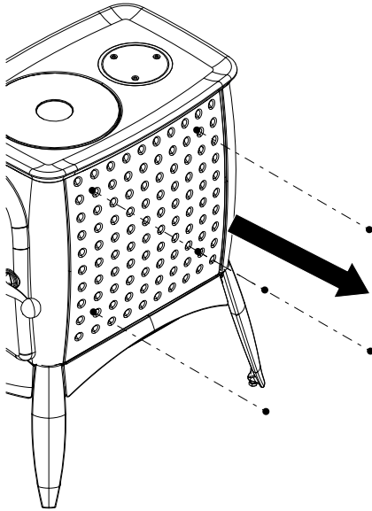
Abb. 18: Stiftschrauben heraus-schrauben
