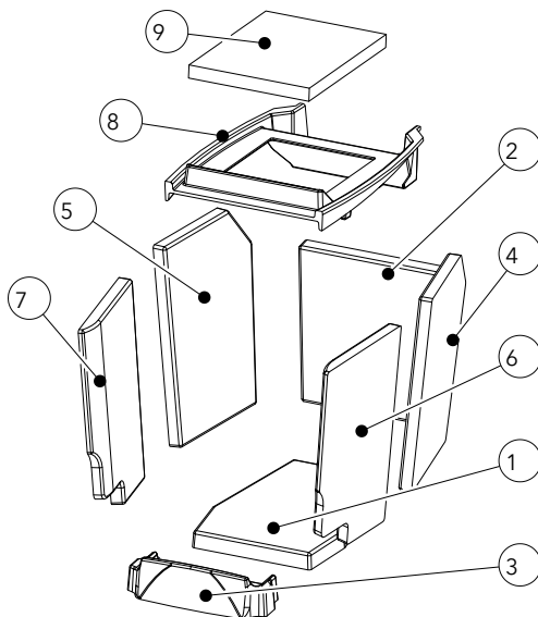
Abb. 20: Keramott einbauen
