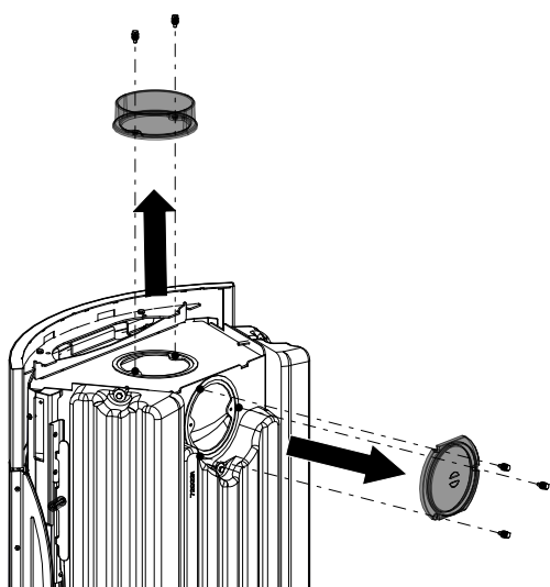
Fig. 8: Démonter le recouvrement et la tubulure de fumées
