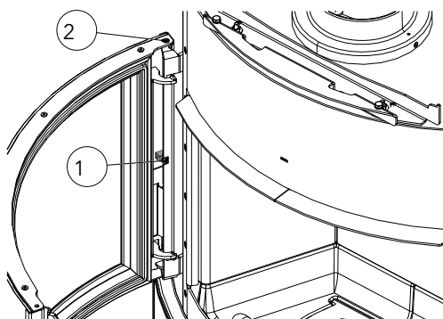
Fig. 34: Tendre ou détendre le ressort
