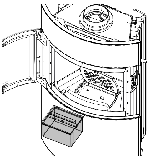
Fig. 40: Enlever et vider le bac à cendres
