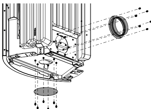
Fig. 18: Démonter le recouvrement et la tubulure de fumées
