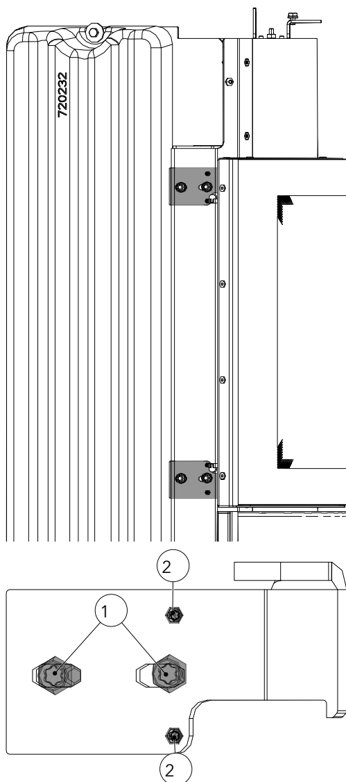
Fig. 28: Régler la porte
