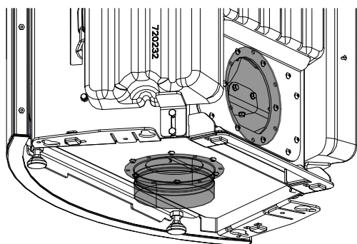
Fig. 15: Pièces interchangeables
