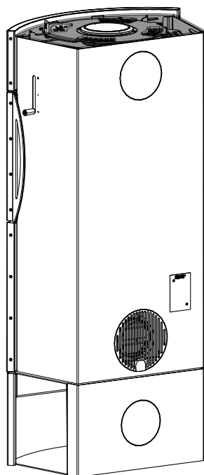
Fig. 26: Installer l'habillage latéral
