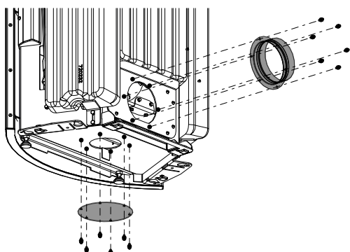
Fig. 23: Démonter le recouvrement et la tubulure de fumées
