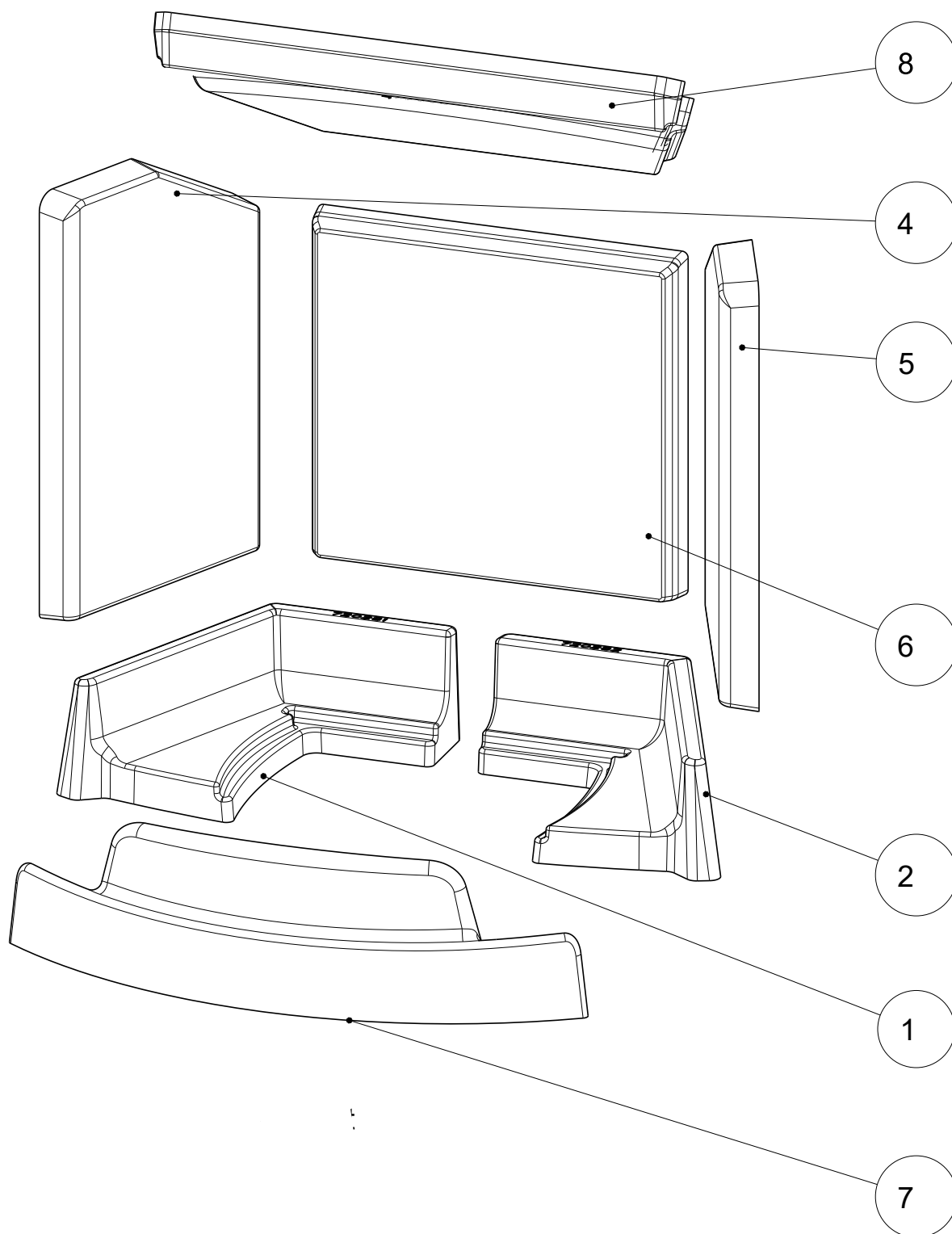
Fig. 27: Installer la Keramott
