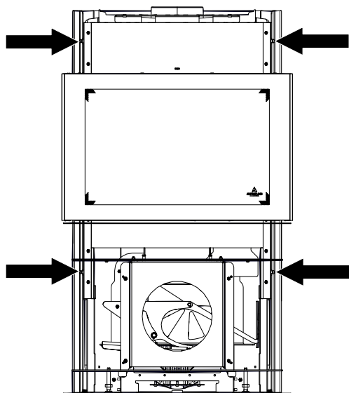
Fig. 44: Dévisser les vis
