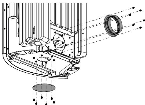
Fig. 14: Démontez le recouvrement et la tubulure de fumées
