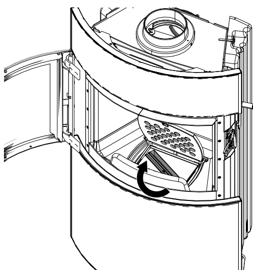
Fig. 39: Mettre le couvercle sur le bac à cendres et l'enclencher
