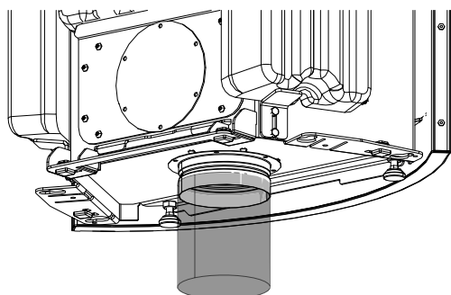
Fig. 16: Fixer le conduit
