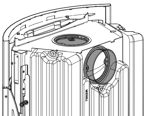
Fig. 10: Recouvrement et tubulure de fumées échangés
