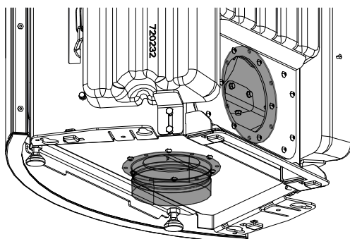
Fig. 19: Pièces interchangeables
