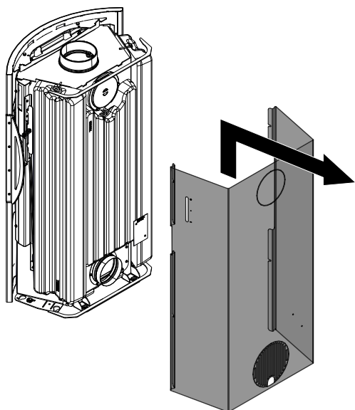
Fig. 45: Enlever l'habillage latéral
