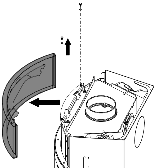
Fig. 42: Enlever le parement supérieur
