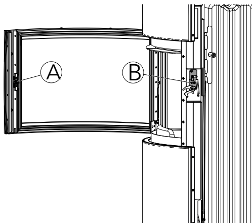
Fig. 30: Régler la serrure de la porte
