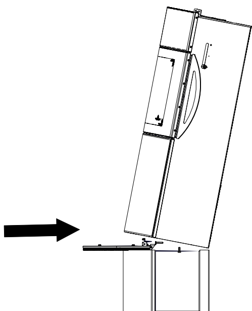
Fig. 42: Poser le poêle à bois sur le socle
