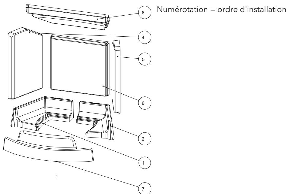
Fig. 49: Installer la Keramott
