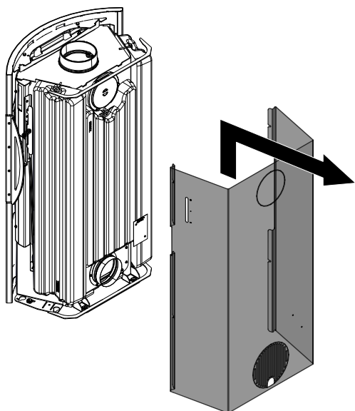
Fig. 71: Enlever l'habillage latéral
