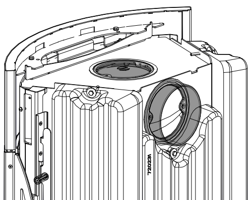
Fig. 10: Recouvrement et tubulure échangés
