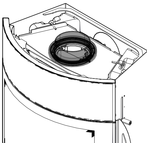
Fig. 44: Installer la tubulure de fumées orientable
