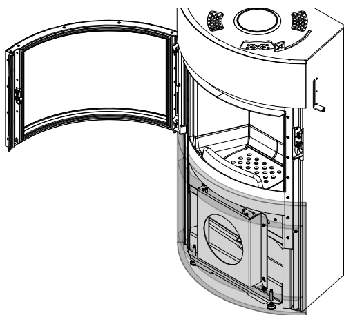
Fig. 31: Poser le parement inférieur
