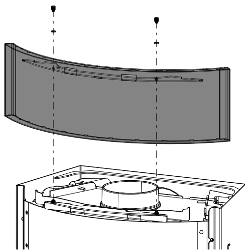
Fig. 29: Poser et fixer le parement
