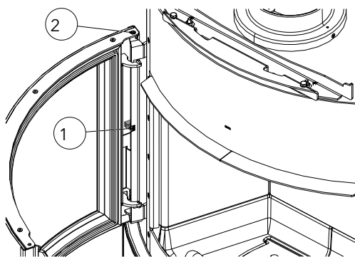
Fig. 59: Tendre ou détendre le ressort
