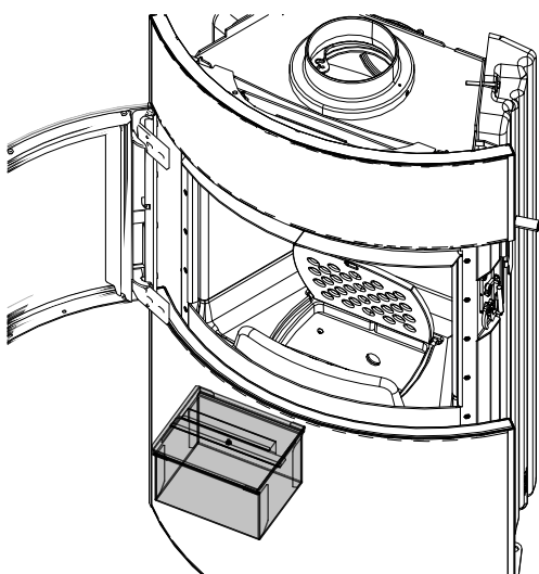
Fig. 66: Enlever et vider le bac à cendres
