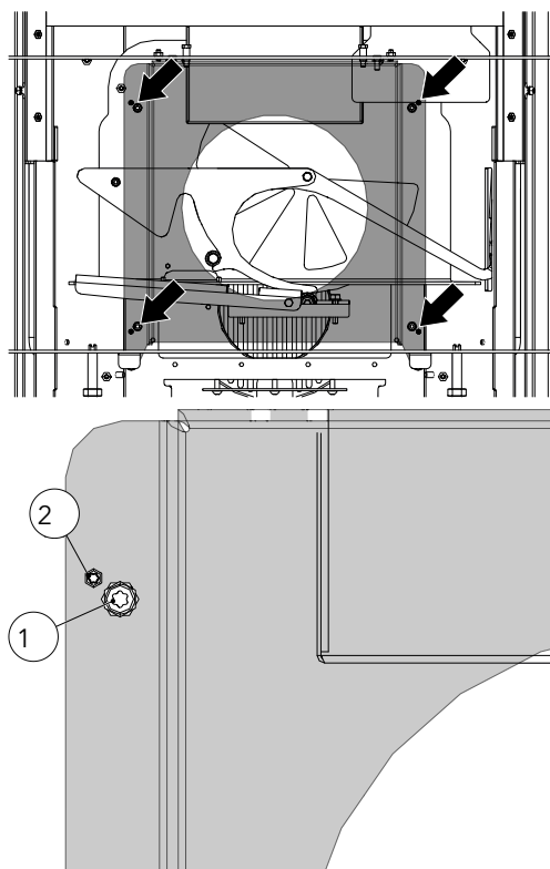
Fig. 51: Ajuster le parement inférieur
