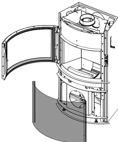
Fig. 69: Ouvrir la porte
