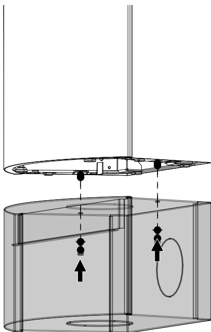
Fig. 48: Fixer le socle par le dessous
