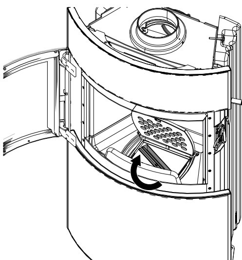
Fig. 65: Mettre le couvercle sur le bac à cendres et l'enclencher
