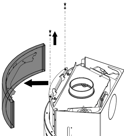
Fig. 68: Enlever le parement supérieur
