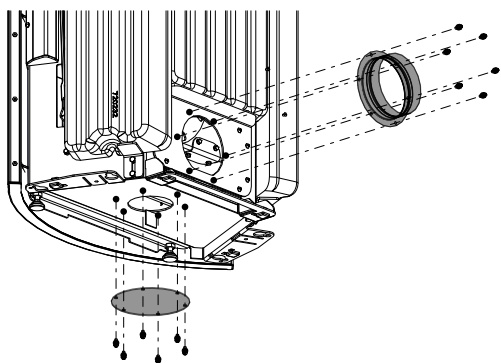
Fig. 14: Enlever la tubulure et le recouvrement
