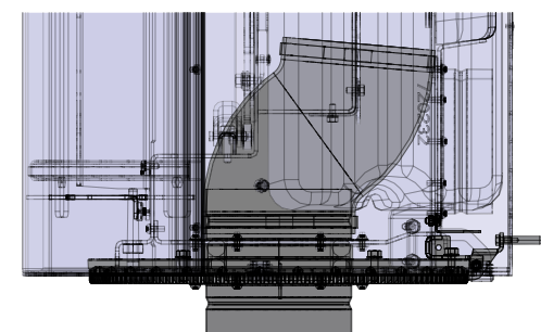
Fig. 40: Fixer le plateau tournant au poêle à bois
