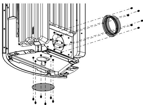
Fig. 18: Enlever la tubulure et le recouvrement
