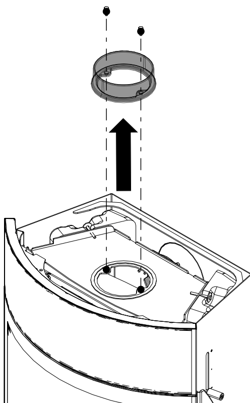
Fig. 43: Démontez la tubulure de fumées
