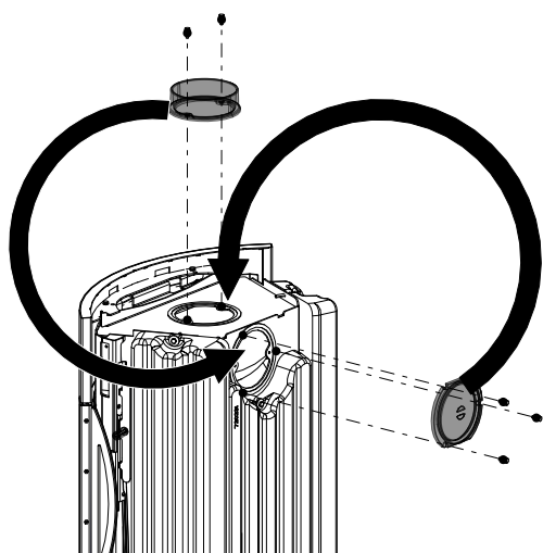
Fig. 9: Échanger le recouvrement et la tubulure
