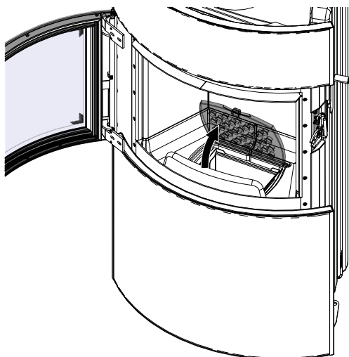
Fig. 64: Relever la grille
