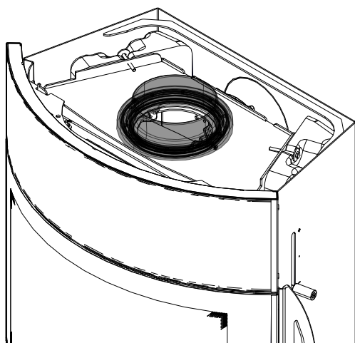
Fig. 38: Installer la tubulure de fumées orientable
