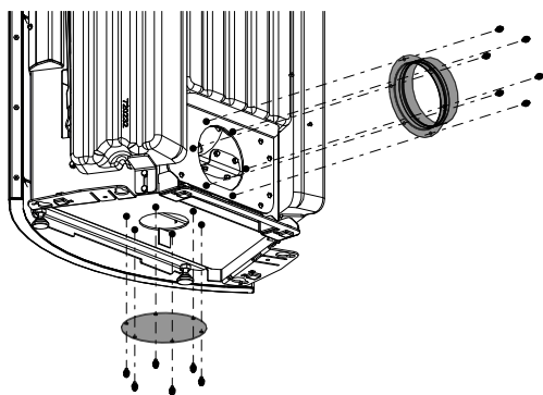
Fig. 23: Enlever la tubulure et le recouvrement
