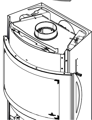
Fig. 27: Enlever le couvercle
