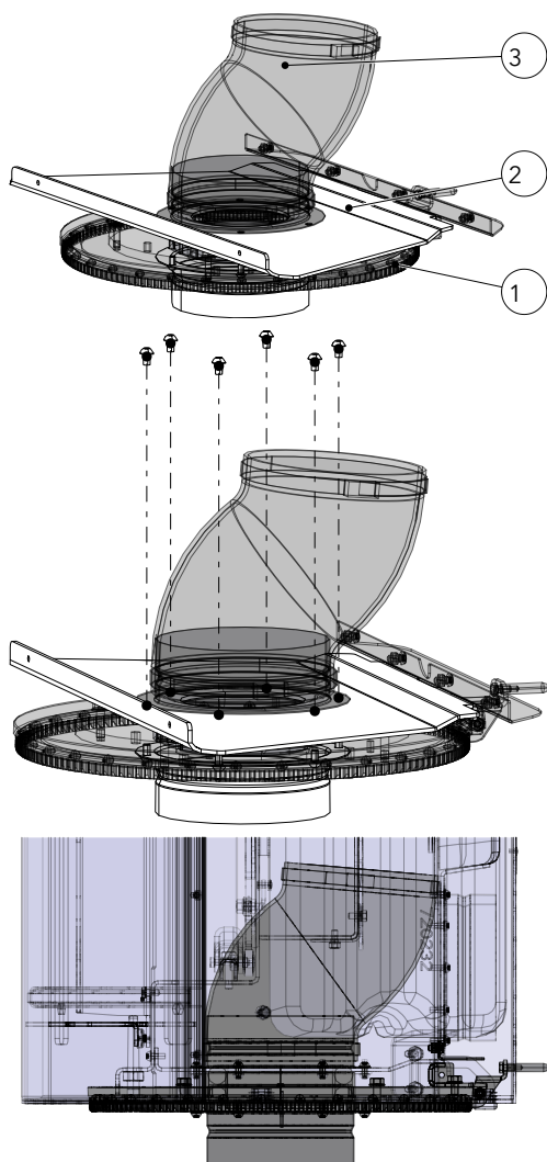
Fig. 46: Fixer le plateau tournant au poêle à bois
