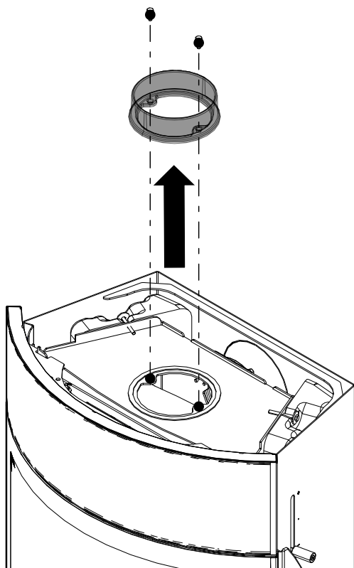
Fig. 37: Démonter la tubulure de fumées
