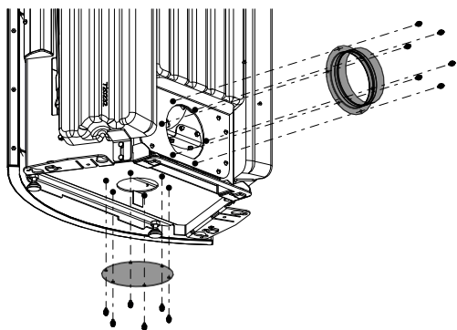
Fig. 23: Smontaggio del coperchio e della presa della canna fumaria
