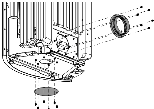
Fig. 14: Smontaggio del coperchio e della presa della canna fumaria
