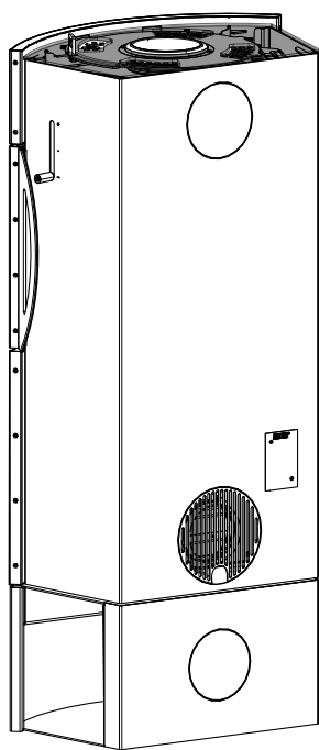
Fig. 26: Montaggio del rivestimento laterale
