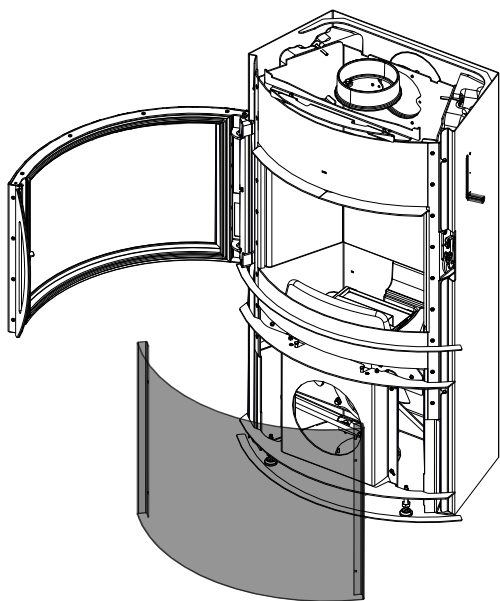
Fig. 43: Apertura dello sportello
