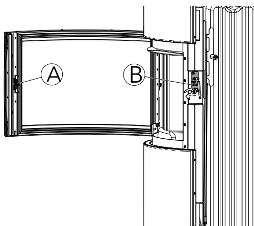
Fig. 30: Regolazione della serratura dello sportello
