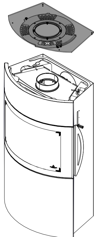
Fig. 41: Rimozione del coperchio
