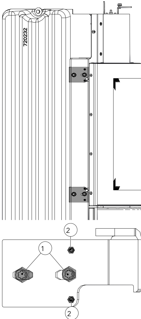
Fig. 28: Regolazione dello sportello
