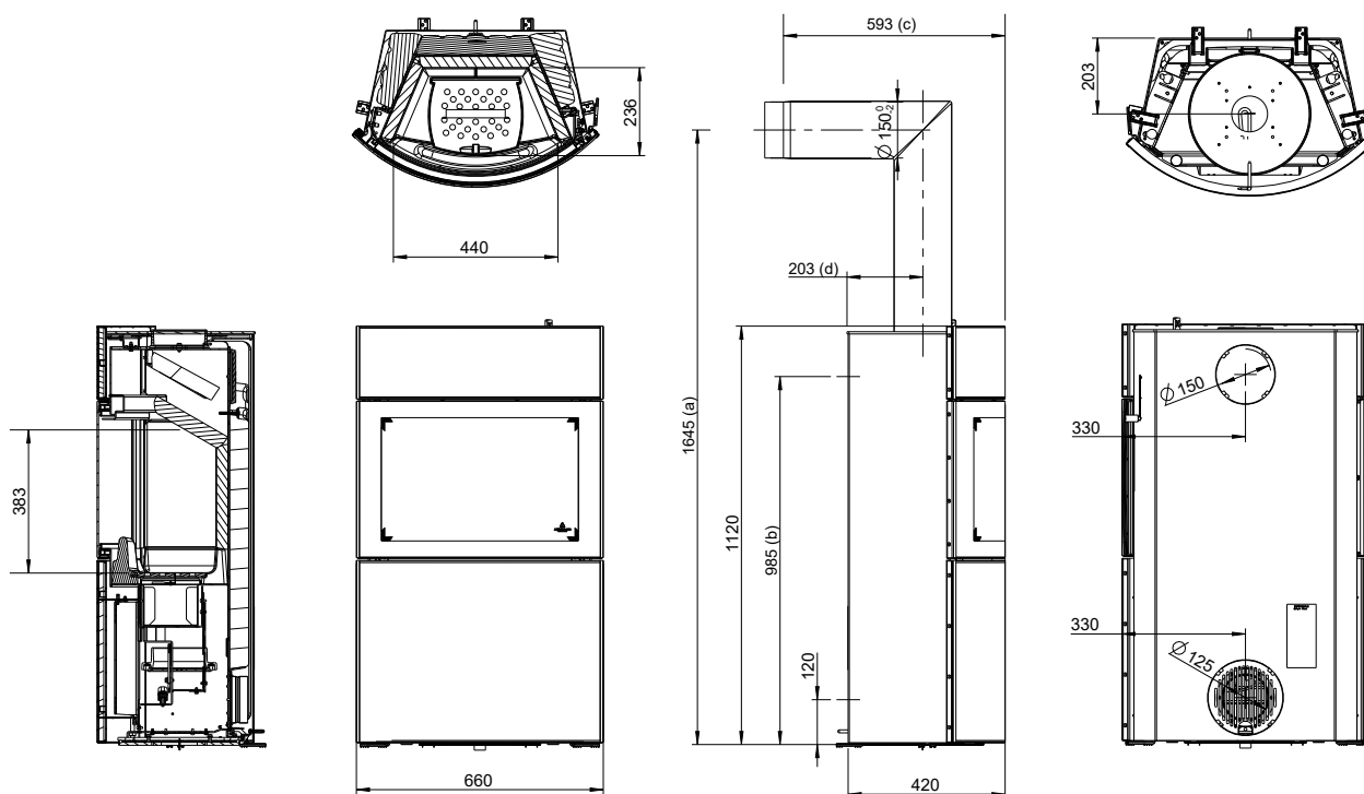
Fig. 1: Dimensioni Fynn Xtra
