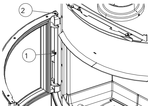
Fig. 34: Tensionamento e detensionamento della molla
