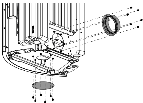
Fig. 18: Smontaggio del coperchio e della presa della canna fumaria
