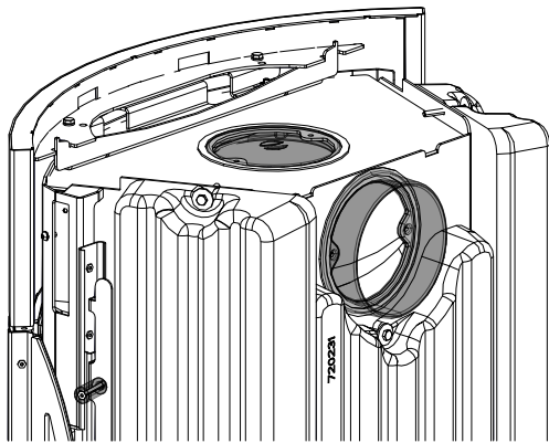
Fig. 10: Coperchio e la presa della canna fumaria scambiati
