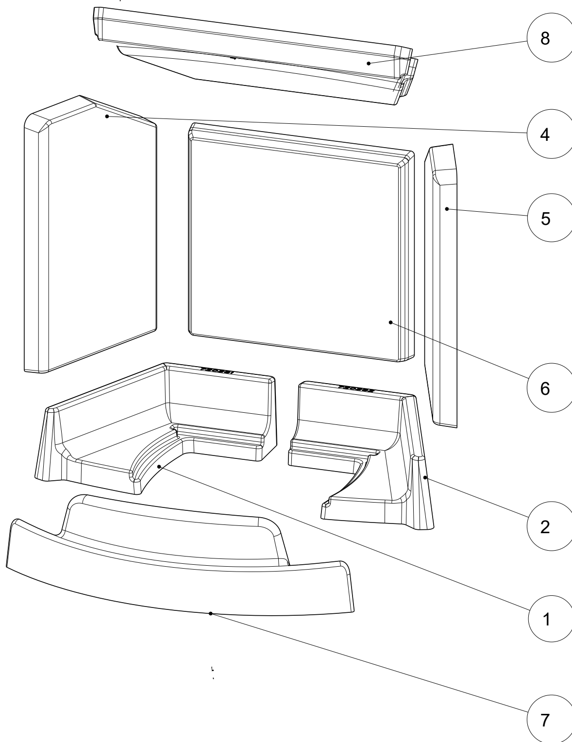
Fig. 27: Installazione del Keramott
