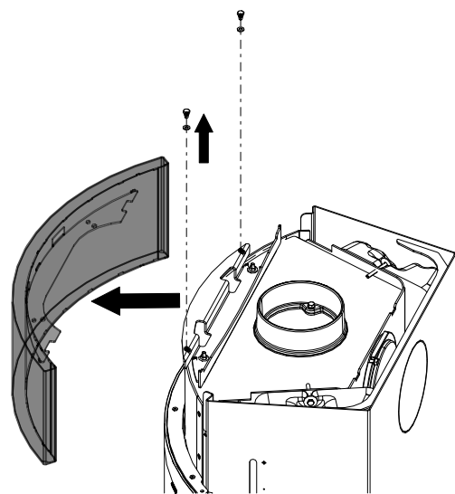
Fig. 42: Rimozione del diaframma superiore
