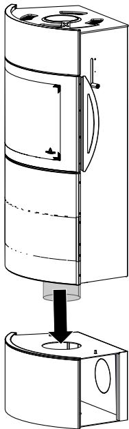
Fig. 20: Posizionamento della stufa sulla base
