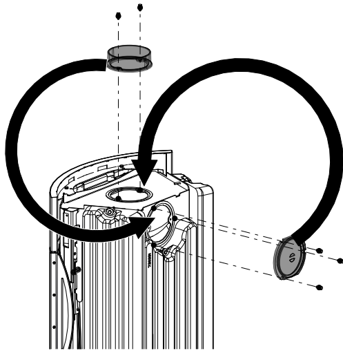
Fig. 9: Sostituire il coperchio e della presa la canna fumaria
