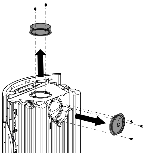
Fig. 8: Smontaggio del coperchio e della presa della canna fumaria
