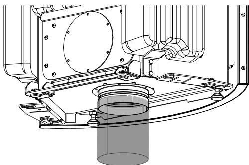
Fig. 16: Fissaggio del tubo
