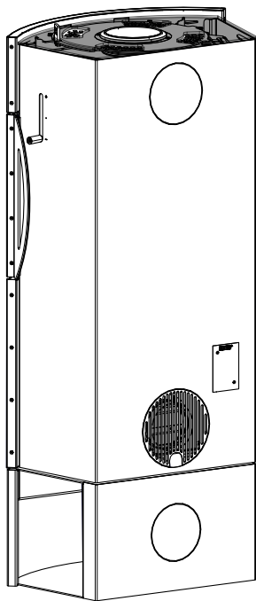
Fig. 21: Montaggio del rivestimento laterale
