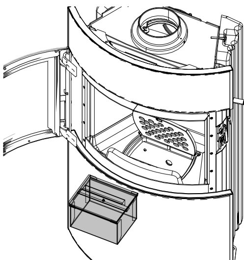
Fig. 40: Rimozione e svuotamento del box cenere
