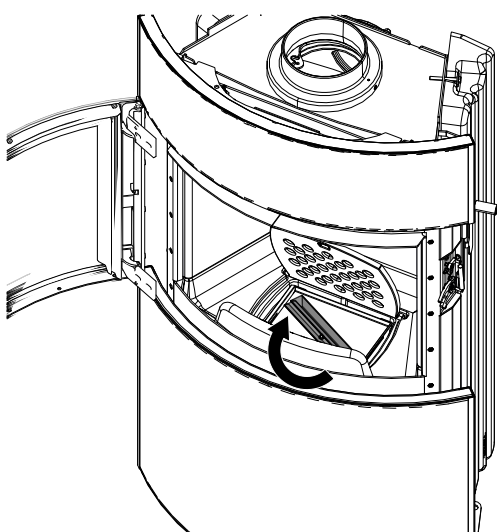
Fig. 39: Collocazione e aggancio a scatto del coperchio sul box cenere
