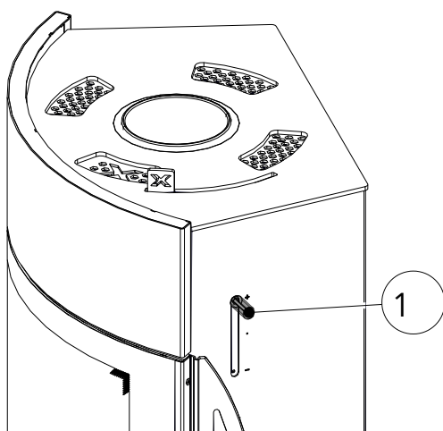
Fig. 35: Regolatore dell'aria primaria/secondaria
