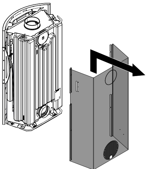
Fig. 45: Rimozione del rivestimento laterale
