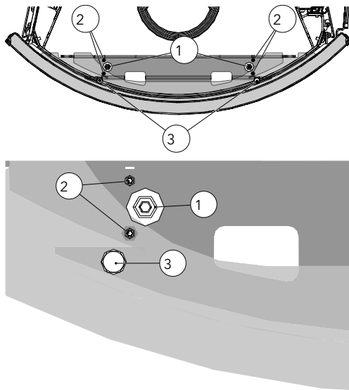
Fig. 50: Regolazione del diaframma in alto
