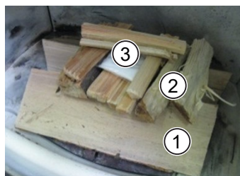
Fig. 62: Prima dell'accensione
