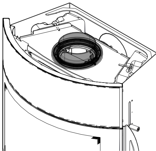
Fig. 38: Montaggio della presa della canna fumaria rotante
