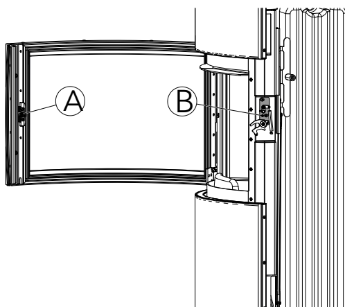
Fig. 55: Regolazione della serratura dello sportello
