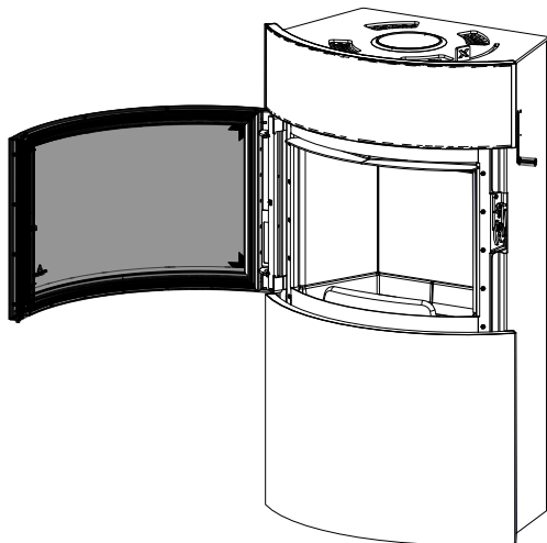
Fig. 54: Apertura dello sportello
