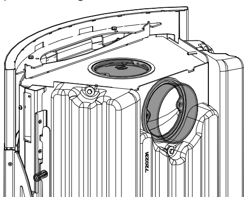
Fig. 10: Copertura e pezzo di collegamento sostituiti
