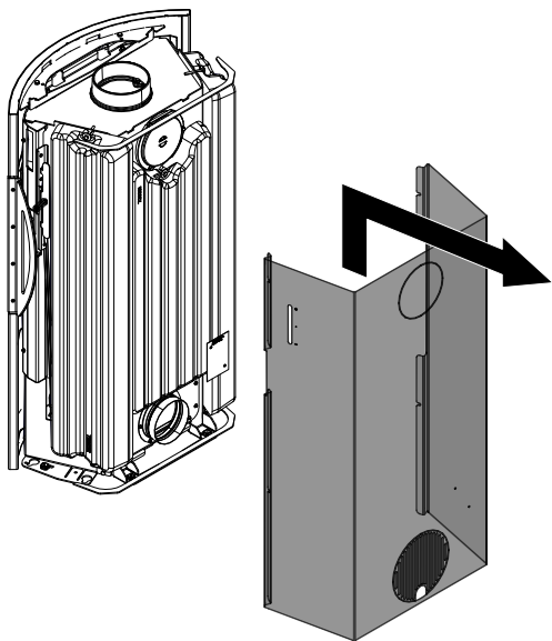
Fig. 71: Rimozione del rivestimento laterale
