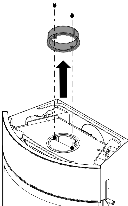
Fig. 33: Smontaggio della presa della canna fumaria
