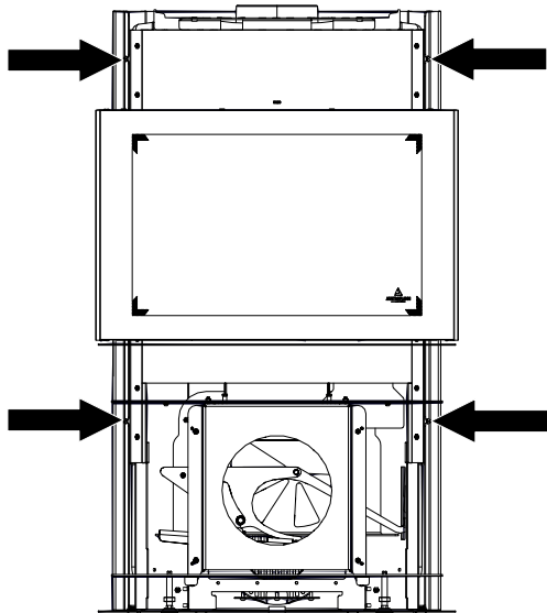
Fig. 70: Svitamento delle viti
