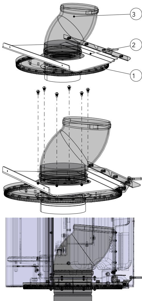
Fig. 46: Fissaggio del disco girevole alla stufa a caminetto
