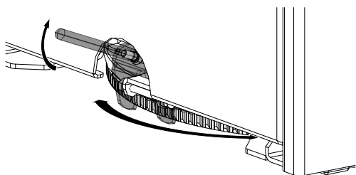
Fig. 60: Regolazione del piatto girevole
