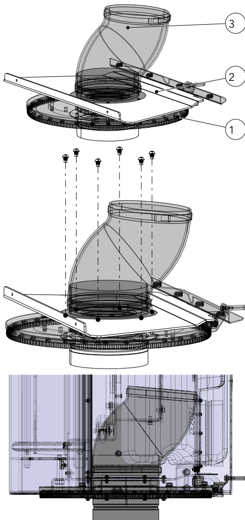
Fig. 40: Fissaggio del disco girevole alla stufa a caminetto
