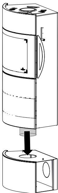
Fig. 20: Posizionamento della stufa sulla base
