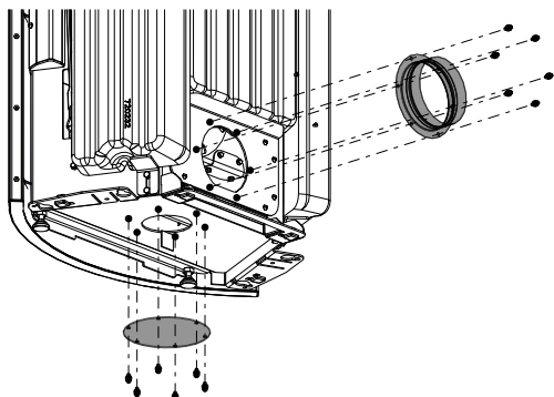
Fig. 14: Rimozione dell'elemento di collegamento e del coperchio
