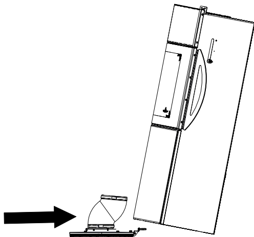
Fig. 39: Inclinamento della stufa
