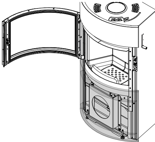
Fig. 31: Inserimento del diaframma in basso
