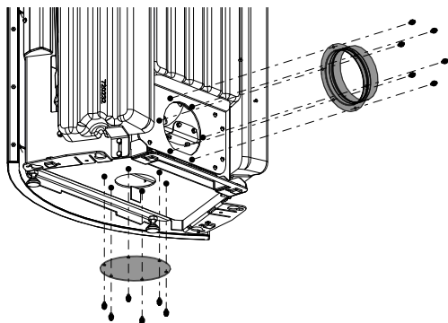
Fig. 23: Rimozione dell'elemento di collegamento e del coperchio
