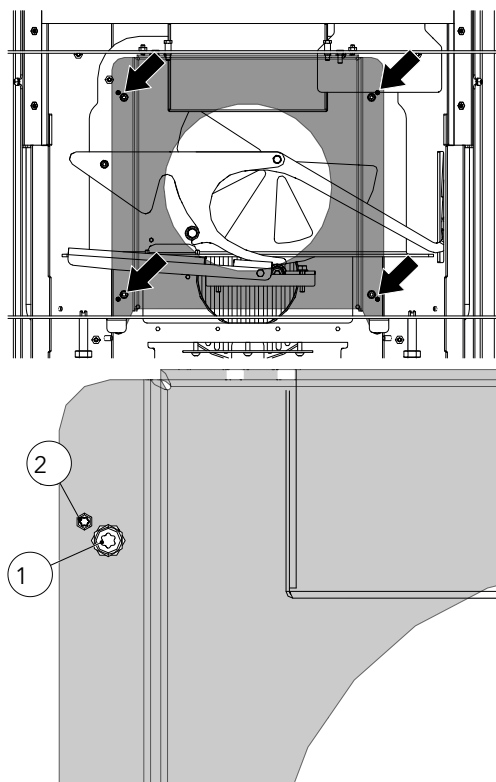
Fig. 51: Regolazione del diaframma in basso
