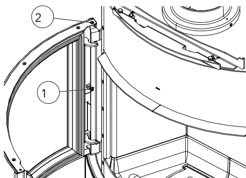
Fig. 59: Tensionamento e detensionamento della molla
