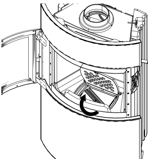
Fig. 65: Collocazione e aggancio a scatto del coperchio sul box cenere
