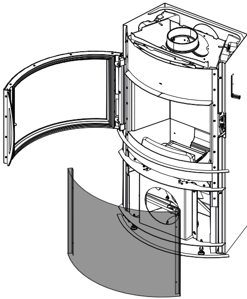
Fig. 69: Apertura dello sportello
