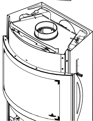
Fig. 27: Rimozione del coperchio
