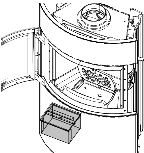
Fig. 66: Rimozione e svuotamento del box cenere
