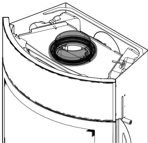
Fig. 44: Montaggio della presa della canna fumaria rotante
