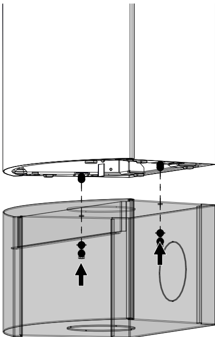
Fig. 48: Montaggio della base da dietro
