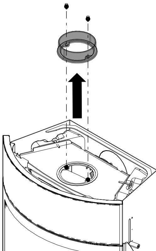
Fig. 37: Smontaggio della presa della canna fumaria
