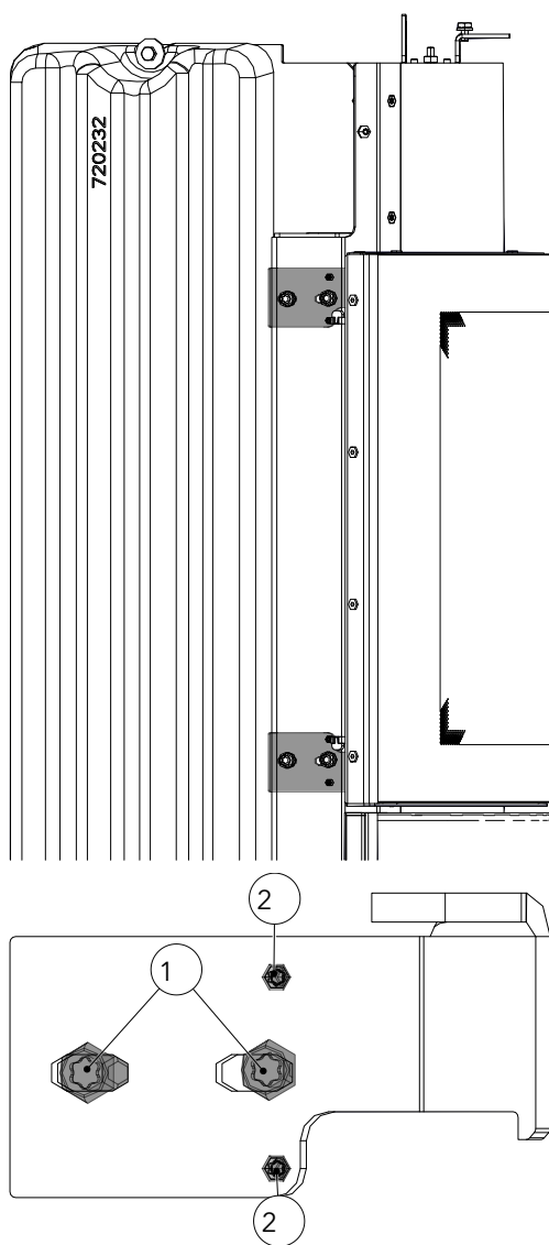
Fig. 53: Regolazione dello sportello
