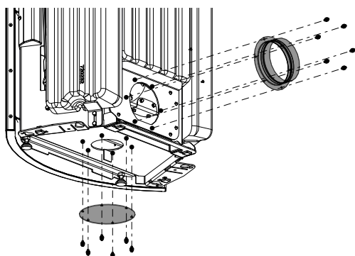
Fig. 18: Rimozione dell'elemento di collegamento e del coperchio
