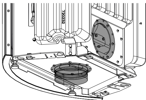
Fig. 24: Pezzi sostituiti
