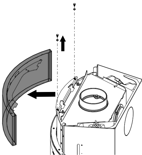
Fig. 68: Rimozione del diaframma superiore
