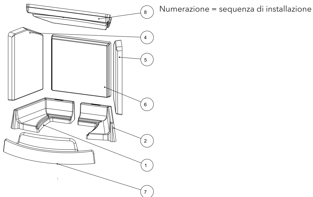
Fig. 49: Installazione del Keramott
