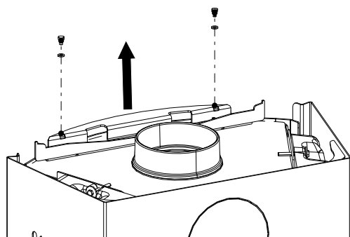
Fig. 28: Svitamento delle viti
