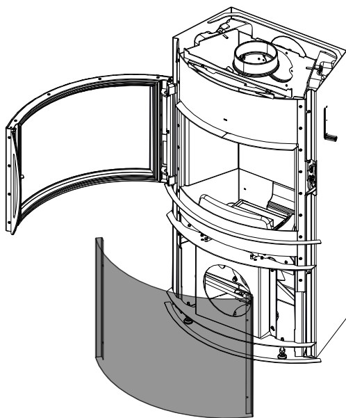
Abb. 44: Tür öffnen
