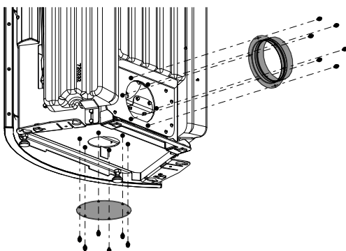
Abb. 19: Abdeckung und Rauchrohrstutzen demontieren
