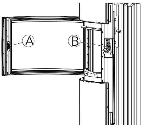
Abb. 31: Türverschluss einstellen
