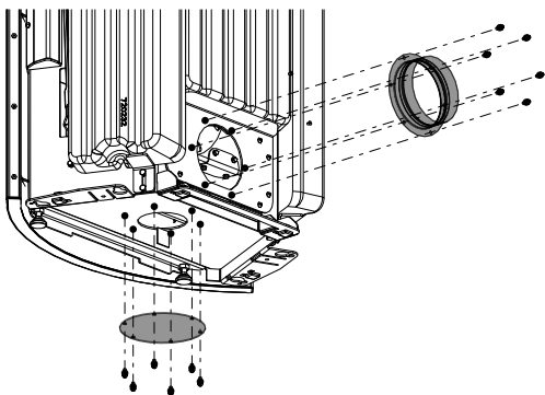
Abb. 24: Abdeckung und Rauchrohrstutzen demontieren
