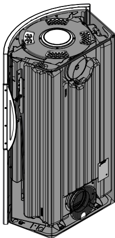
Abb. 14: Seitenverkleidung montieren
