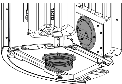
Abb. 25: Teile getauscht
