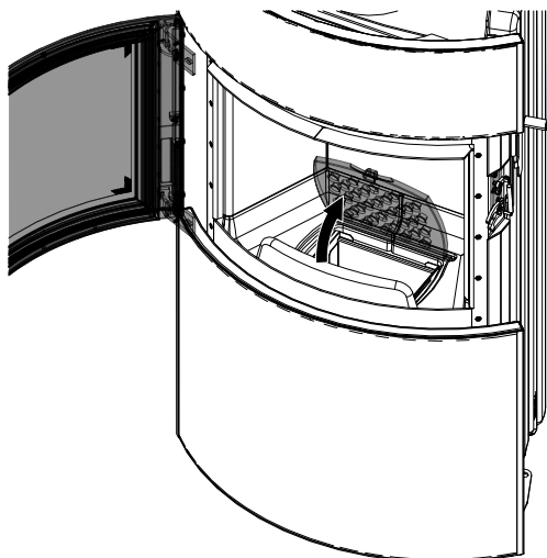
Abb. 39: Rost hochklappen
