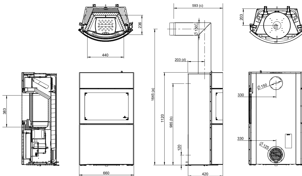
Abb. 2: Abmessungen Fynn Xtra
