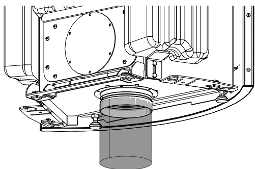
Abb. 17: Rohr befestigen
