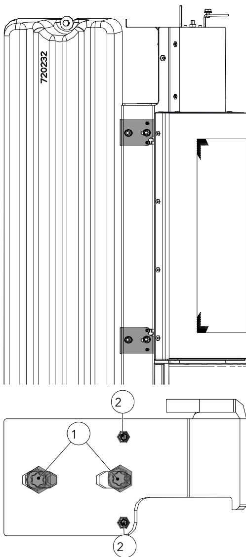
Fig. 52: Regolazione dello sportello
