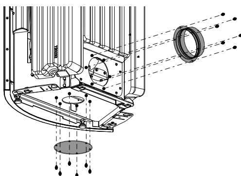
Fig. 17: Rimozione dell'elemento di collegamento e del coperchio
