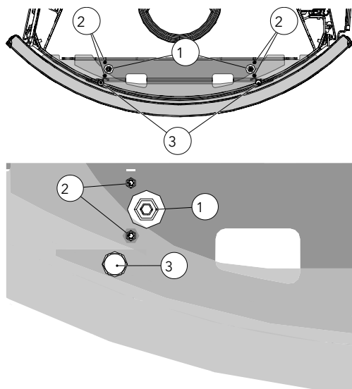
Fig. 49: Regolazione del diaframma in alto
