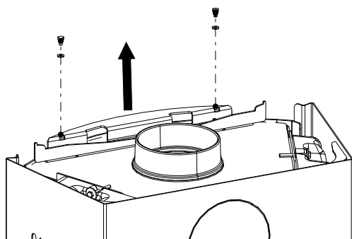
Fig. 27: Svitamento delle viti
