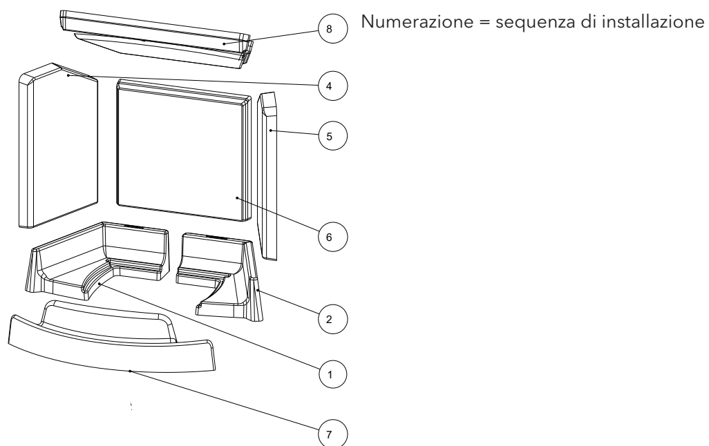
Fig. 48: Installazione del Keramott
