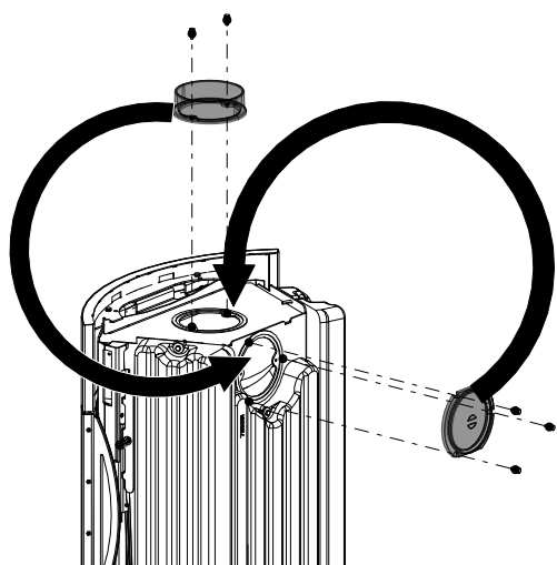
Fig. 8: Sostituzione del coperchio e del pezzo di collegamento
