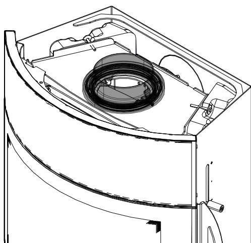
Fig. 43: Montaggio della presa della canna fumaria rotante
