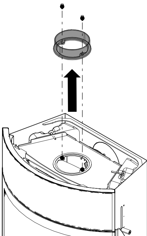
Fig. 32: Smontaggio della presa della canna fumaria
