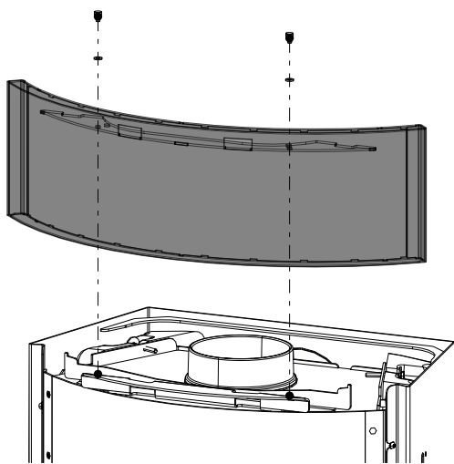
Fig. 28: Collocazione e fissaggio del diaframma
