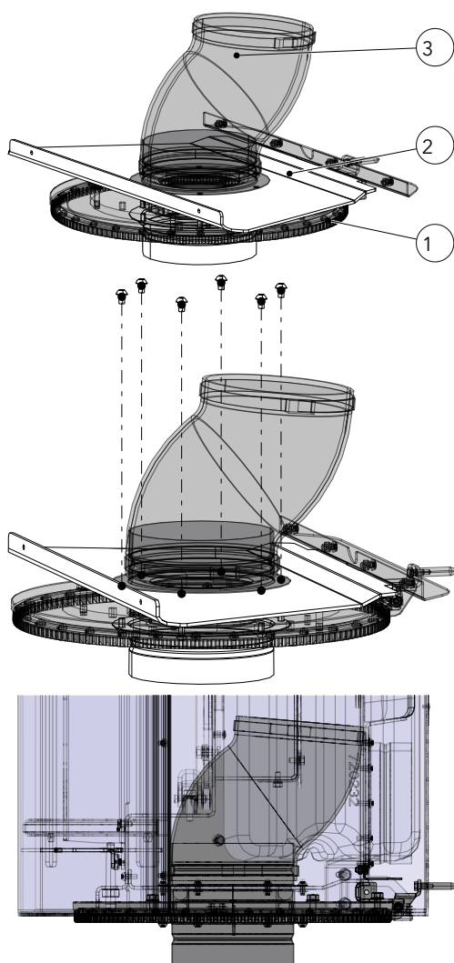
Fig. 39: Fissaggio del disco girevole alla stufa a caminetto
