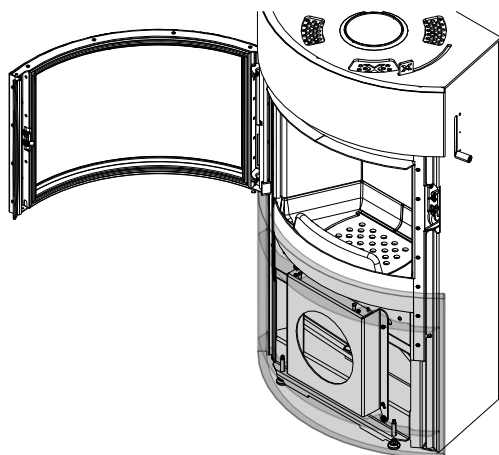
Fig. 30: Inserimento del diaframma in basso
