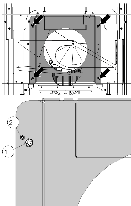
Fig. 50: Regolazione del diaframma in basso
