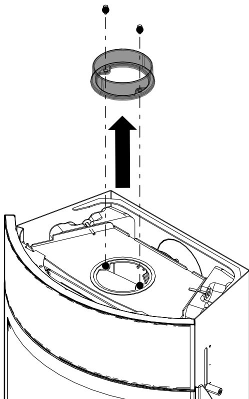
Fig. 42: Smontaggio della presa della canna fumaria
