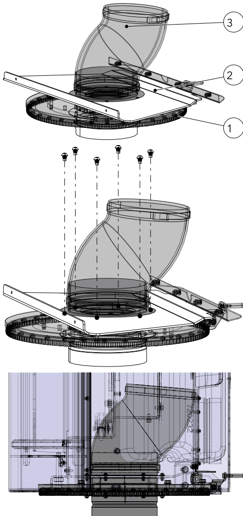
Fig. 45: Fissaggio del disco girevole alla stufa a caminetto
