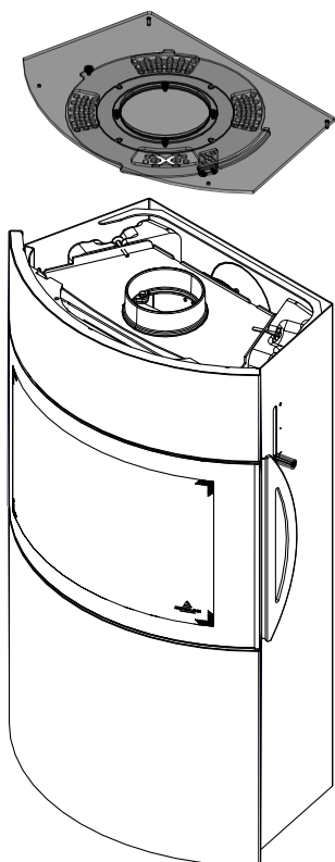
Fig. 31: Rimozione del coperchio
