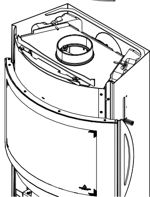
Fig. 26: Rimozione del coperchio
