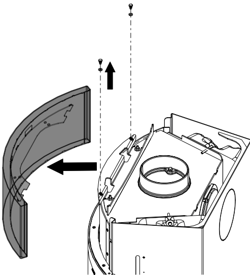
Fig. 67: Rimozione del diaframma superiore
