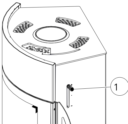
Fig. 60: Regolatore dell'aria primaria/secondaria
