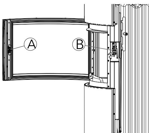
Fig. 54: Regolazione della serratura dello sportello
