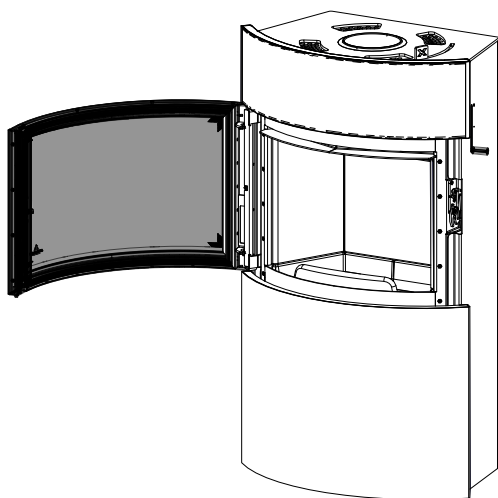
Fig. 57: Apertura dello sportello
