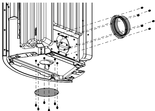
Fig. 13: Rimozione dell'elemento di collegamento e del coperchio
