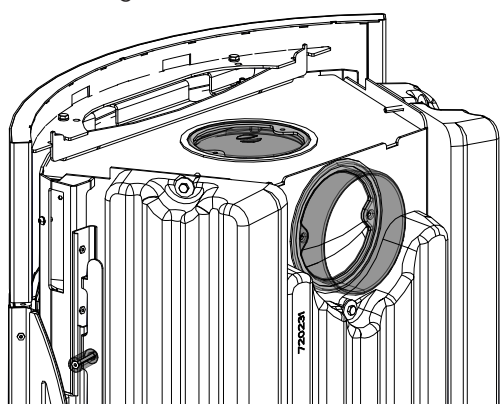
Fig. 9: Coperchio e pezzo di collegamento sostituiti
