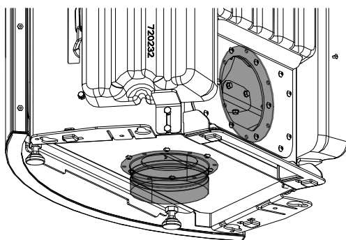
Fig. 18: Pezzi sostituiti
