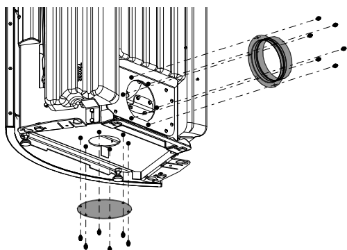
Fig. 22: Rimozione dell'elemento di collegamento e del coperchio
