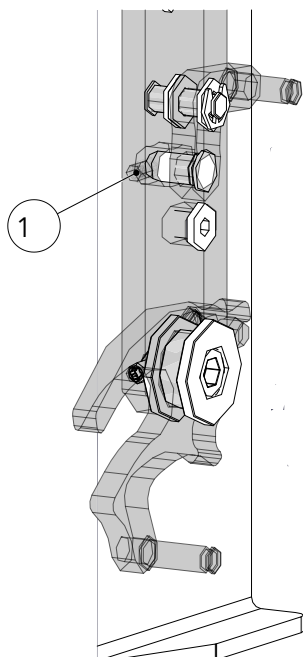
Fig. 56: Posizione B
