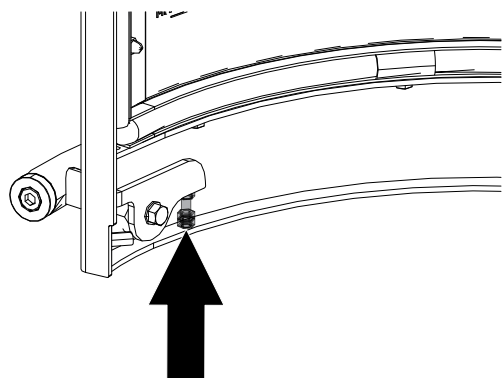
Fig. 37: Regolazione della maniglia dello sportello
