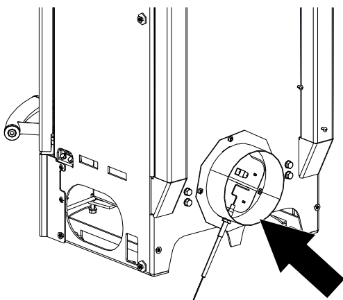
Fig. 16: Fissaggio del tubo Aluflex
