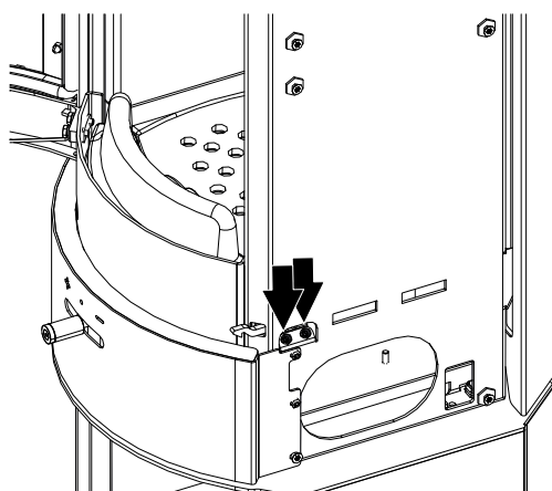
Fig. 36: Regolazione della serratura dello sportello
