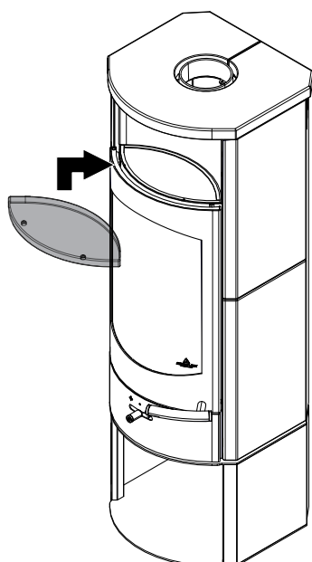
Fig. 31: Inserimento della piastra scaldavivande
