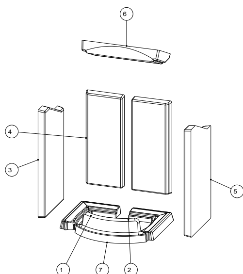
Fig. 32: Installazione del Keramott
