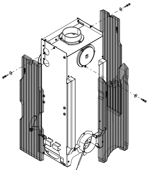
Fig. 48: Svitamento delle viti e smontaggio dell'HMS
