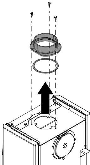
Fig. 18: Smontaggio della presa della canna fumaria
