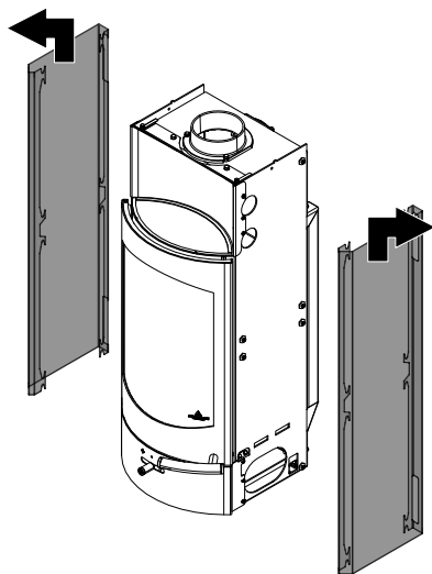
Fig. 47: Rimozione del rivestimento laterale
