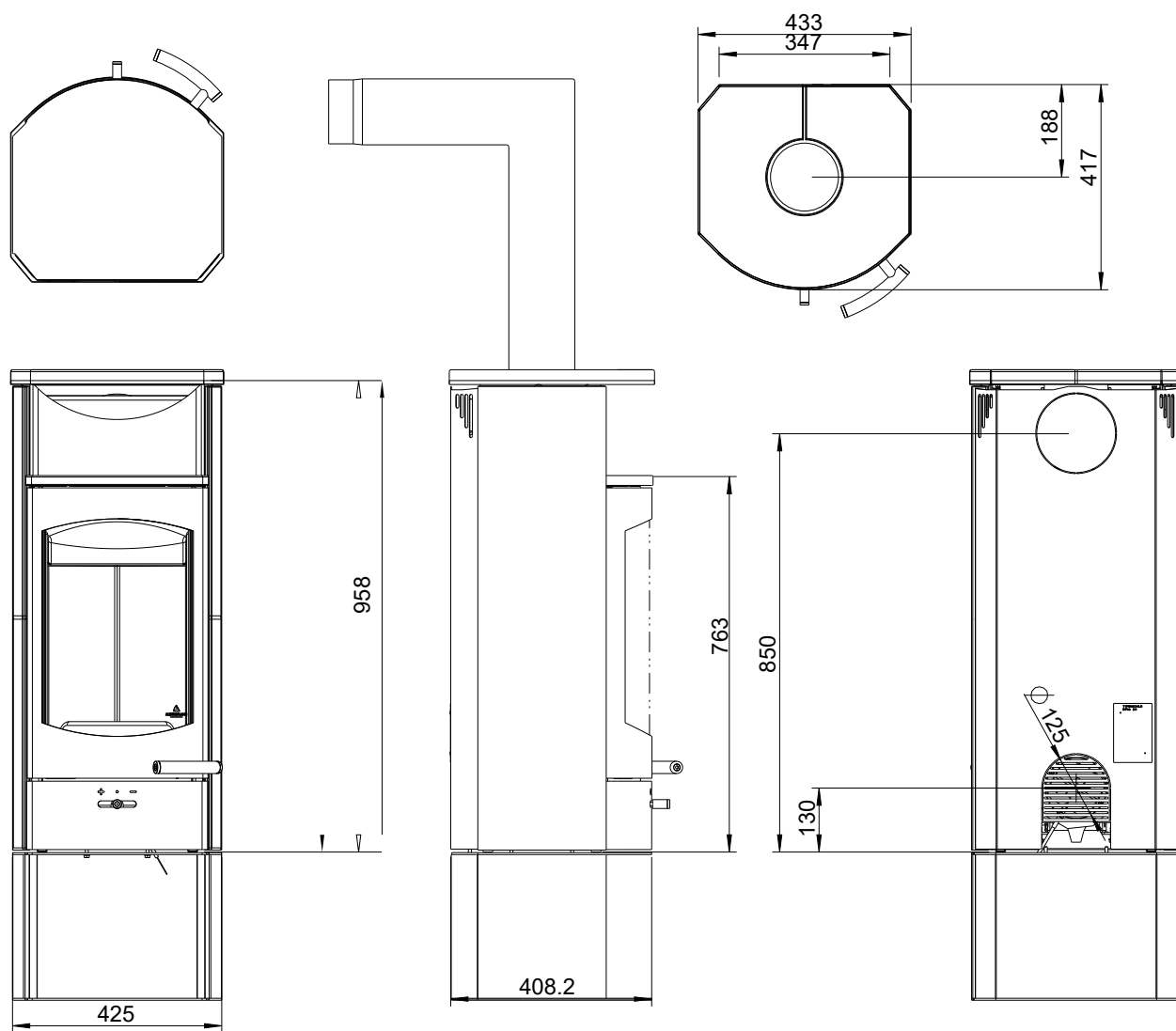
Fig. 2: Dimensioni con box portautensili
