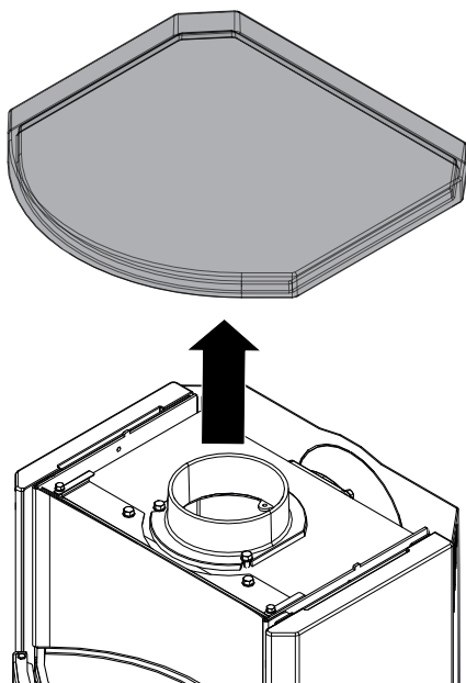
Fig. 45: Rimozione del coperchio
