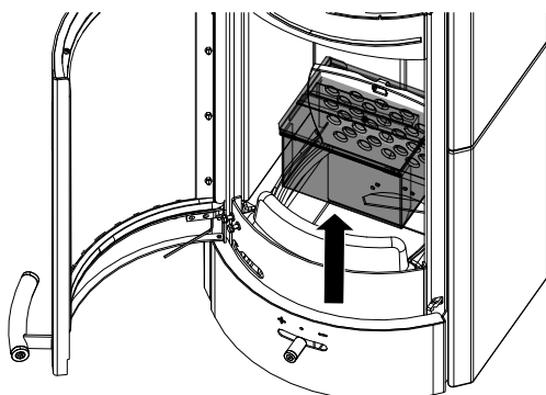
Fig. 44: Rimozione e svuotamento del box cenere
