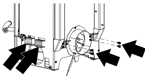
Fig. 26: Montaggio dei lamierini dell'HMS
