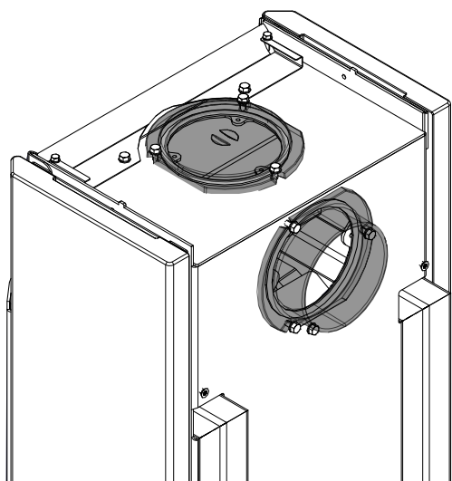
Fig. 13: Coperchio e pezzo di collegamento sostituiti
