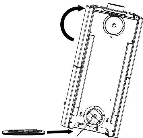
Fig. 21: Inclinamento della stufa
