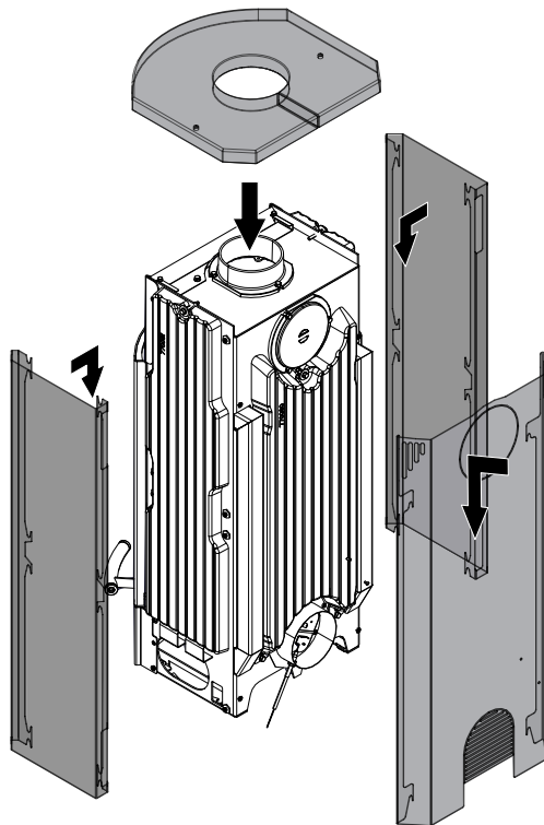
Fig. 28: Installazione del cappotto
