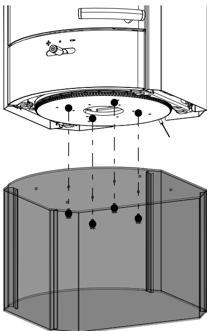
Fig. 24: Montaggio della base da dietro
