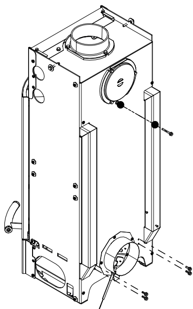
Fig. 25: Svitamento dei tappi d'arresto
