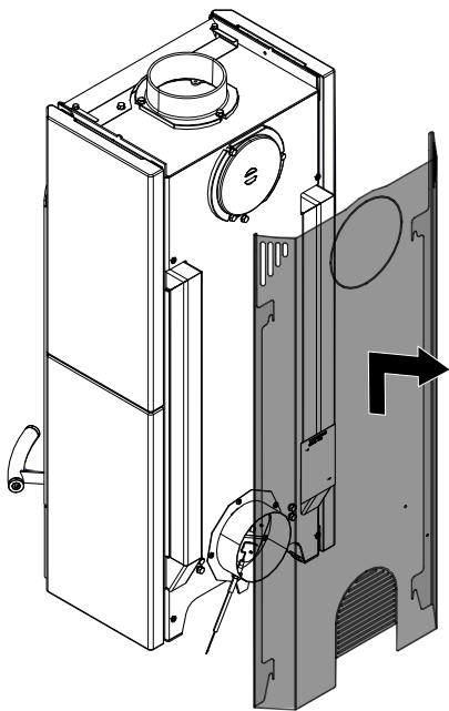
Fig. 46: Rimozione della parete posteriore
