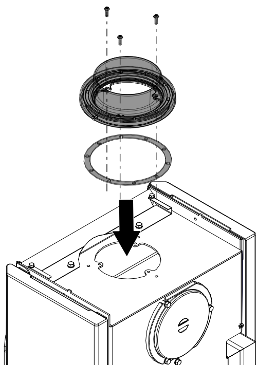
Fig. 19: Montaggio della presa della canna fumaria rotante
