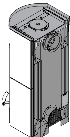
Fig. 14: Montaggio della parete posteriore e ricollocazione del coperchio
