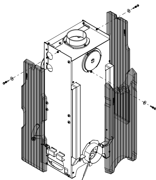
Fig. 27: Montaggio dell'HMI
