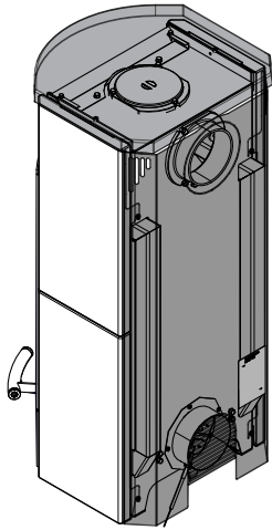
Fig. 17: Montaggio della parete posteriore e ricollocazione del coperchio
