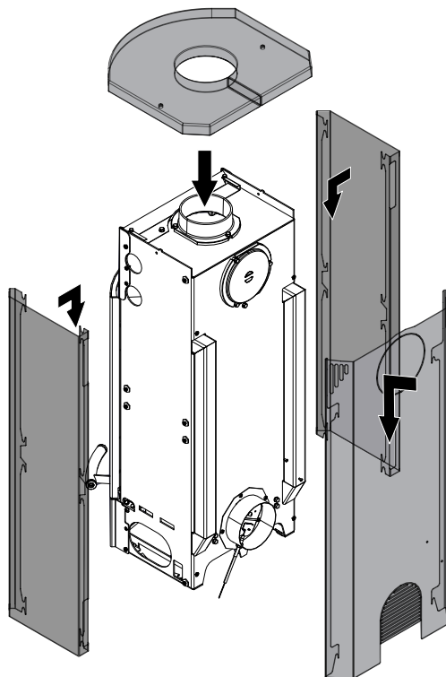
Fig. 29: Installazione dei cappotti
