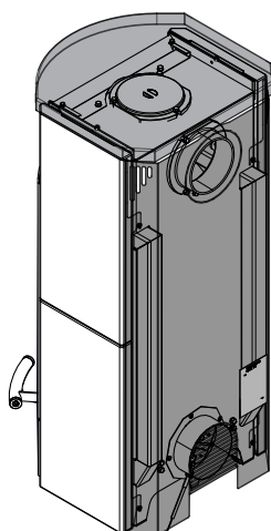
Fig. 20: Montaggio della parete posteriore e ricollocazione del coperchio
