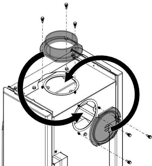
Fig. 12: Sostituzione del coperchio e del pezzo di collegamento
