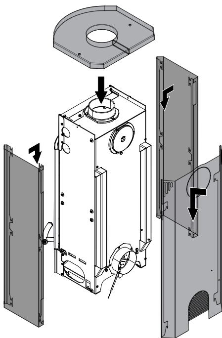
Fig. 49: Installazione dei cappotti
