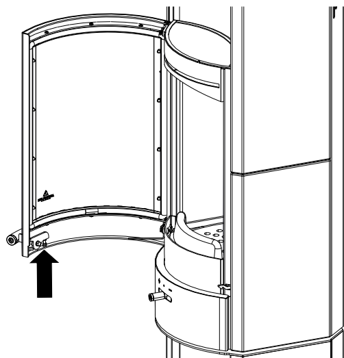
Fig. 37: Regolazione della maniglia dello sportello
