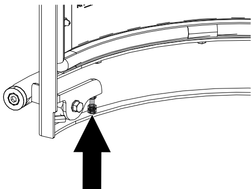
Abb. 38: Türgriff einstellen
