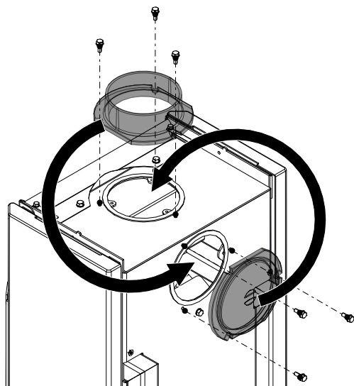
Abb. 13: Abdeckung und Stützen tauschen
