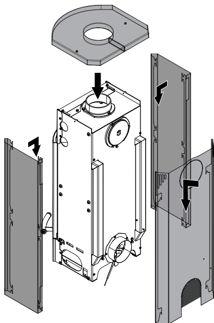
Abb. 30: Verkleidungen anbringen
