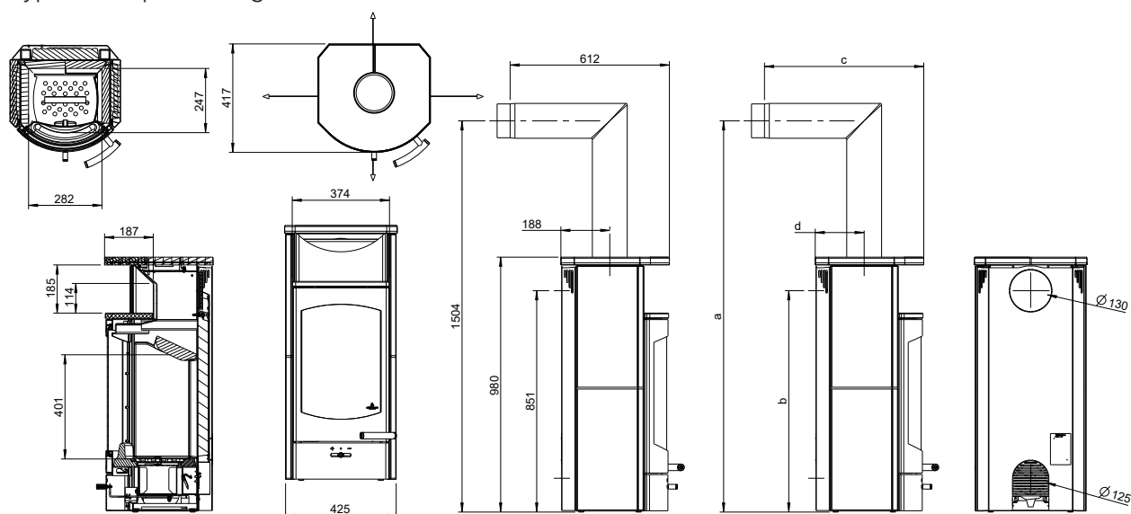
Abb. 2: Abmessungen Grundgerät
