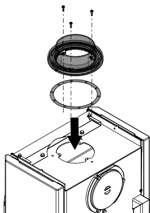
Abb. 20: Drehrauchrohrstutzen montieren
