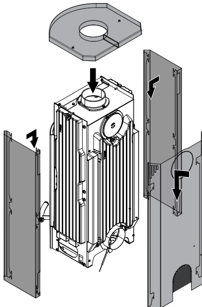
Abb. 29: Verkleidung anbringen
