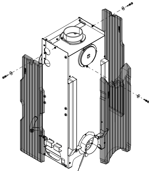
Abb. 28: HMI montieren
