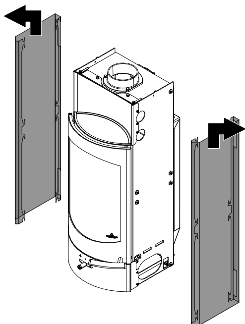
Abb. 48: Seitenverkleidung abnehmen
