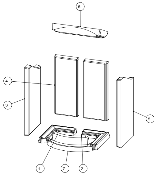
Abb. 33: Keramott einbauen
