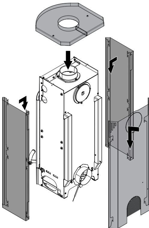
Abb. 50: Verkleidungen anbringen
