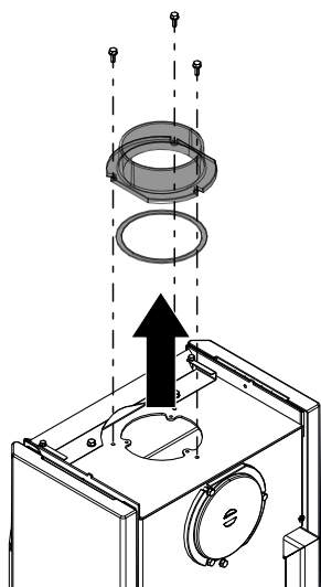
Abb. 19: Rauchrohrstutzen abmontieren
