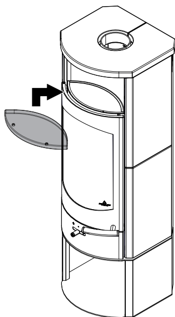
Abb. 32: Warmhalteplatte einlegen
