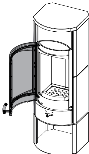
Abb. 36: Tür öffnen
