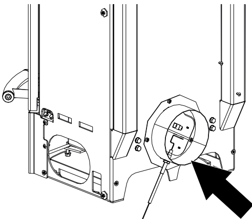
Abb. 17: Aluflexschlauch befestigen
