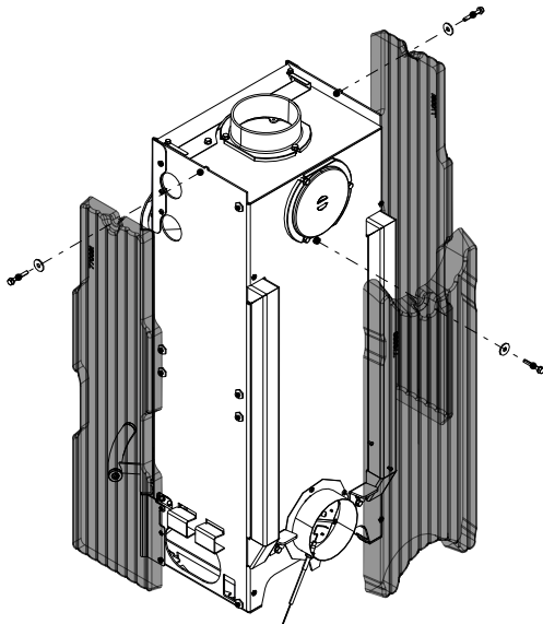
Abb. 49: Schrauben lösen und HMS demontieren
