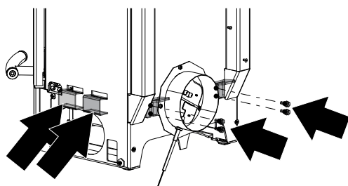
Abb. 27: HMS-Bleche montieren
