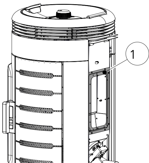
Fig. 17: Installer le couvercle d'installation du PGI
