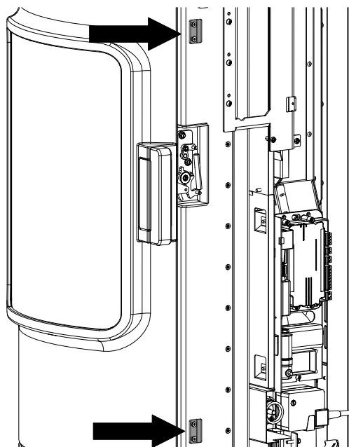
Fig. 9: Plaques d'appui
