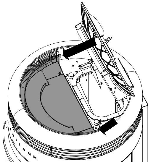
Fig. 42: Ouvrir le couvercle du réservoir
