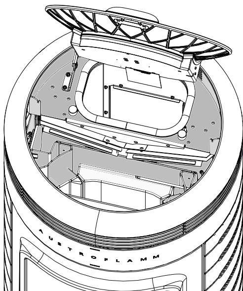
Fig. 47: Nettoyer les vides
