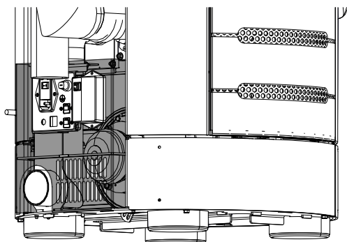
Fig. 19: Accrocher la paroi arrière basse du PGI.
