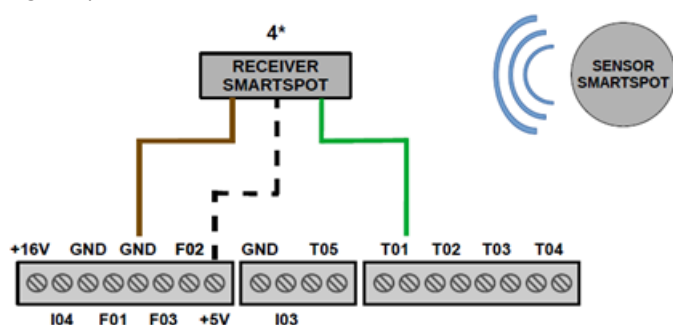
Fig. 32: Récepteur Smart Spot
