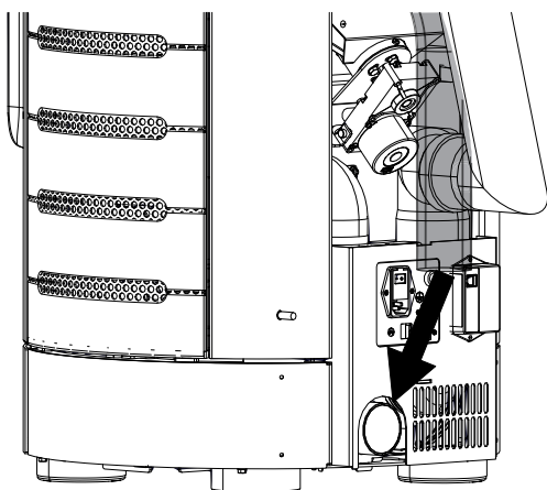
Fig. 20: Raccorder le flexible à l'arrivée d'air entrant
