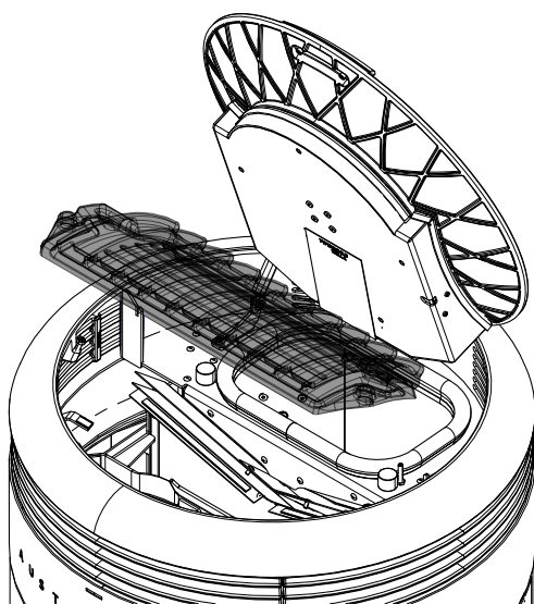
Fig. 45: Extraire le couvercle en fonte de la chambre de combustion
