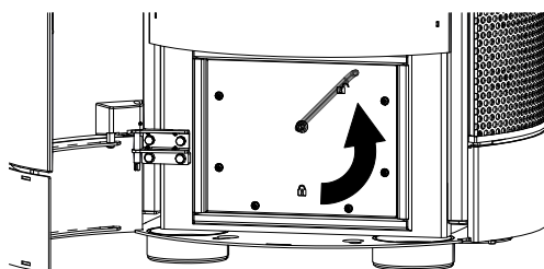
Fig. 49: Extraire le bac à cendres
