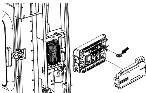
Fig. 40: Remplacer la pile mémoire
