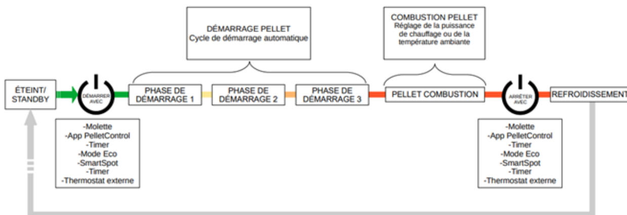
Fig. 31: Diagramme des fonctions
