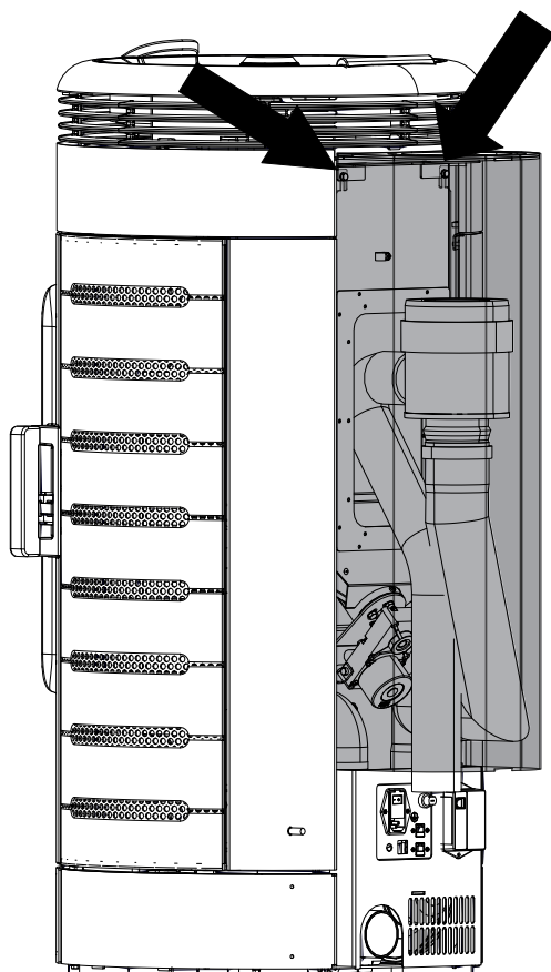
Fig. 21: Accrocher la paroi arrière du PGI
