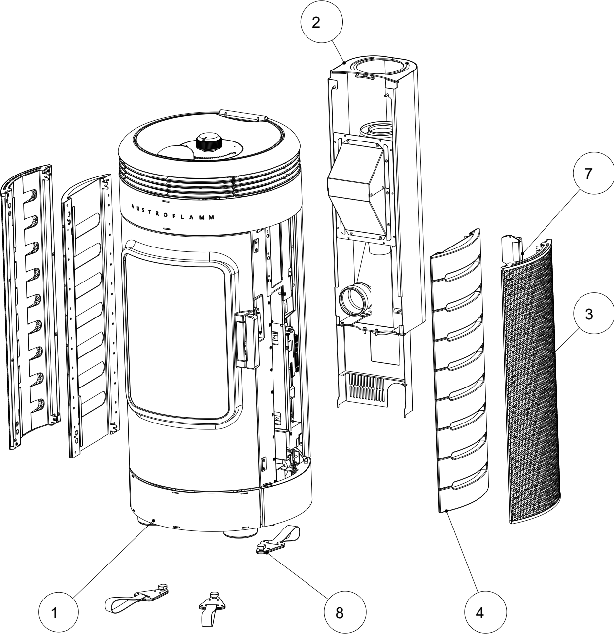
Fig. 57: Accessoires du Ella
