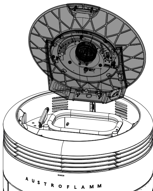
Fig. 42: Ouvrir le couvercle du réservoir
