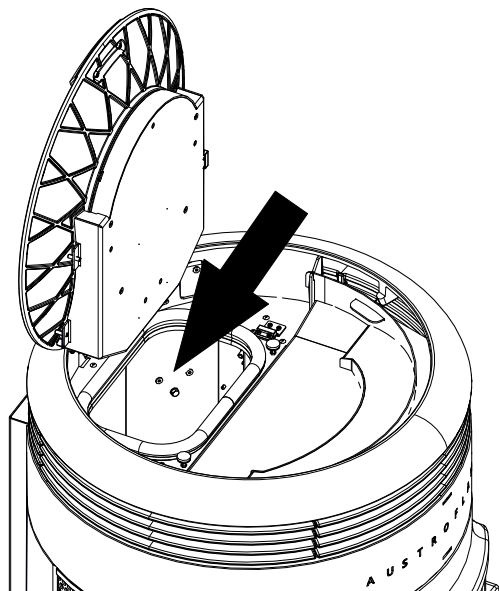
Fig. 23: Remplir les pellets
