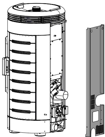
Fig. 15: Enlever l'habillage arrière
