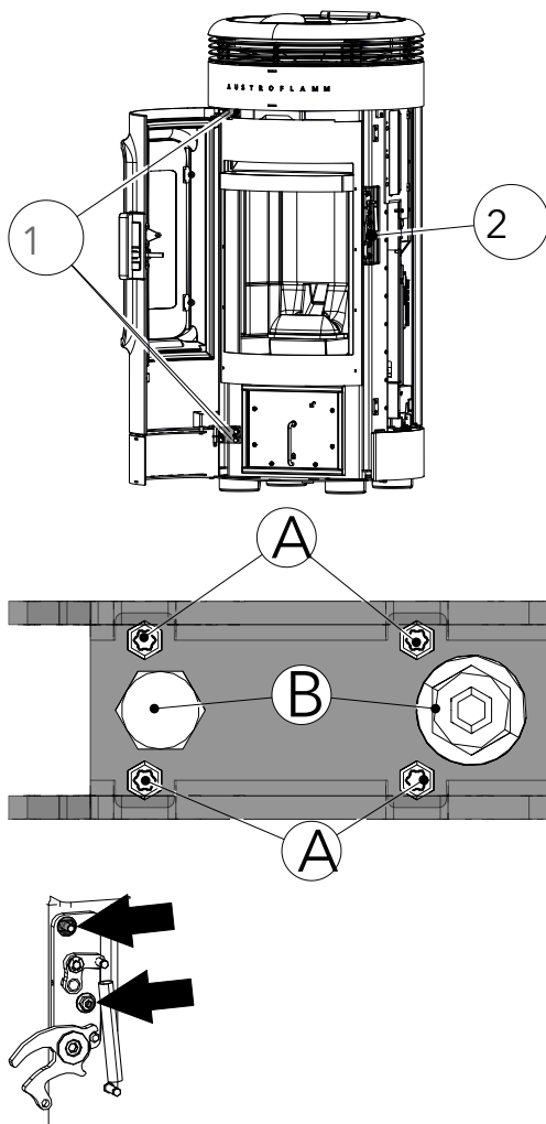
Fig. 37: Ajuster la porte du foyer
