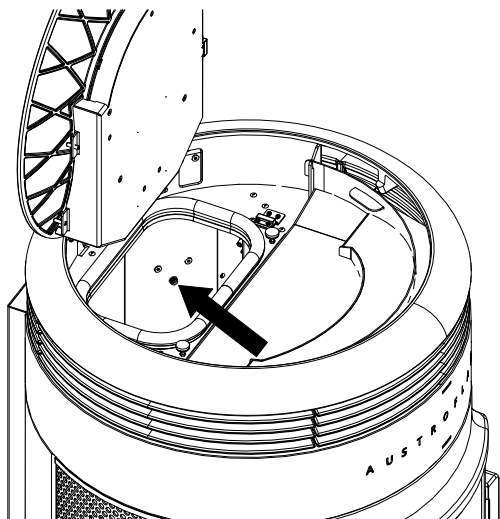
Fig. 39: Dévisser la vis
