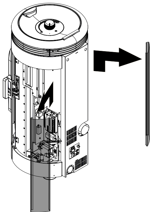
Fig. 56: Enlever l'habillage latéral
