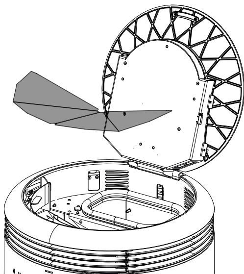
Fig. 44: Extraire la plaque de protection contre le rayonnement
