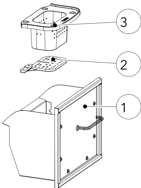
Fig. 41: Nettoyer la grille basculante
