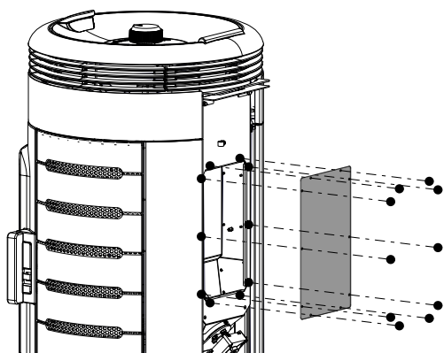
Fig. 16: Déposer le capot
