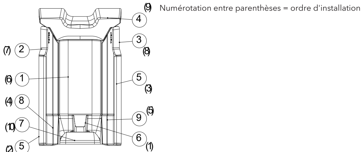
Fig. 14: Installer la Keramott
