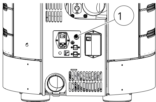
Fig. 52: Limiteur de température de sécurité
