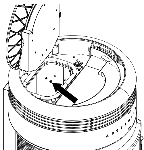
Fig. 55: Dévisser la vis
