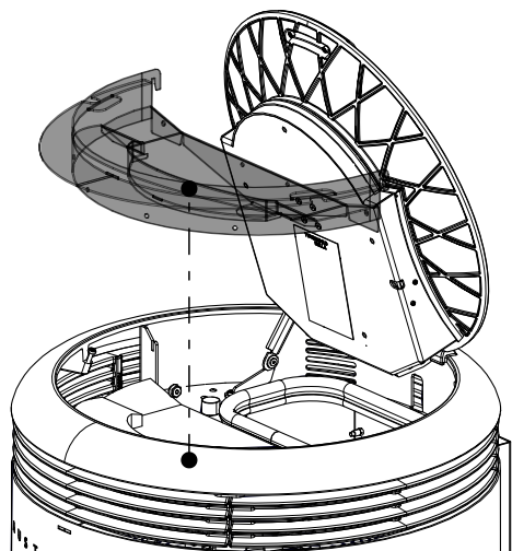
Fig. 43: Extraire le caisson isolant
