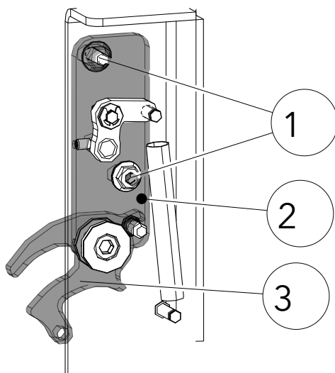
Fig. 38: Régler la force de fermeture de la porte
