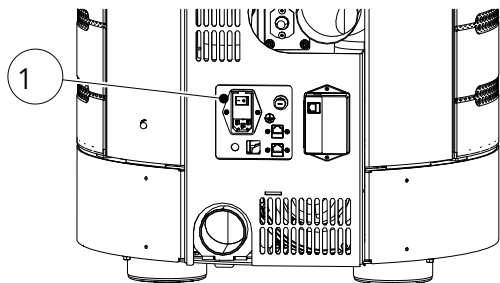
Fig. 53: Cartouche fusible avec fusibles à tube de verre T2,5 A
