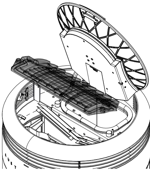
Abb. 45: Guss-Feuerraumdeckel herausnehmen
