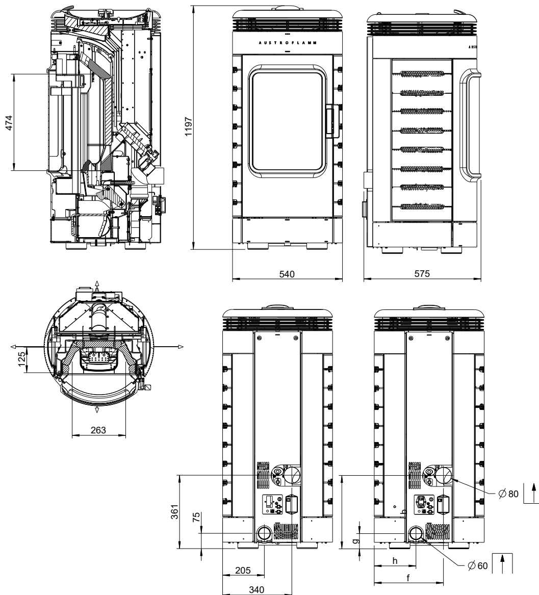
Abb. 2: Ella Abmessungen
