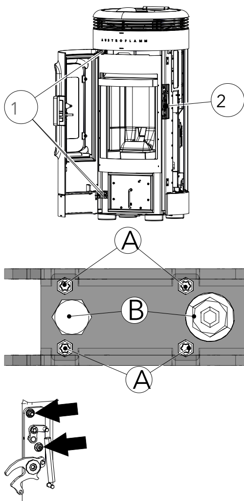
Abb. 37: Feuerraumtür einstellen
