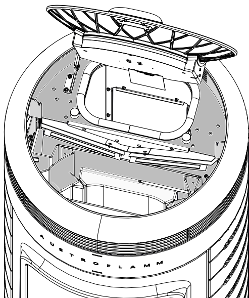
Abb. 47: Hohlraum reinigen
