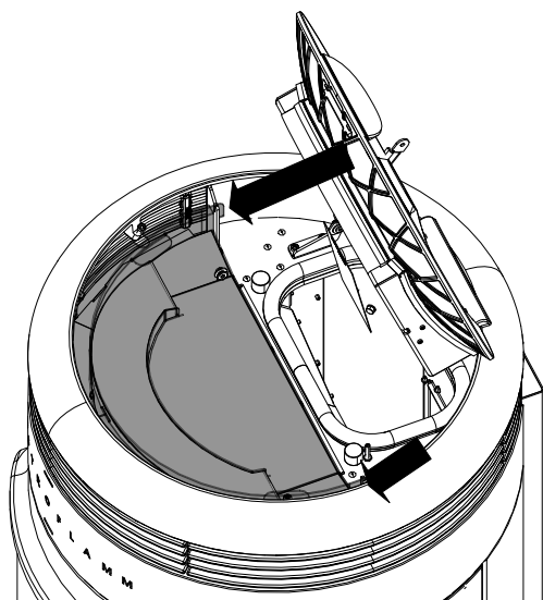
Abb. 42: Tankdeckel öffnen
