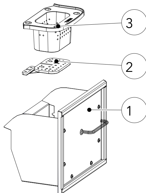
Abb. 41: Kipprost reinigen
