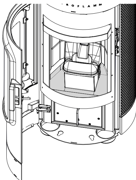
Abb. 48: Feuerraum reinigen
