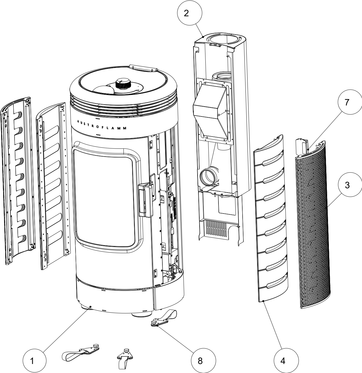
Abb. 57: Ella Zubehör
