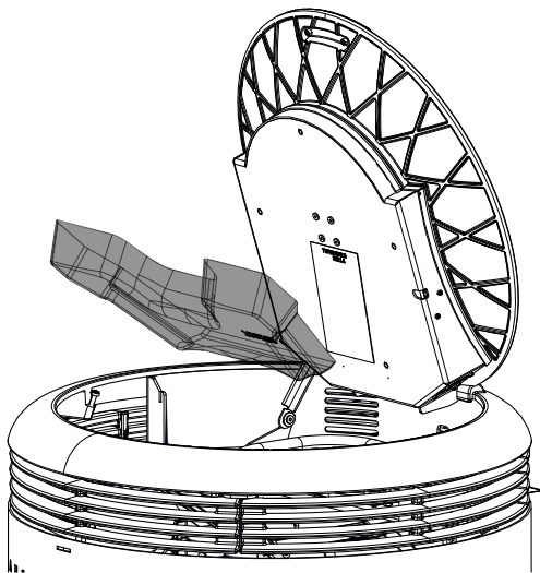
Abb. 46: Keramik herausnehmen
