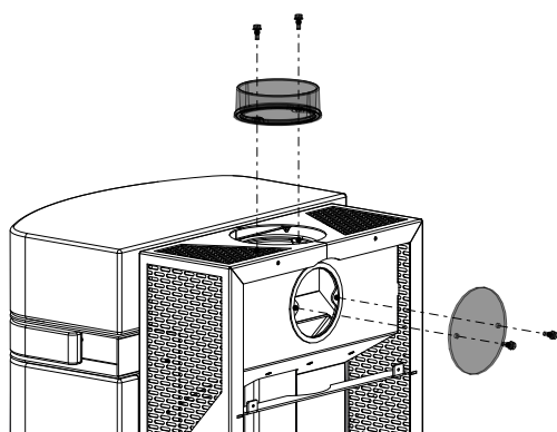
Abb. 11: Abdeckung und Rauchrohrstutzen demontieren
