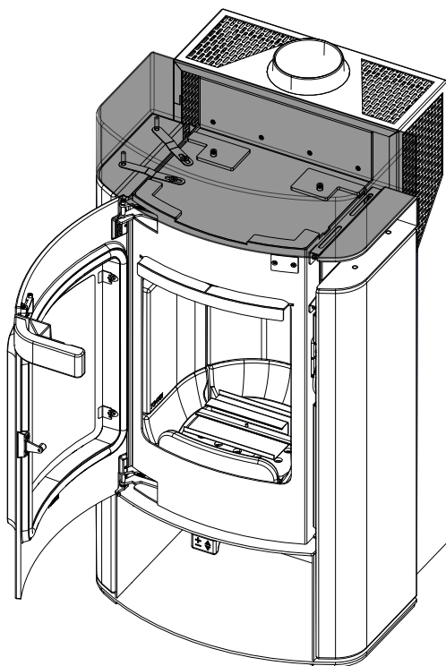
Abb. 46: Deckel abnehmen
