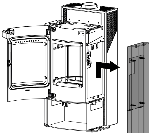
Abb. 50: Verkleidung rechts abnehmen
