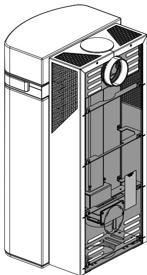
Abb. 14: Rückwand montieren
