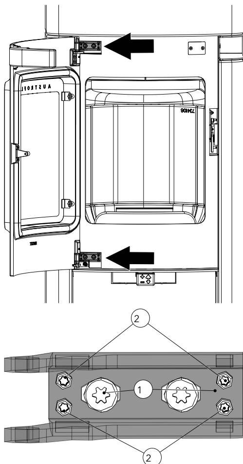
Abb. 36: Türeinstellschrauben
