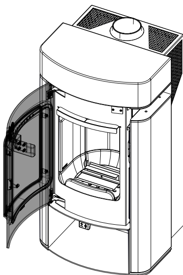
Abb. 45: Tür öffnen
