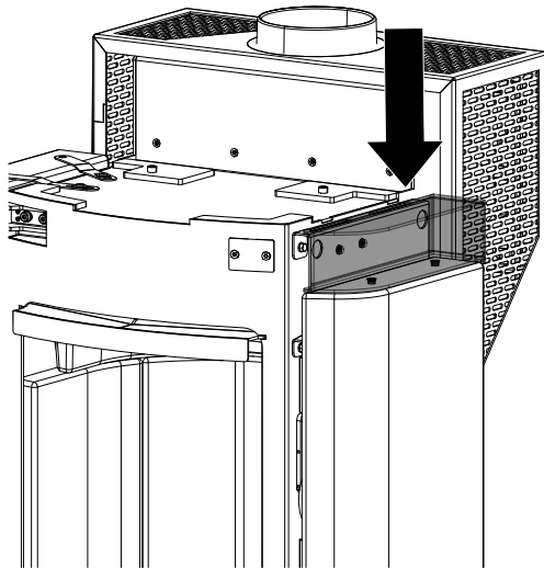
Abb. 27: Griffbox einsetzen
