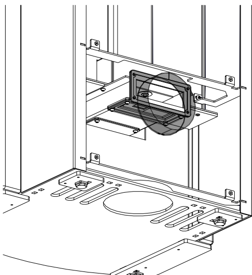
Abb. 20: Luftanschluss hinten
