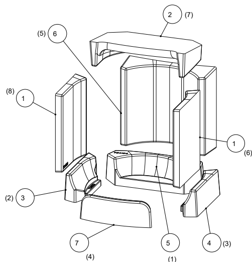
Abb. 31: Keramott
