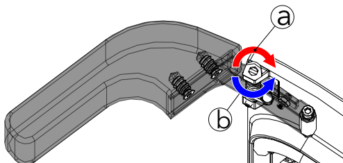
Abb. 35: Griff schließt leicht / stark
