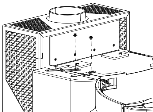
Abb. 25: Schrauben Halter verschrauben
