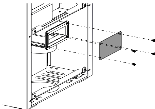
Abb. 17: hinteren Deckel demontieren
