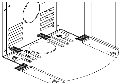
Abb. 7: Transportsicherung entfernen (Ansicht von unten)
