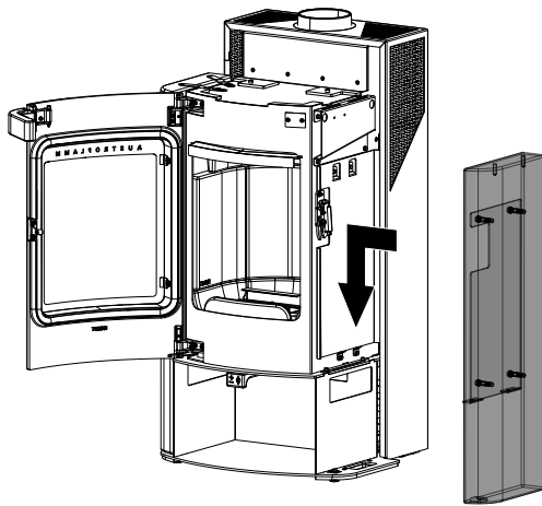
Abb. 26: Rechte Verkleidung einhängen
