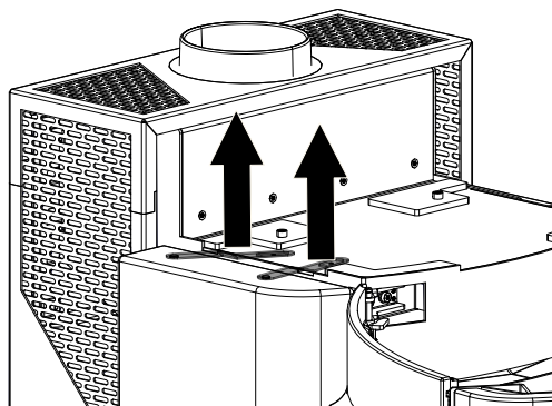
Abb. 52: Halter entfernen
