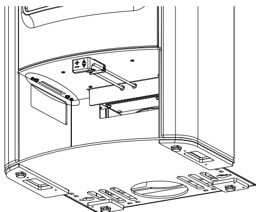
Abb. 37: Einstellschrauben Seitenverkleidung
