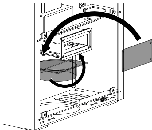
Abb. 19: Zuluftflansch und Deckel tauschen
