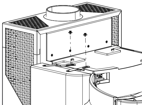
Abb. 51: Halter lösen
