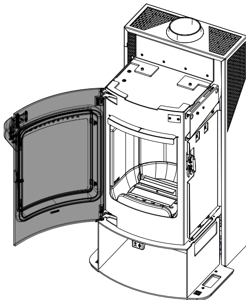
Abb. 21: Tür öffnen
