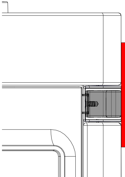
Abb. 33: Griff bündig mit Seitenverkleidung
