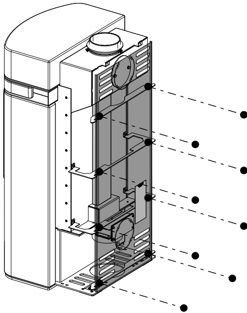
Abb. 15: Rückwand abnehmen
