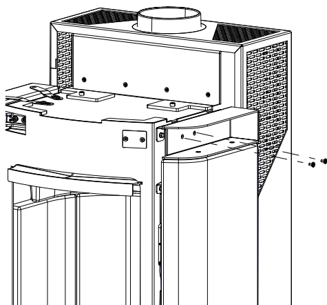
Abb. 48: Schrauben entfernen
