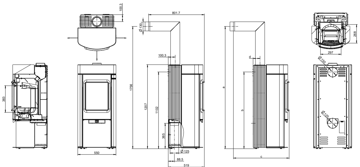
Abb. 3: Abmessungen Elisabeth
