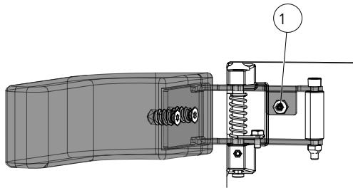
Abb. 32: Griff einstellen
