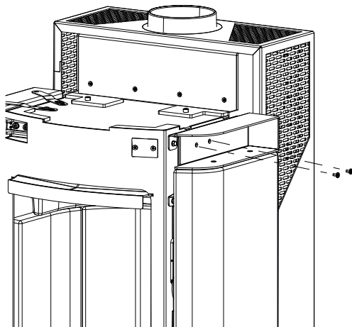
Abb. 28: Rechte Verkleidung sichern
