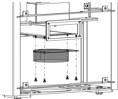
Abb. 18: Zuluftflansch unten demontieren
