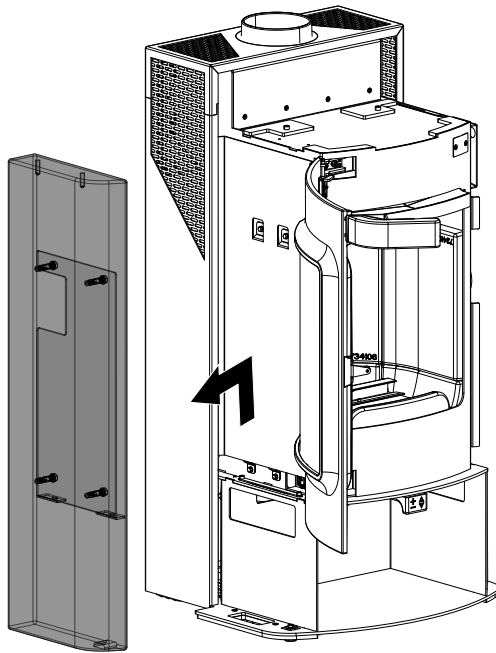
Abb. 53: Verkleidung links abnehmen
