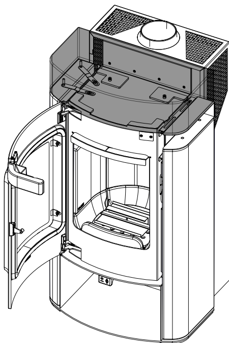
Abb. 29: Deckel anbringen
