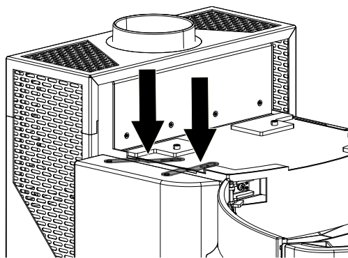
Abb. 24: Halter anbringen
