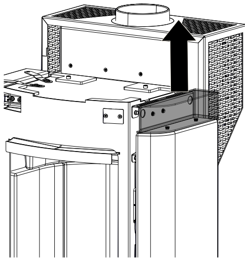
Abb. 49: Griffbox anheben
