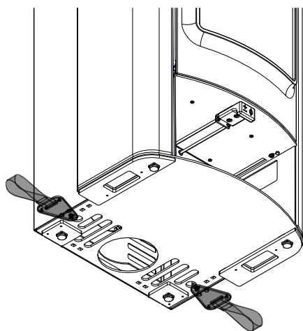
Abb. 8: Transporthilfe
