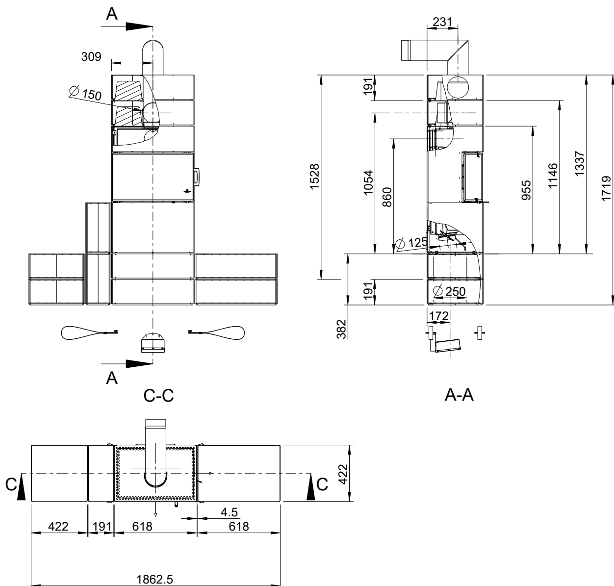
Fig. 1: Dimensions
