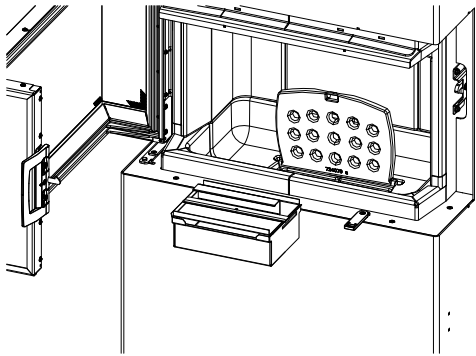
Fig. 36: Enlever et vider le bac à cendres
