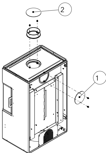
Fig. 8: Démonter le recouvrement et la tubulure
