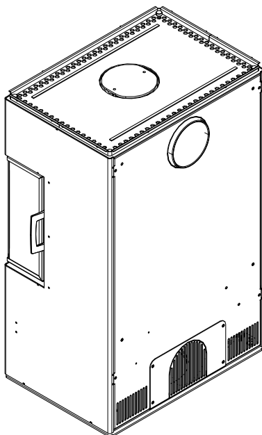
Fig. 10: Installer la paroi arrière
