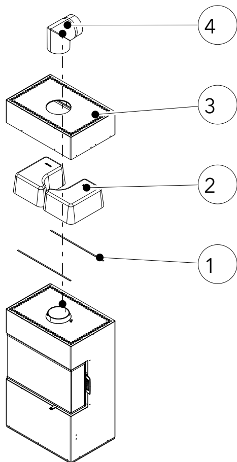
Fig. 15: Installer l'HMS
