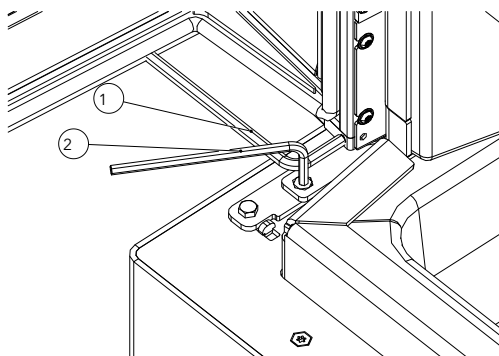
Fig. 27: Libérer le ressort et sécuriser
