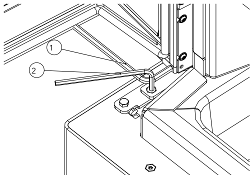
Fig. 37: Bloquer le ressort et dévisser la vis
