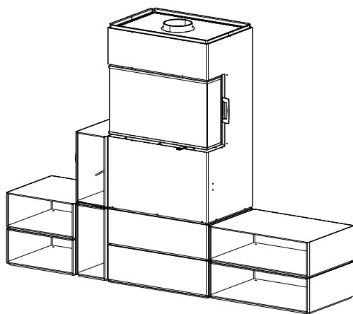
Fig. 17: Ajout des modules latéraux
