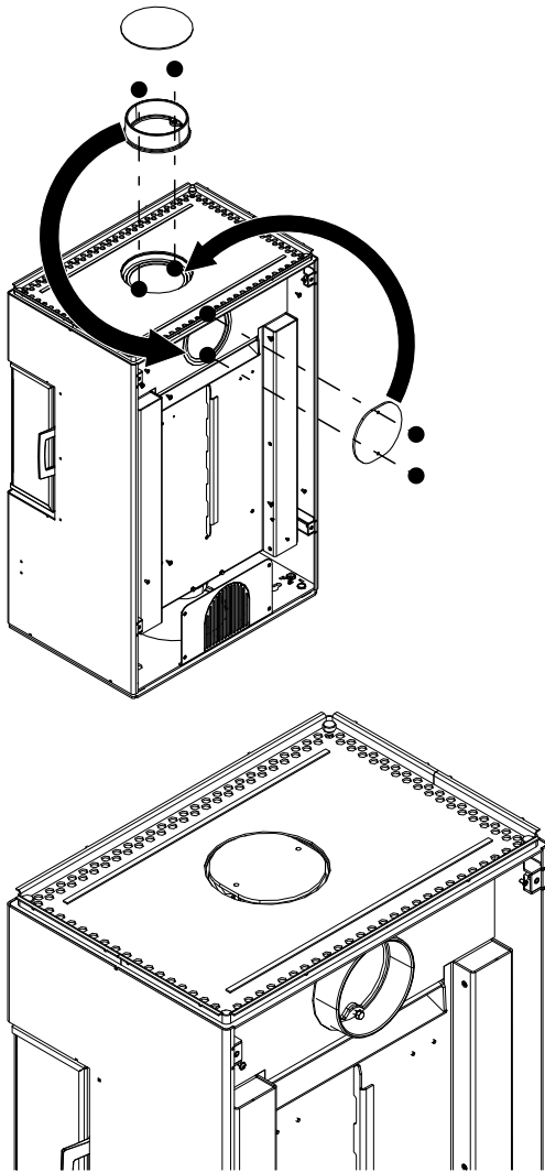
Fig. 9: Interchanger le recouvrement et la tubulure
