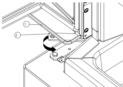
Fig. 26: Tendre le ressort
