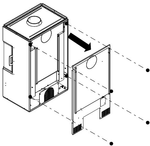
Fig. 6: Installer la paroi arrière
