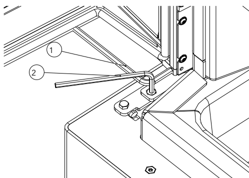
Fig. 24: Bloquer le ressort et dévisser la vis
