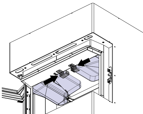
Fig. 32: Extraire les pierres HMS
