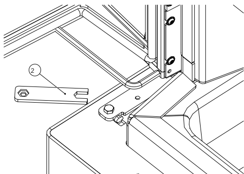
Fig. 38: Extraire le dispositif de serrage de la porte
