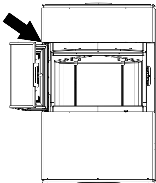
Fig. 39: Décrocher et déposer la porte
