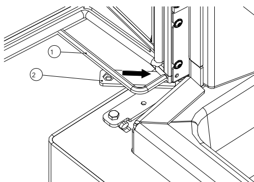
Fig. 25: Libérer le ressort
