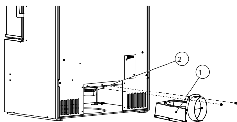
Fig. 12: Installer l'adaptateur d'arrivée d'air
