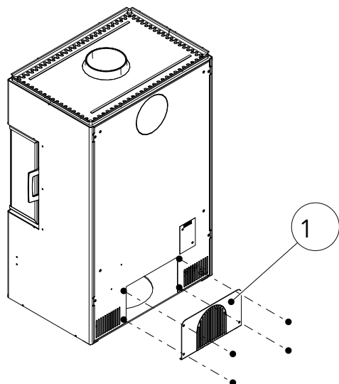
Fig. 11: Démontez le couvercle de révision de la paroi arrière
