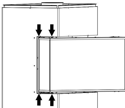
Fig. 23: Régler la porte avec les vis
