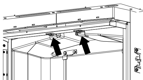
Fig. 14: Installer la Keramott
