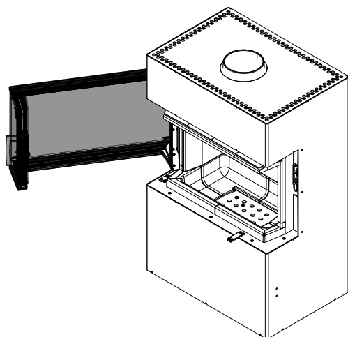
Abb. 19: Tür öffnen
