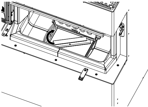
Abb. 35: Deckel auf Aschebox geben
