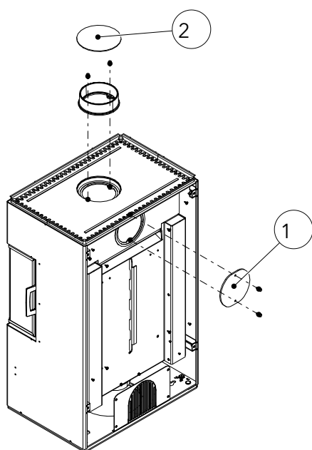
Abb. 9: Abdeckung und Stützen demontieren
