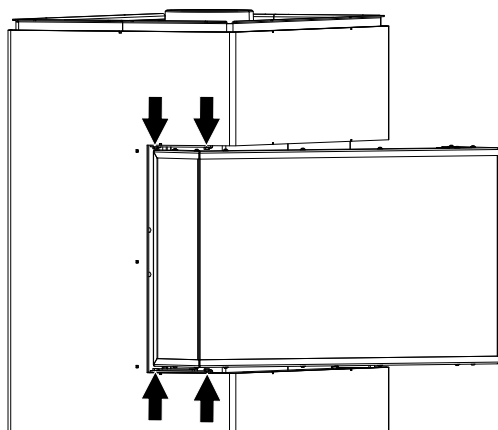
Abb. 24: Tür mit Schrauben einstellen
