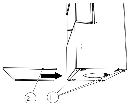
Abb. 17: Schattenfuge montieren
