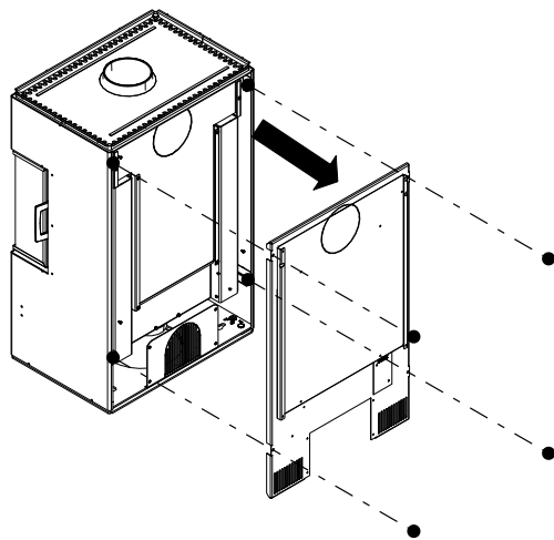
Abb. 7: Rückwand abmontieren
