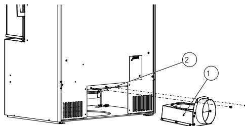
Abb. 13: Zuluftadapter montieren
