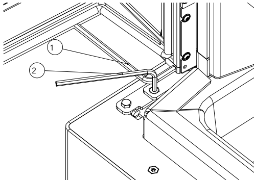
Abb. 25: Feder sichern und Schraube lösen
