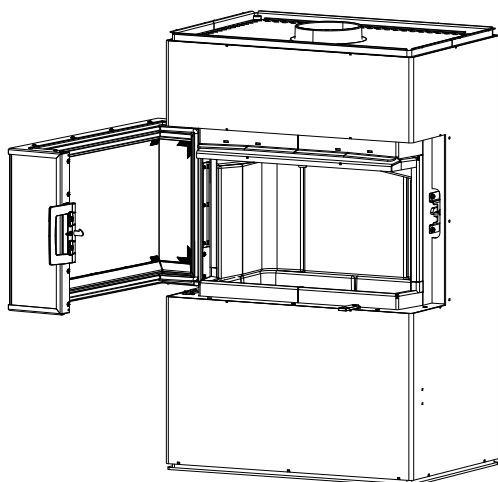
Abb. 23: Tür öffnen
