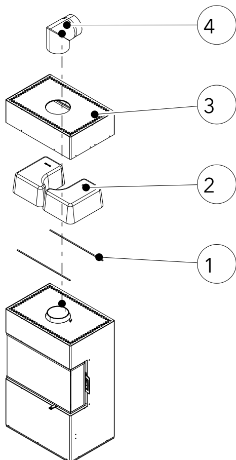
Abb. 16: HMS montieren
