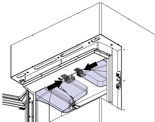
Abb. 33: HMS-Steine herausnehmen
