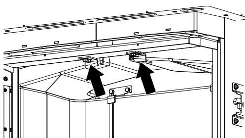
Abb. 15: Keramott einbauen
