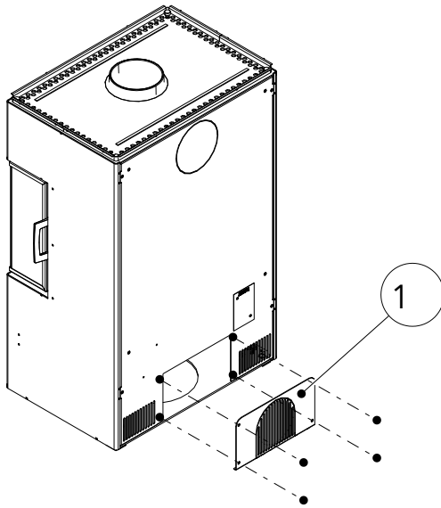
Abb. 12: Rückwandrevision demontieren
