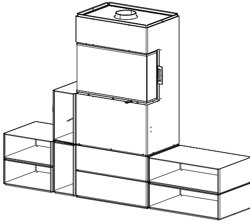
Abb. 18: Beistellboxen dazustellen
