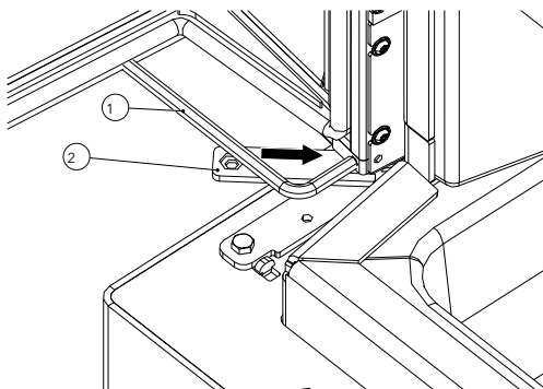
Abb. 26: Feder lösen
