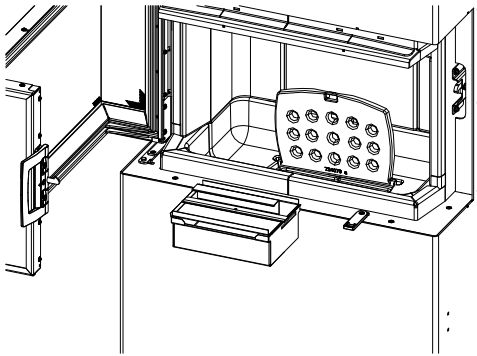
Abb. 37: Aschebox rausnehmen und entleeren
