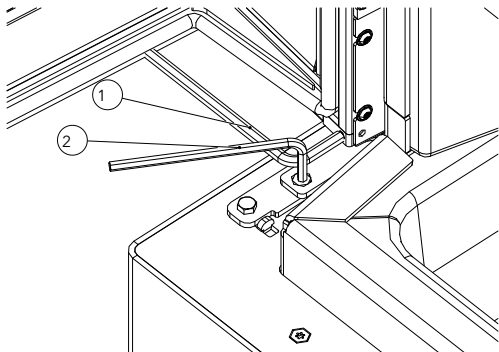
Abb. 38: Feder sichern und Schraube lösen
