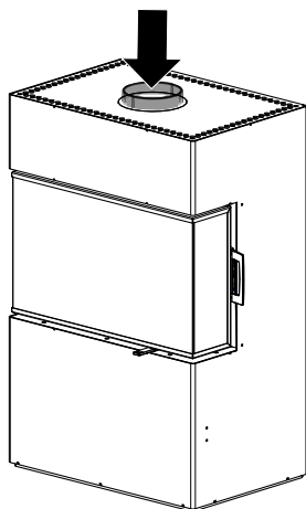
Abb. 32: Rauchgaswege von oben reinigen
