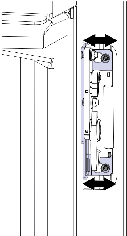
Abb. 21: Verschluss einstellen
