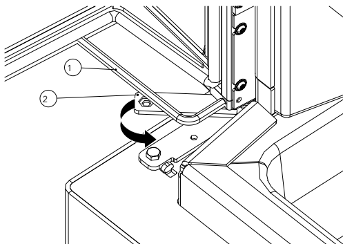
Abb. 27: Feder spannen
