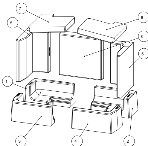
Abb. 14: Keramott
