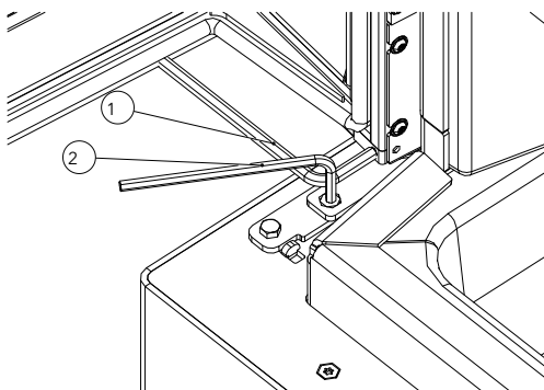
Abb. 28: Feder lösen und sichern
