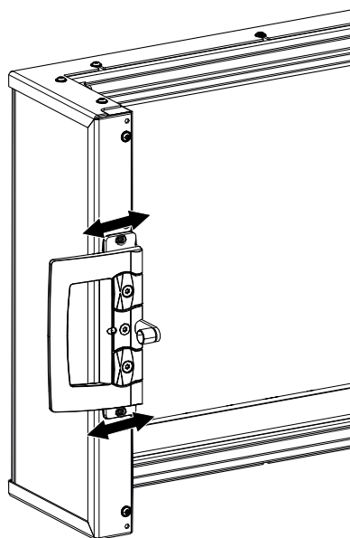
Abb. 20: Griff einstellen
