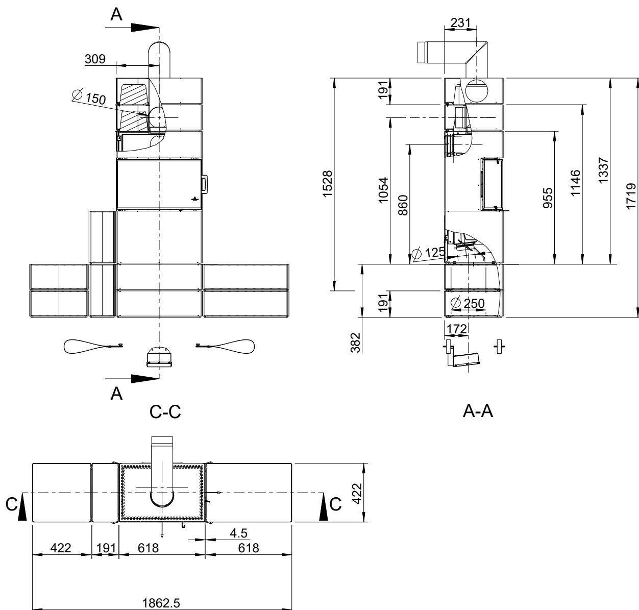
Abb. 2: Abmessungen
