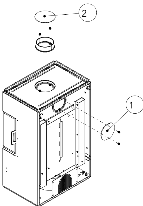
Fig. 13: Démonter le recouvrement et la tubulure
