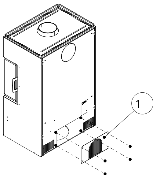
Fig. 16: Démontez le couvercle de révision de la paroi arrière
