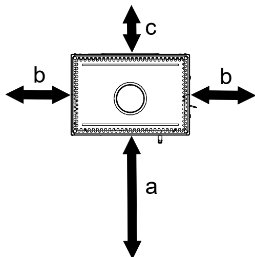
Fig. 9: Distances de sécurité (vue de dessus) - installation au mur
