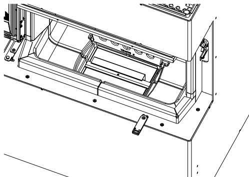
Fig. 39: Fermer le couvercle
