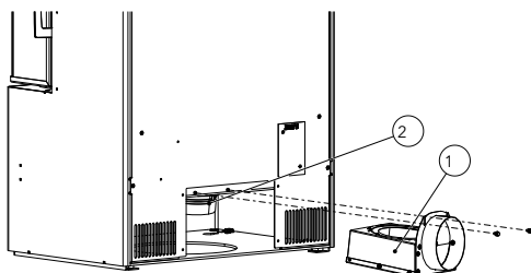
Fig. 17: Installer l'adaptateur d'arrivée d'air
