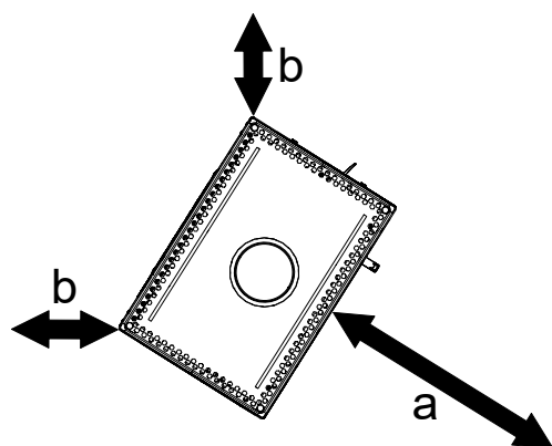
Fig. 10: Distances de sécurité (vue de dessus) - installation en angle
