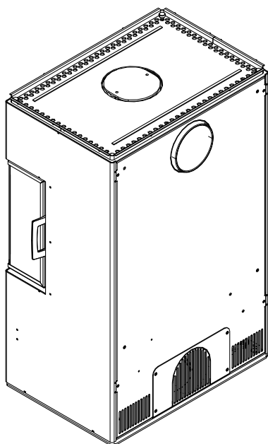
Fig. 15: Installer la paroi arrière
