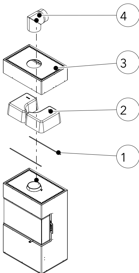
Fig. 20: Montaggio dell'HMS
