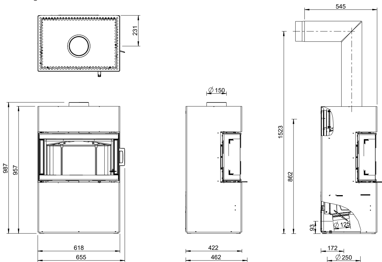
Fig. 1: Dimensioni
