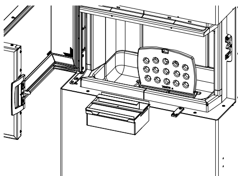
Fig. 40: Rimozione e svuotamento del box cenere
