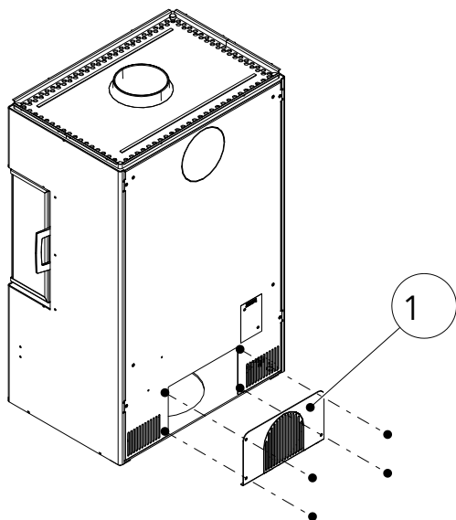
Fig. 16: Smontaggio della modifica della parete posteriore
