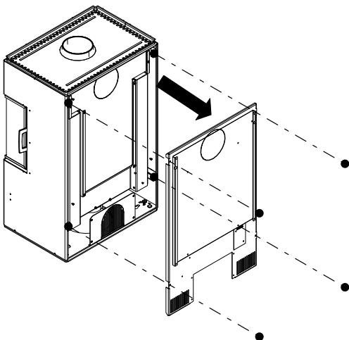
Fig. 10: Smontaggio della parete posteriore
