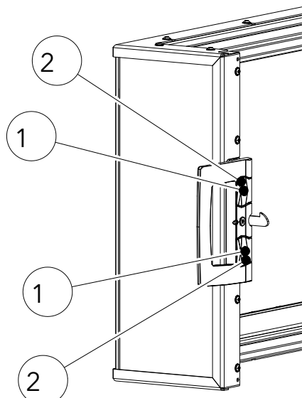
Fig. 23: Regolazione della maniglia
