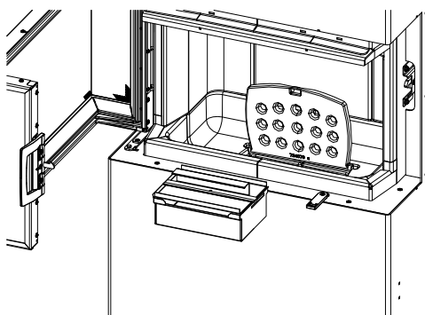
Fig. 40: Rimozione e svuotamento del box cenere
