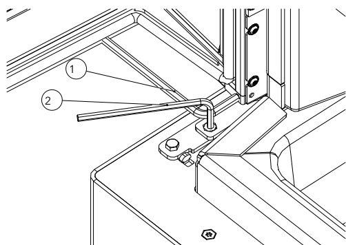
Fig. 32: Allentamento e fissaggio della molla
