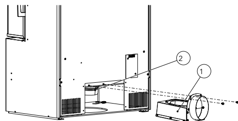
Fig. 16: Montaggio dell'adattatore dell'aria di alimentazione
