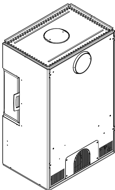
Fig. 14: Rimontaggio della parete posteriore
