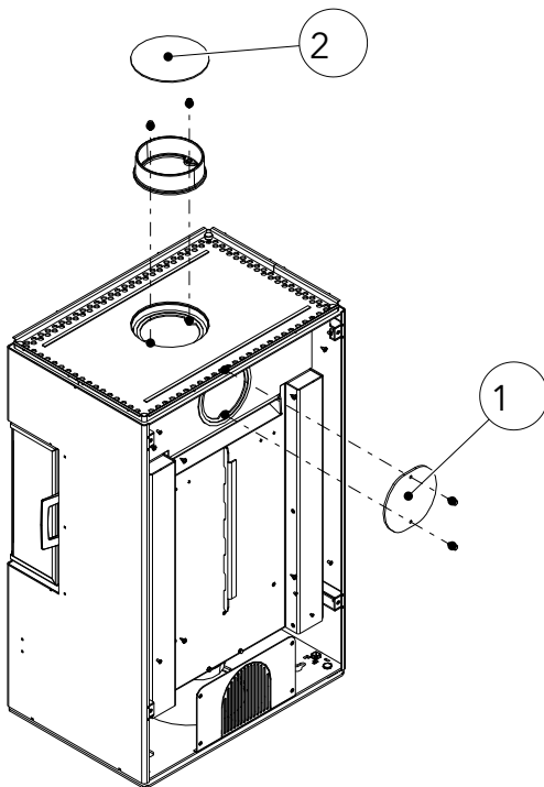
Fig. 12: Smontaggio del coperchio e del pezzo di collegamento
