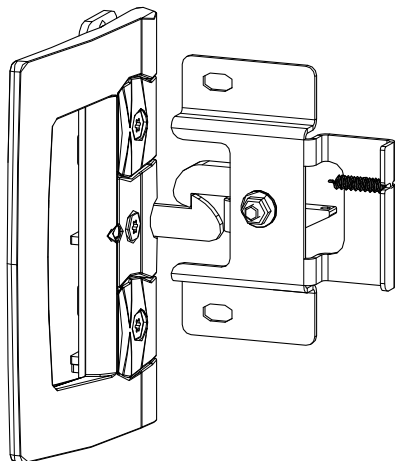
Fig. 26: Innesto della maniglia
