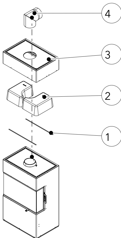
Fig. 19: Montaggio dell'HMS
