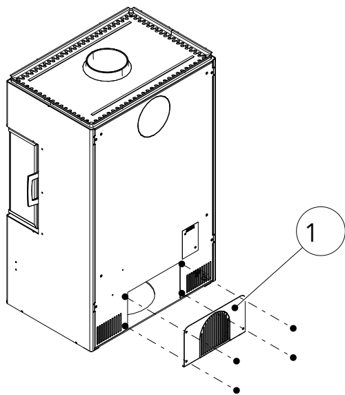
Fig. 15: Smontaggio della modifica della parete posteriore
