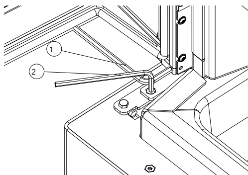
Fig. 29: Fissaggio della molla e allentamento della vite
