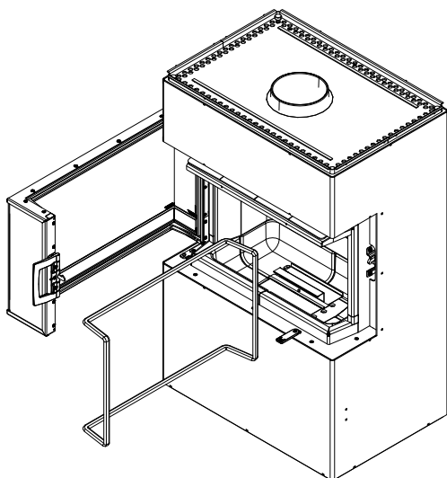
Fig. 36: Sostituzione della guarnizione
