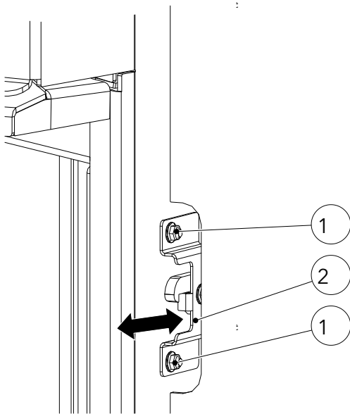
Fig. 25: Regolazione della chiusura
