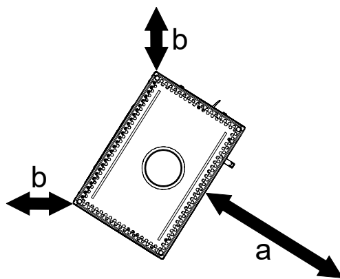
Fig. 9: Distanze di sicurezza (vista dall'alto) - Installazione ad angolo
