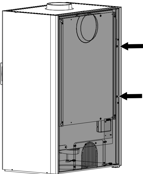
Fig. 39: Smontaggio della parete posteriore
