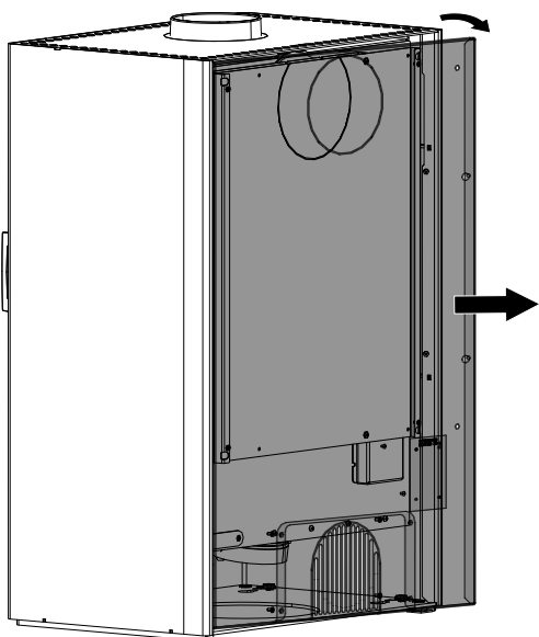
Fig. 40: Sganciamento della parete posteriore
