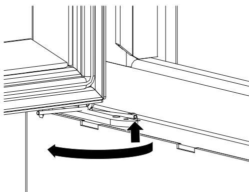
Fig. 43: Allentamento della molla
