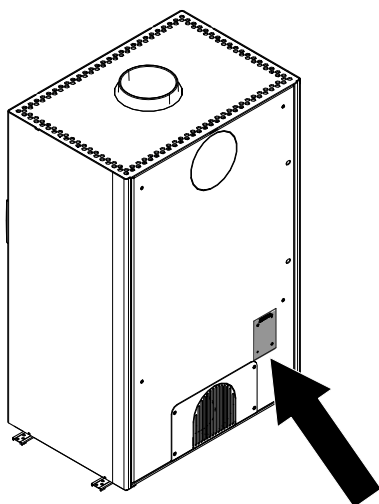
Fig. 5: Plaque signalétique
