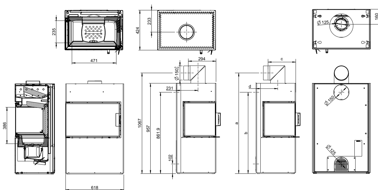
Fig. 1: Dimensions Dexter 2.0 gauche
