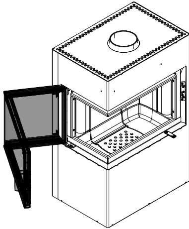
Fig. 22: Ouvrir la porte
