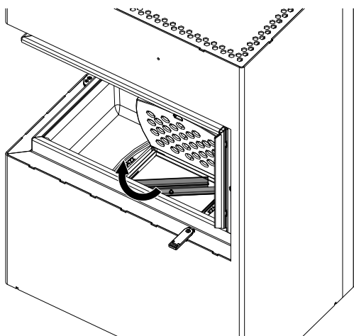
Fig. 30: Mettre le couvercle sur le bac à cendres
