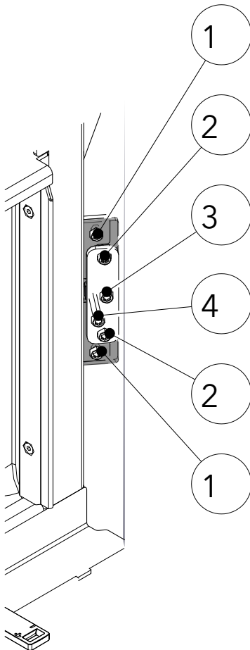
Fig. 23: Régler la serrure de la porte
