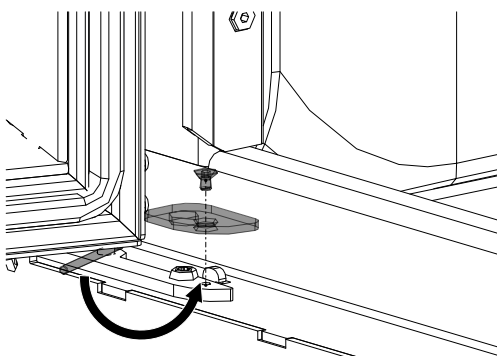
Fig. 21: Accrocher la porte et tendre le ressort
