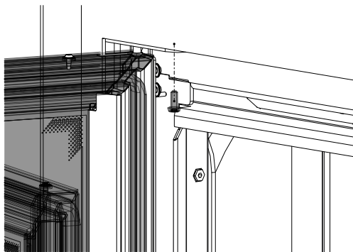
Fig. 20: Accrocher la porte
