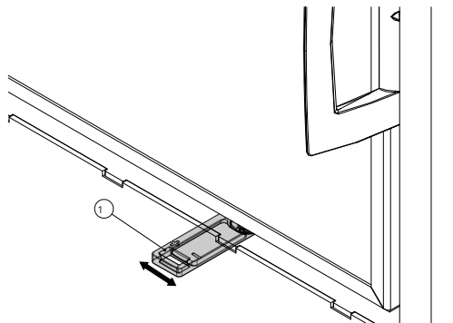
Fig. 26: Manette de régulation de l'air primaire / secondaire
