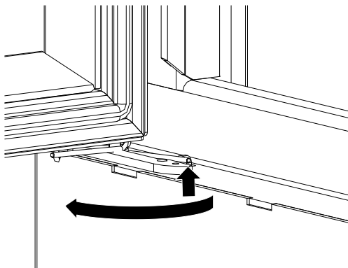
Fig. 37: Libérer le ressort
