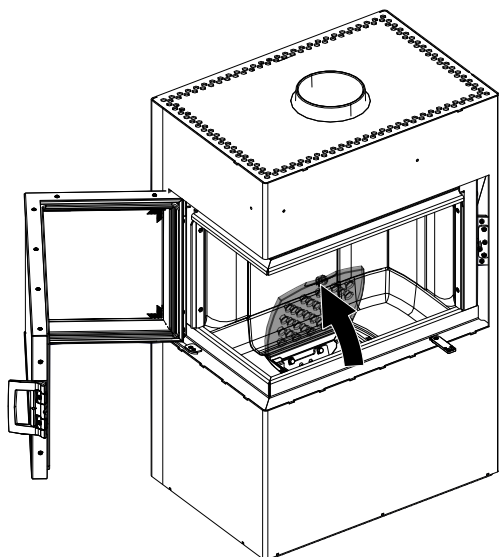
Fig. 29: Relever la grille
