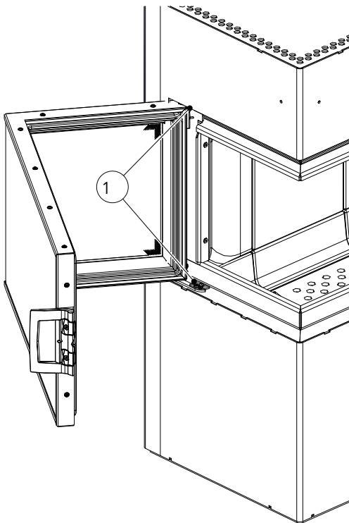
Fig. 24: Ouvrir la porte
