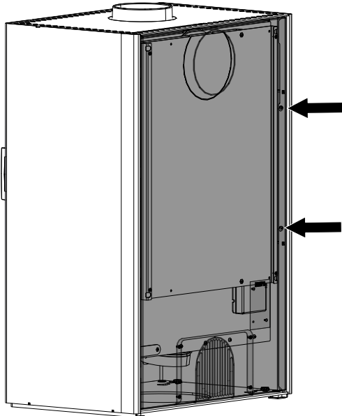
Fig. 37: Smontaggio della parete posteriore
