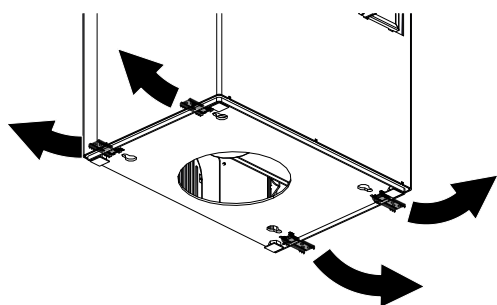
Fig. 6: Rimozione dei fermi di trasporto
