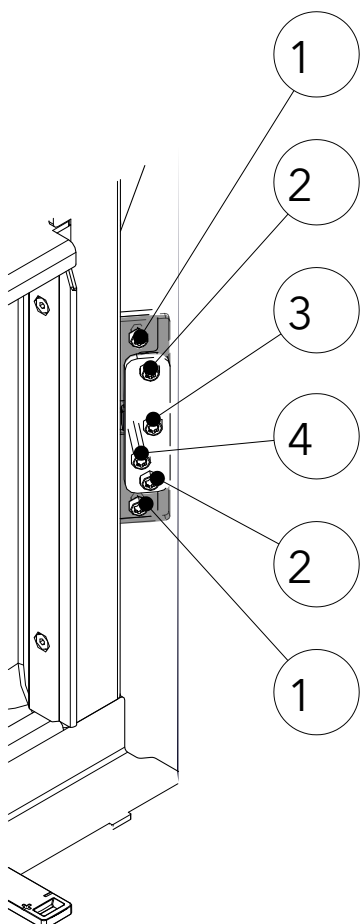
Fig. 28: Regolazione della serratura dello sportello
