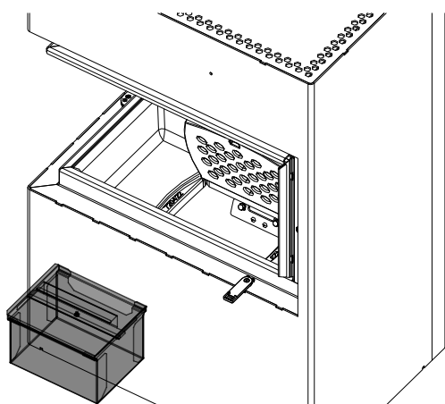
Fig. 38: Rimozione e svuotamento del box cenere
