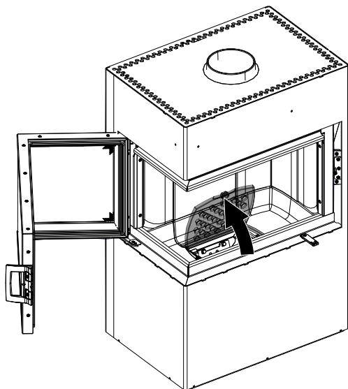
Fig. 35: Sollevamento della griglia
