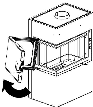
Fig. 44: Rimozione dello sportello
