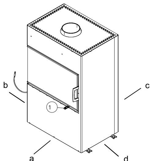
Fig. 8: Distanze di sicurezza
