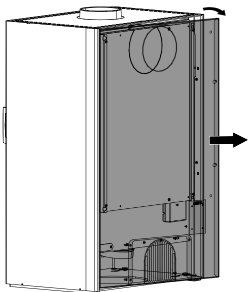
Fig. 40: Sganciamento della parete posteriore
