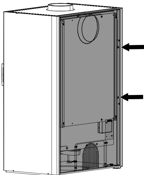
Fig. 39: Smontaggio della parete posteriore
