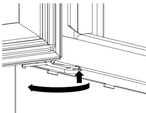
Fig. 43: Allentamento della molla
