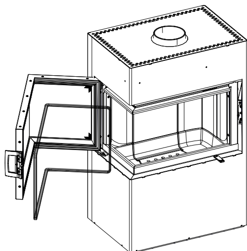
Fig. 34: Sostituzione della guarnizione
