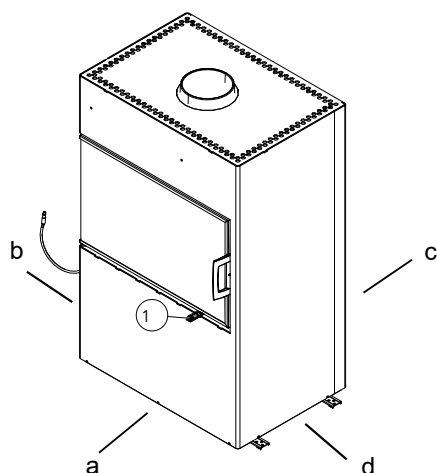
Fig. 3: Distanze di sicurezza (a,b,c) / regolatore dell'aria
